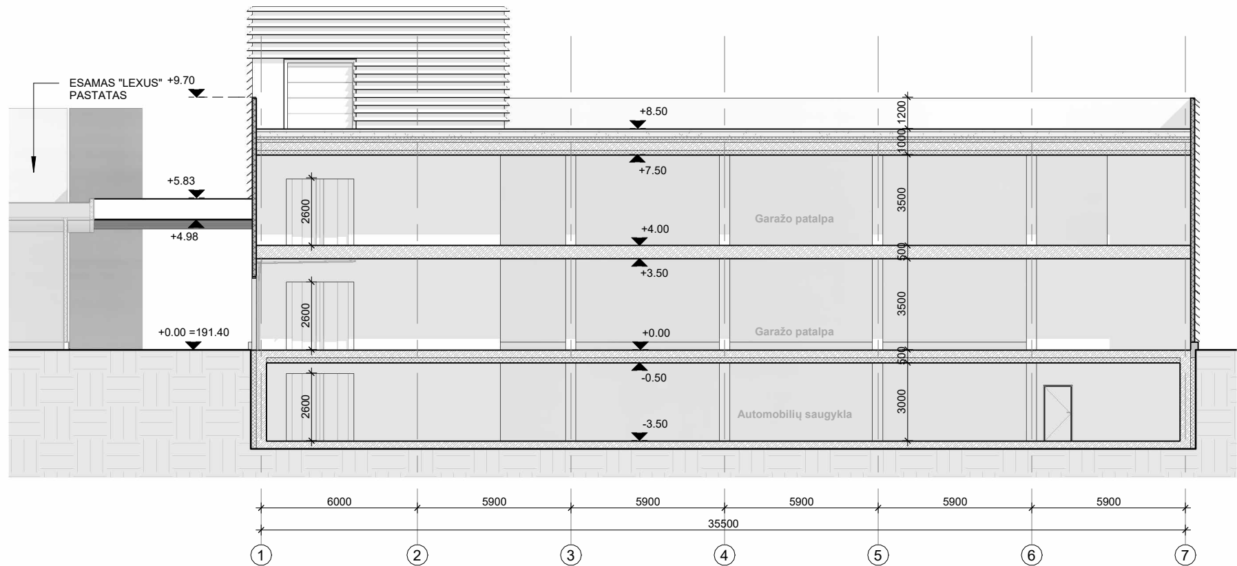
AUTOMOBILIŲ GARAŽAS. PJŪVIS 2 1 : 200
