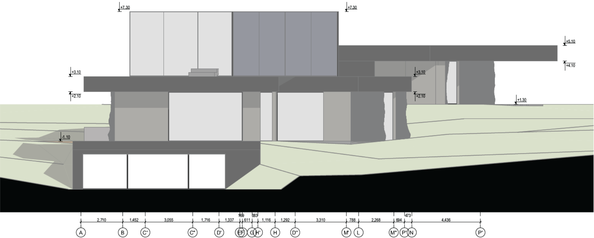
FASADAS A-P1
