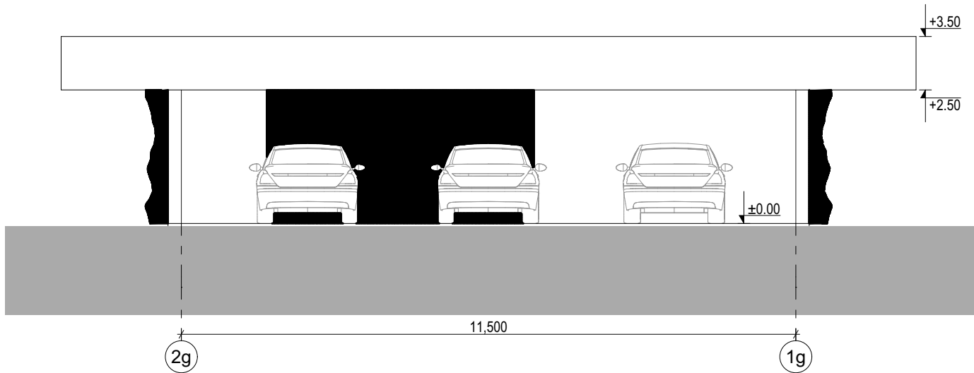
FASADAS 2g1g M 1:100
