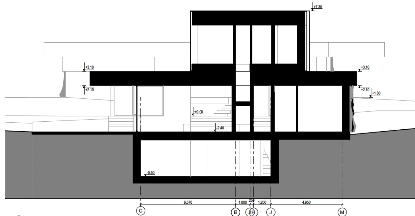
PJŪVIS A-A
