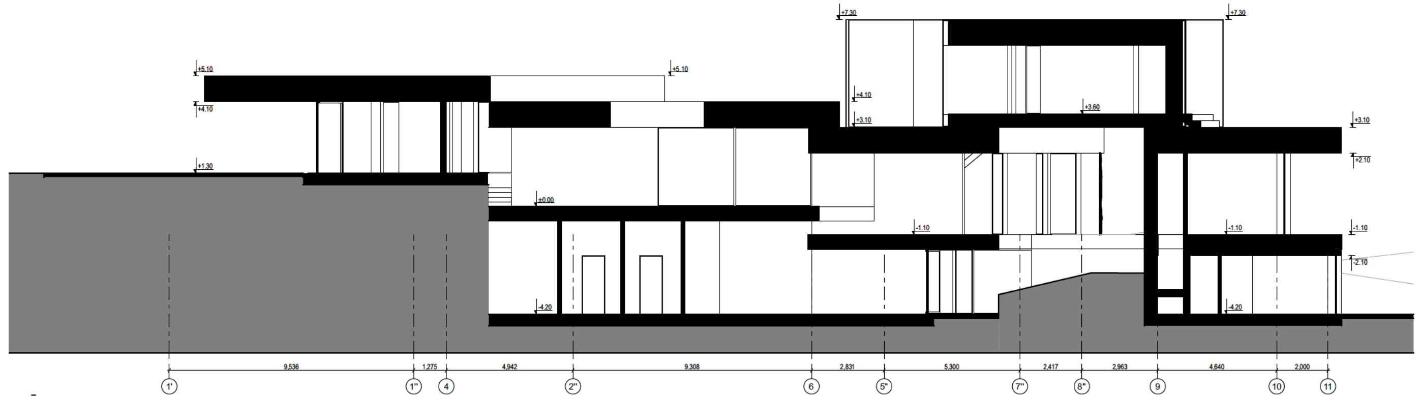
PJŪVIS B-B
