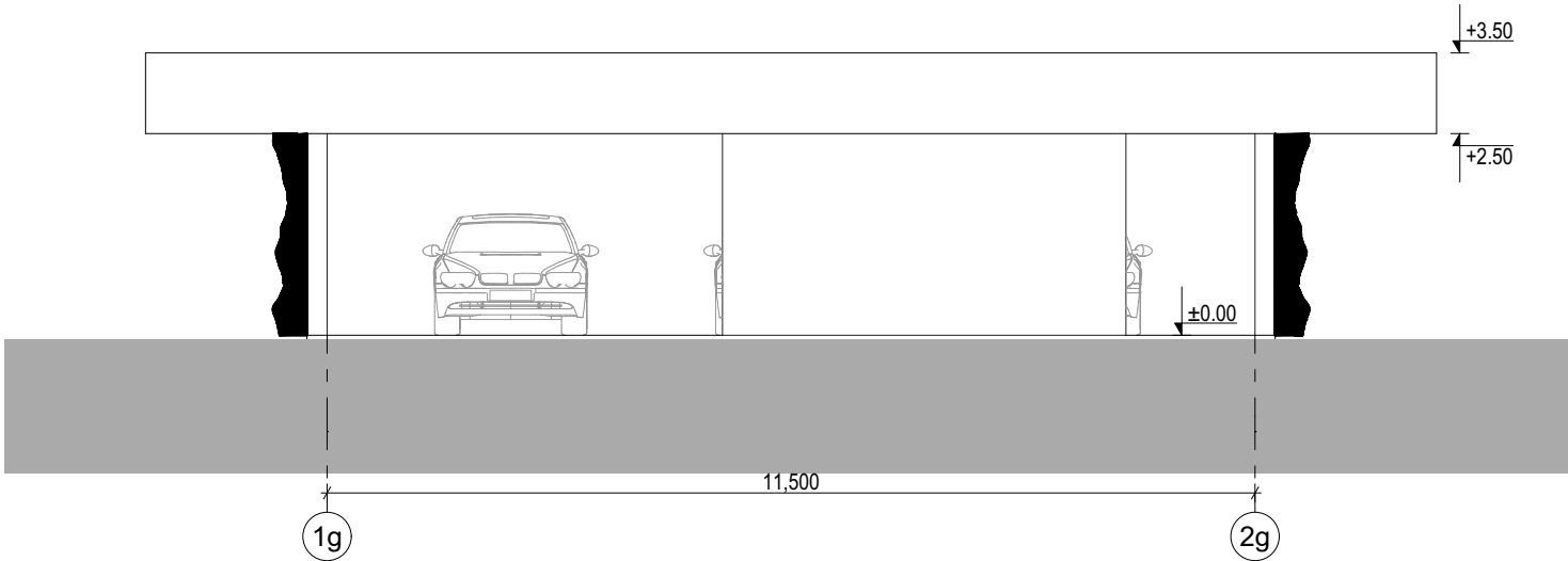
FASADAS 1g2g M 1:100
