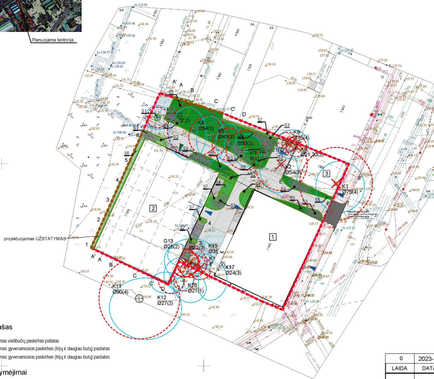
SITUACIJOS SCHEMA
