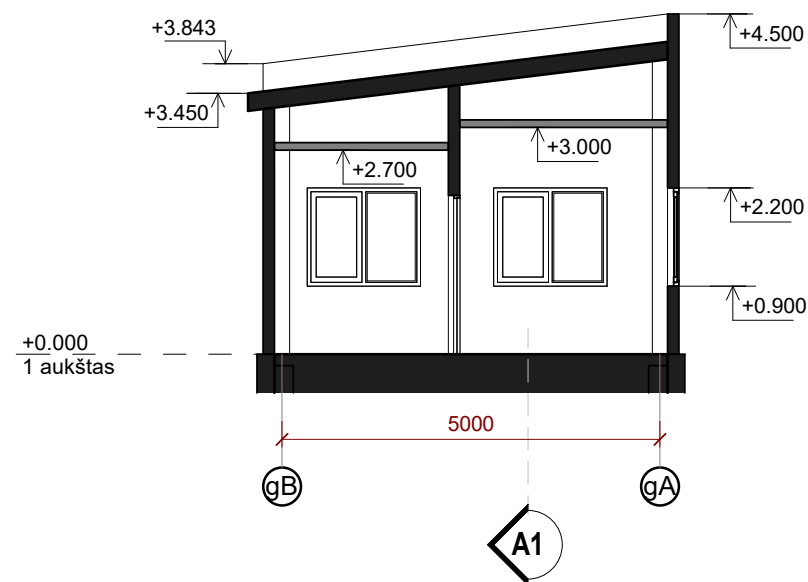
PJŪVIS A2
