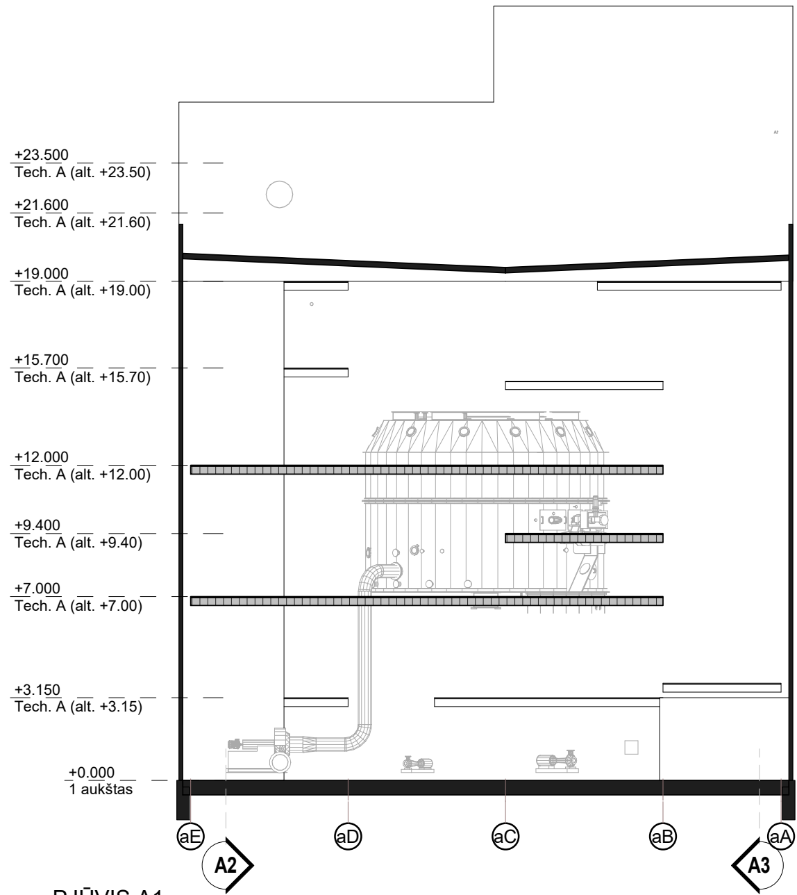
PJŪVIS A1
