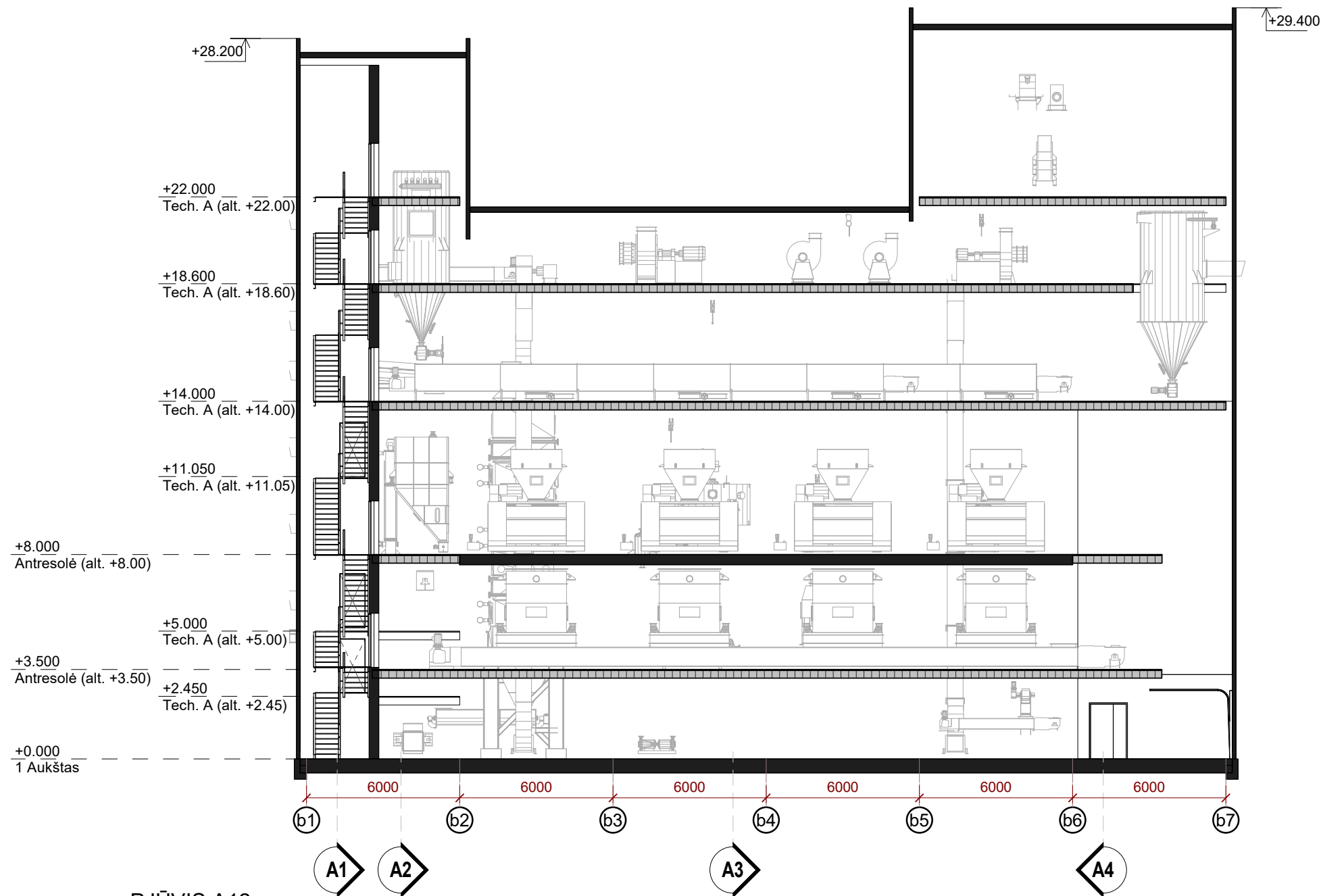
PJŪVIS A12 1 : 200
