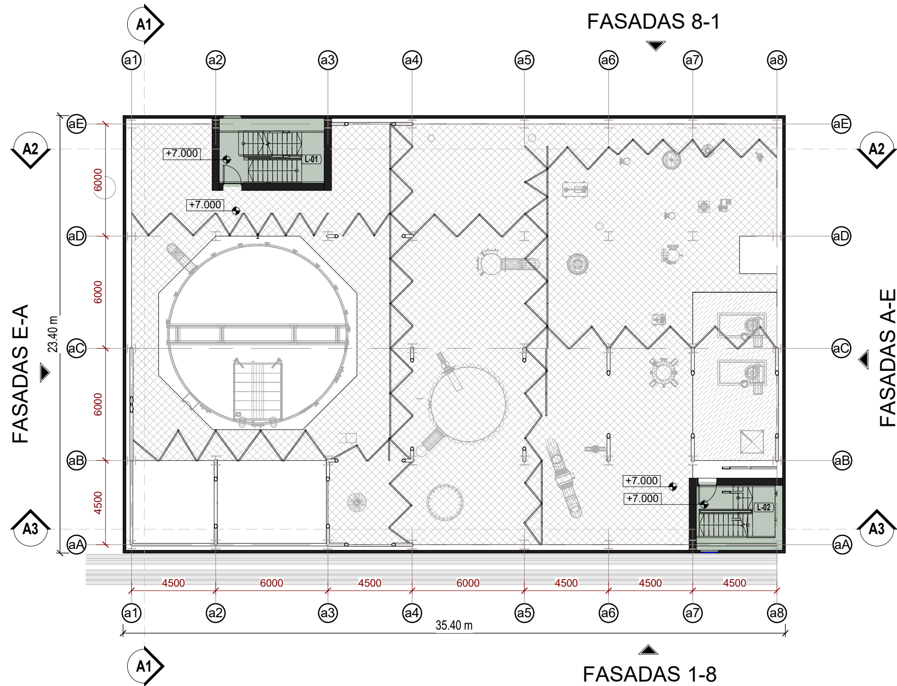
PLANAS 1 : 200
