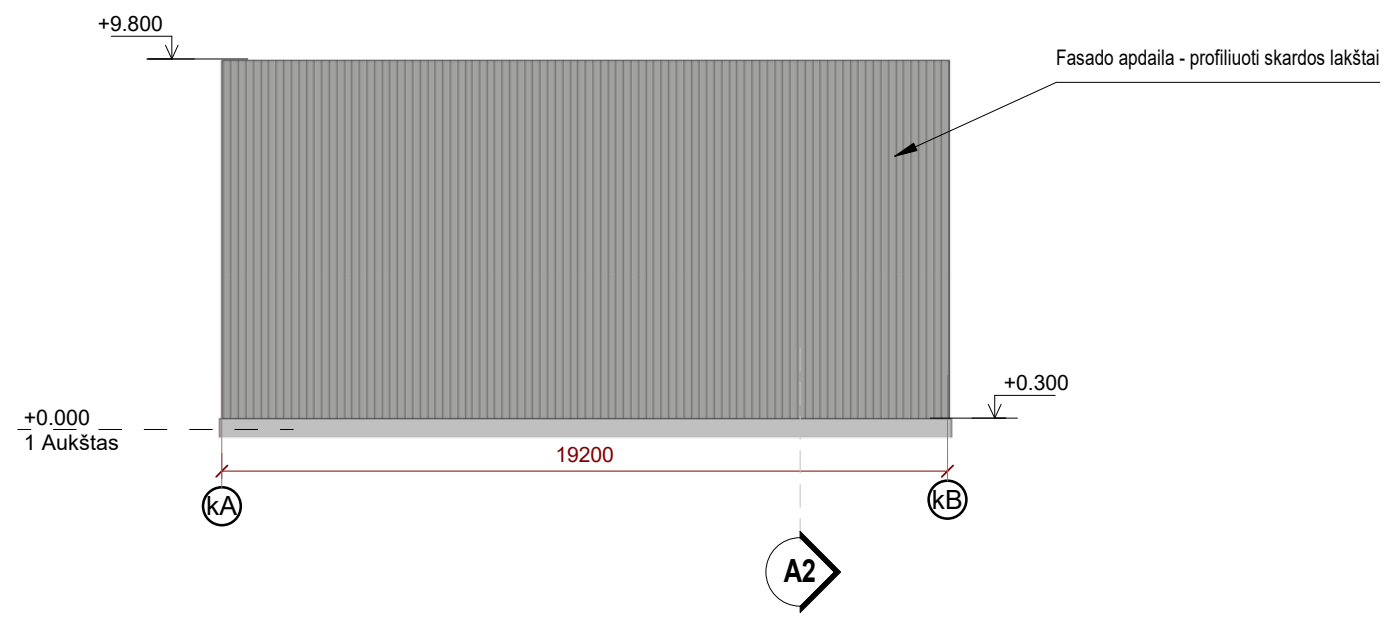
FASADAS A-B
