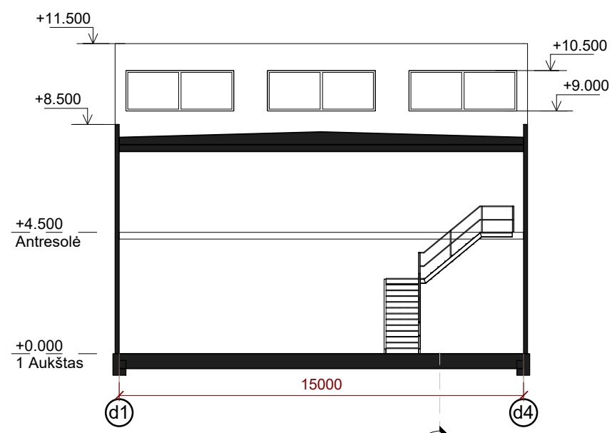
PJŪVIS A2 1 : 200
