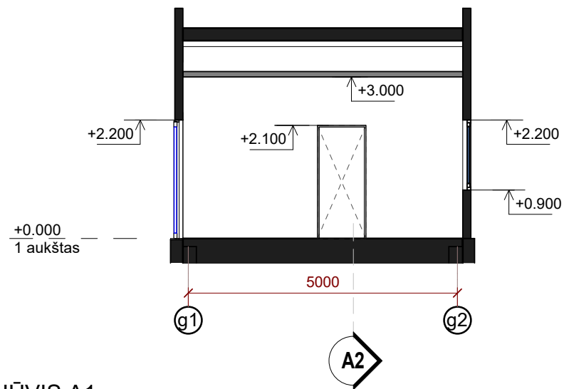
PJŪVIS A1
