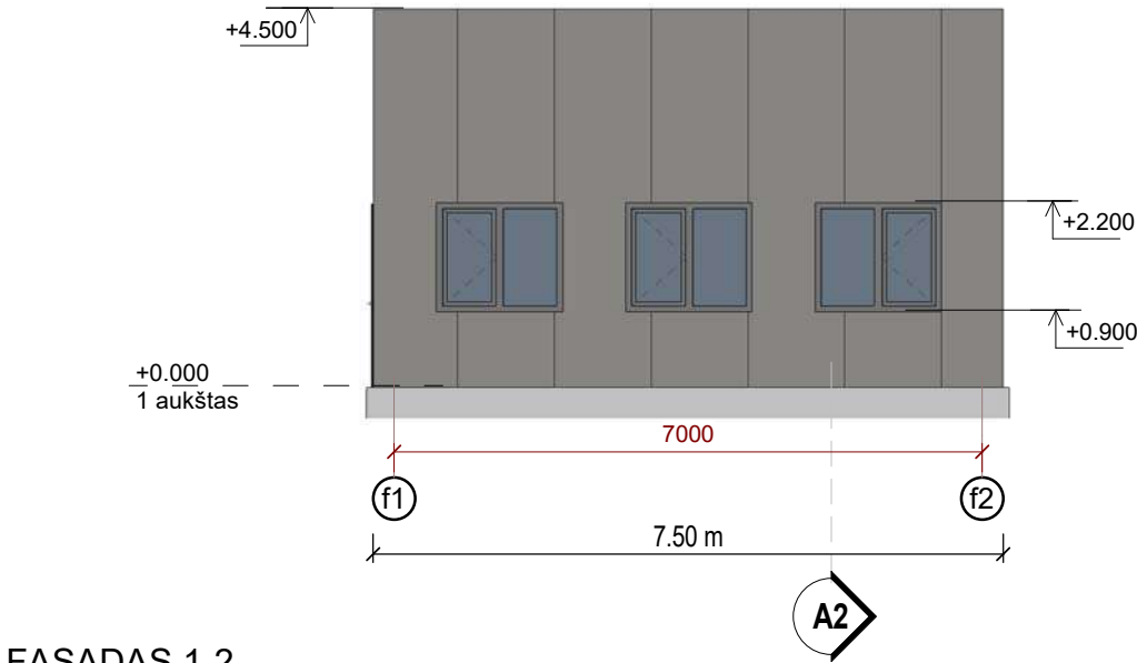
FASADAS 1-2 1 : 100
