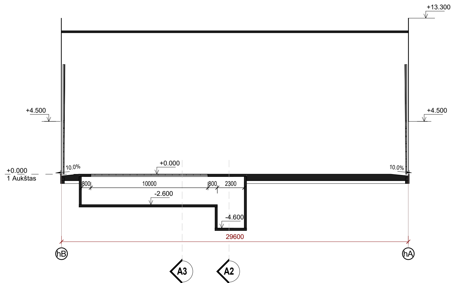
PJŪVIS A1 1 : 200
