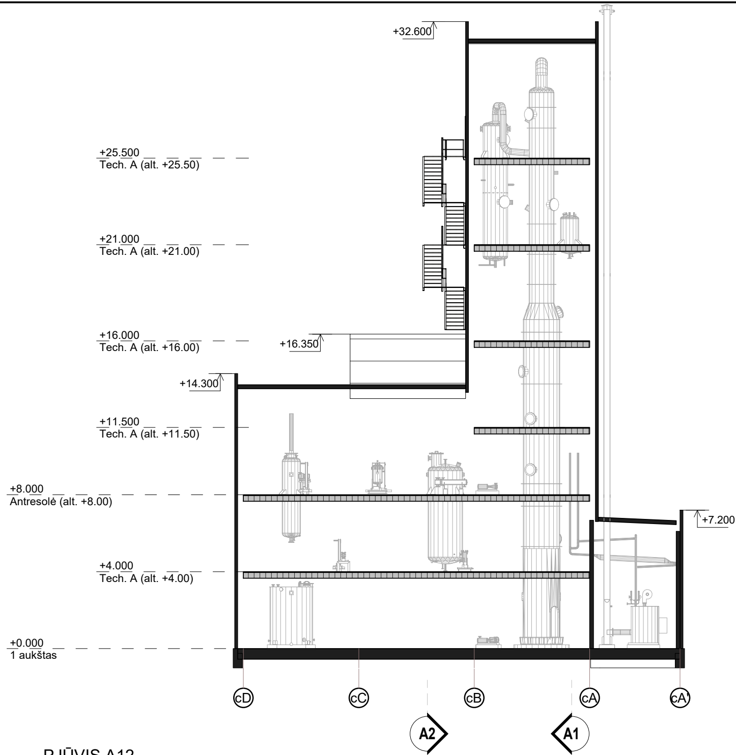
PJŪVIS A12 1 : 200
