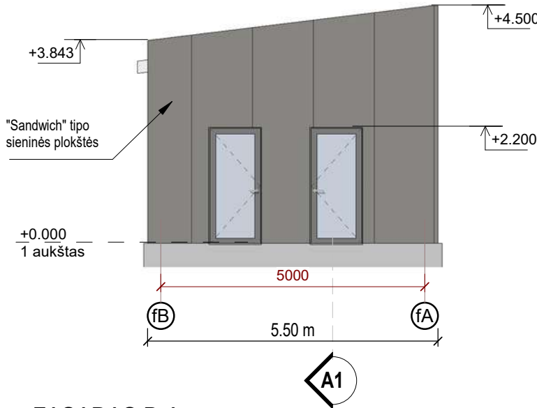
FASADAS B-A 1 : 100
