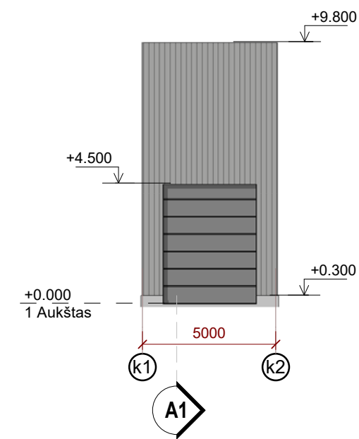
FASADAS 1-2
