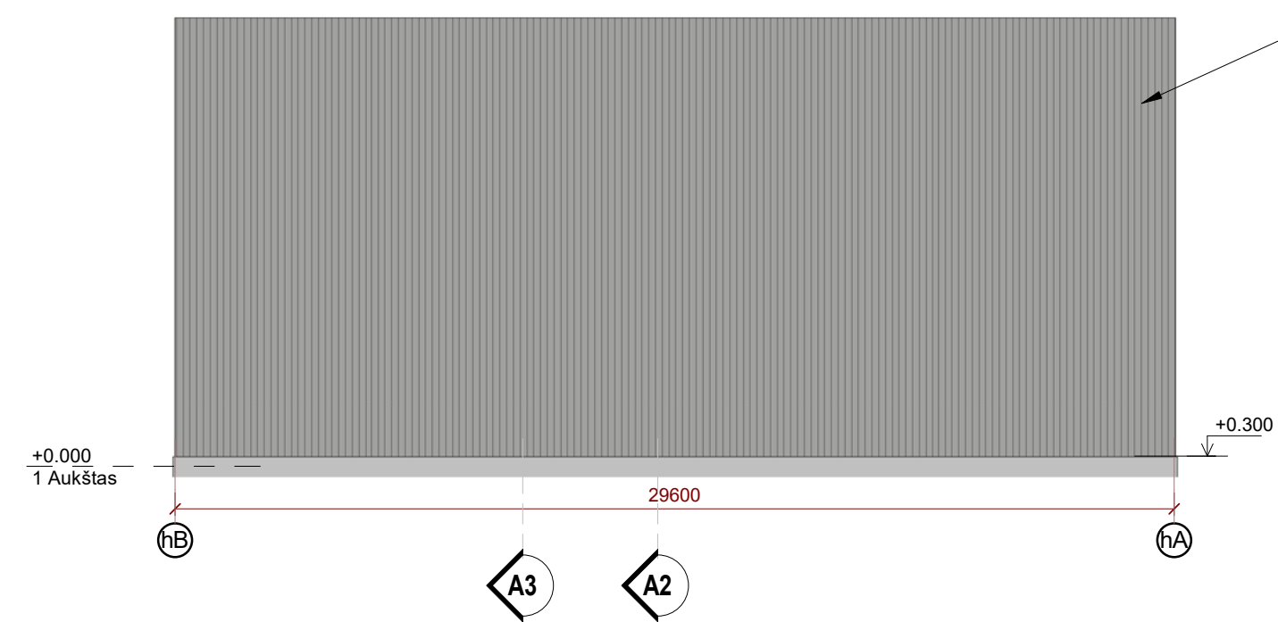
FASADAS B-A 1 : 200
