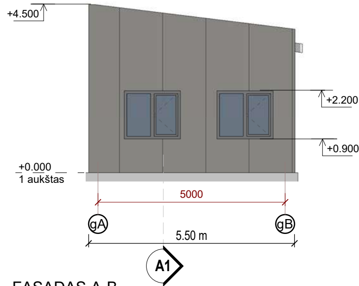
FASADAS A-B
