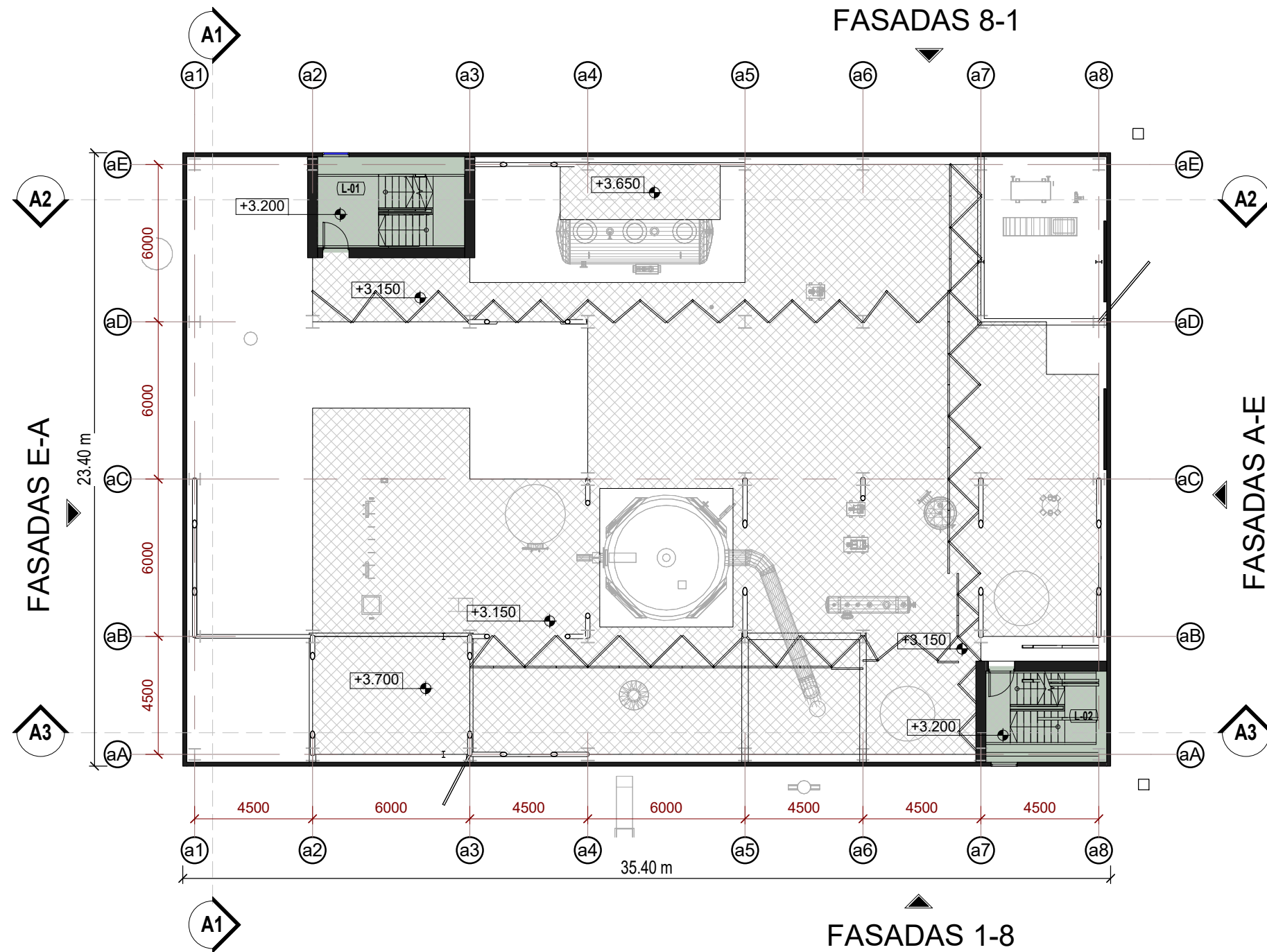
PLANAS 1 : 200
