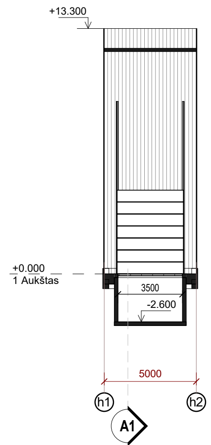
PJŪVIS A3 1 : 200
