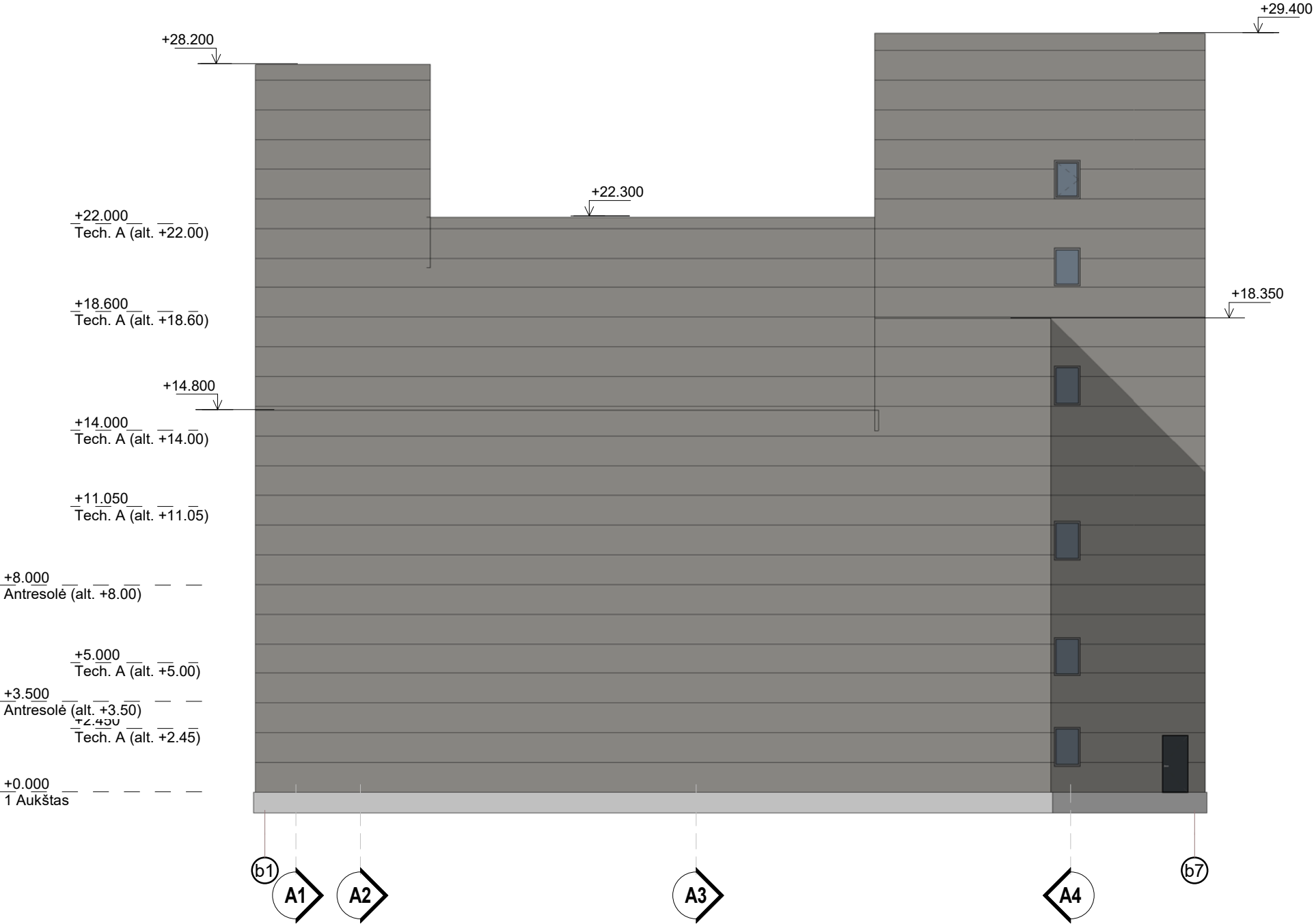
FASADAS 1-7 1 : 200
