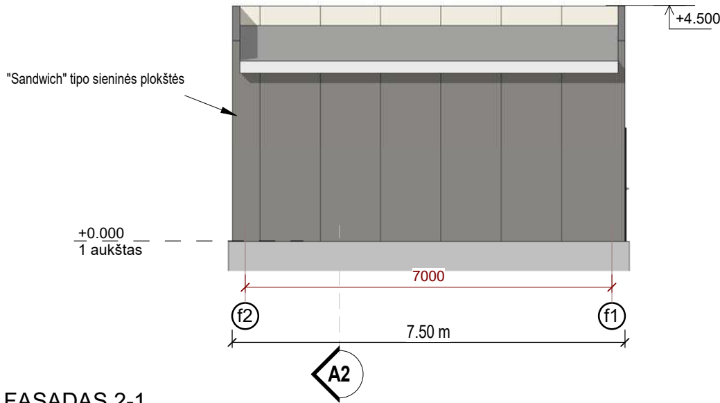
FASADAS 2-1 1 : 100
