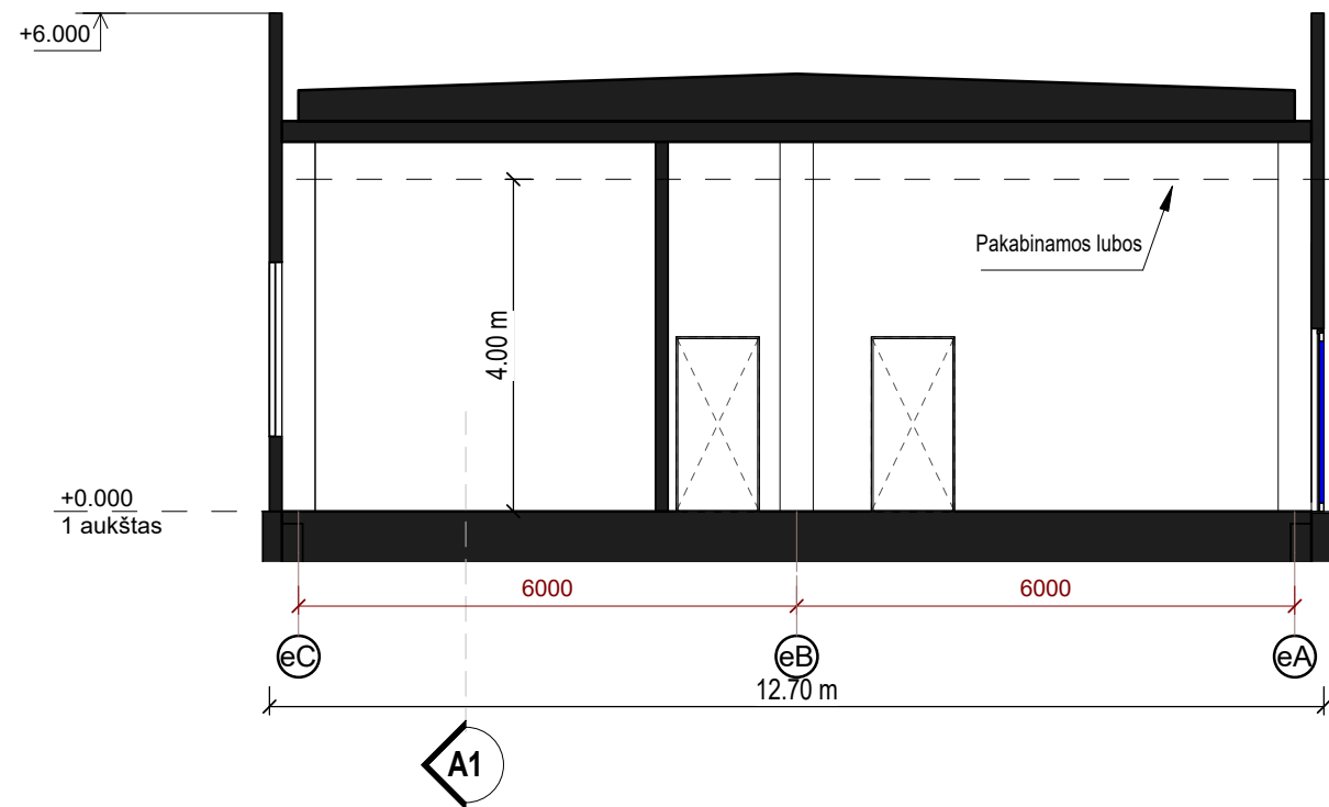
PJŪVIS A2 1 : 100
