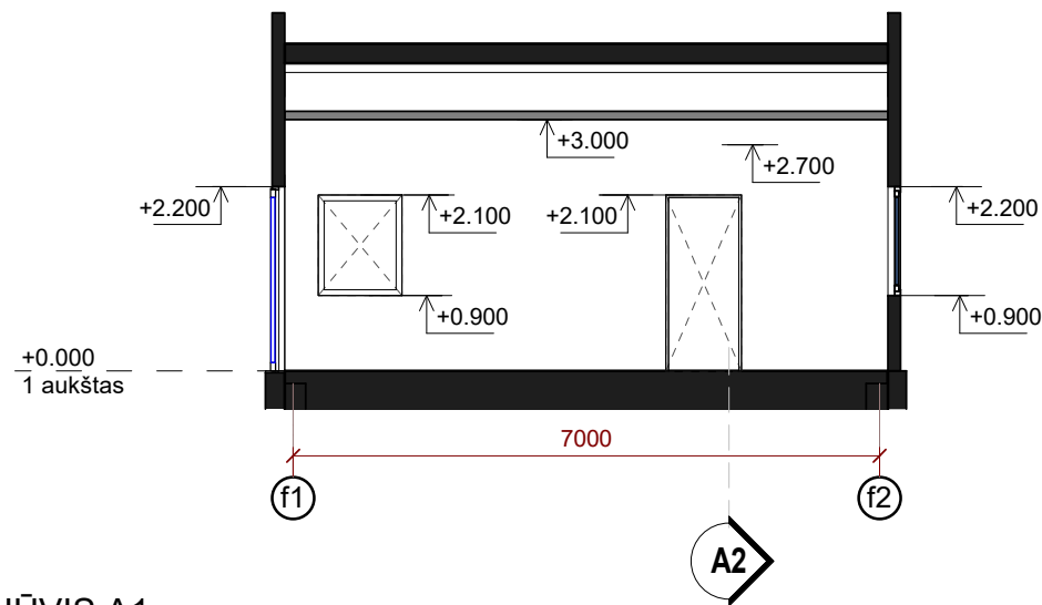
PJŪVIS A1
