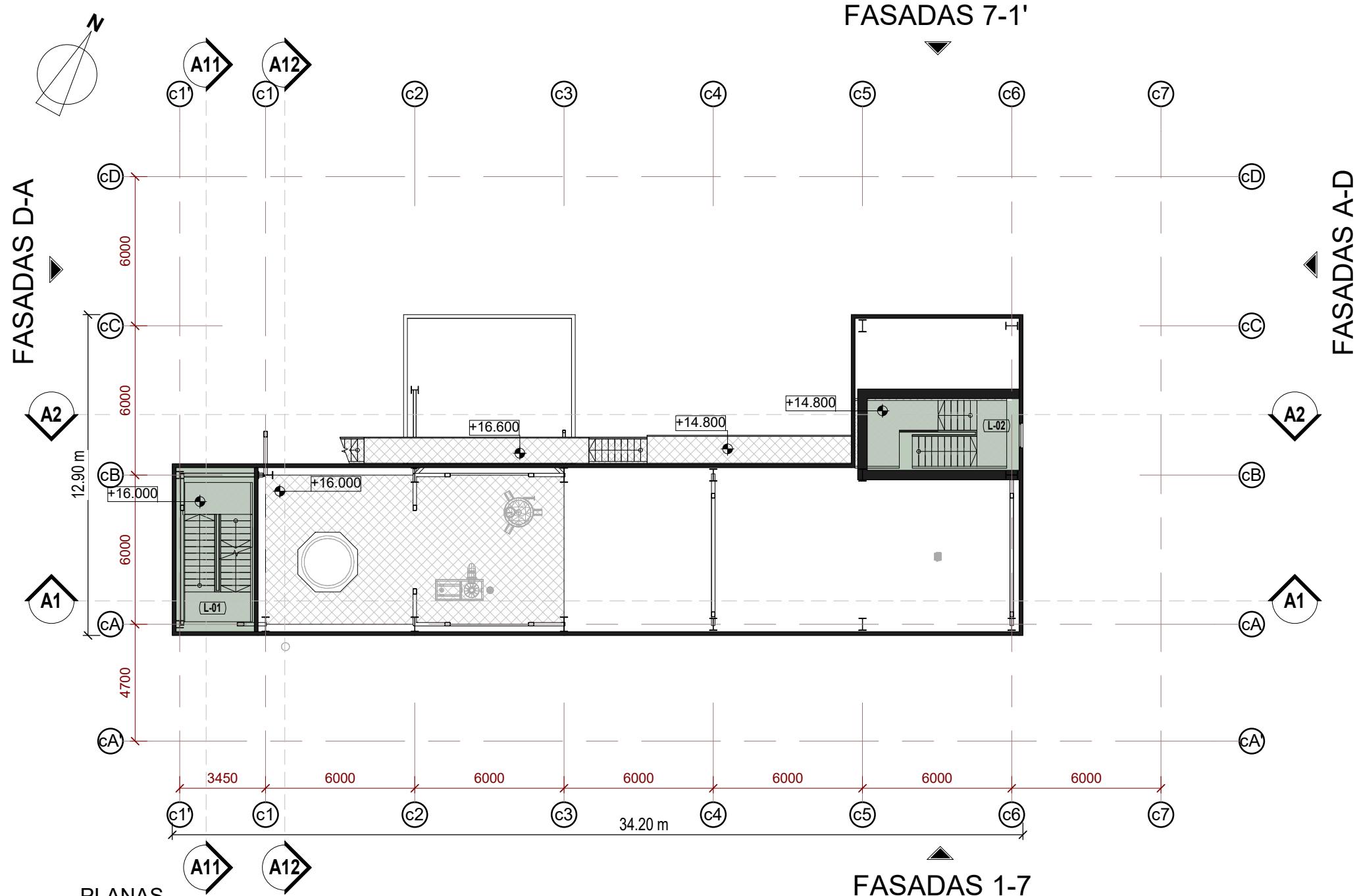
PLANAS 1 : 200
