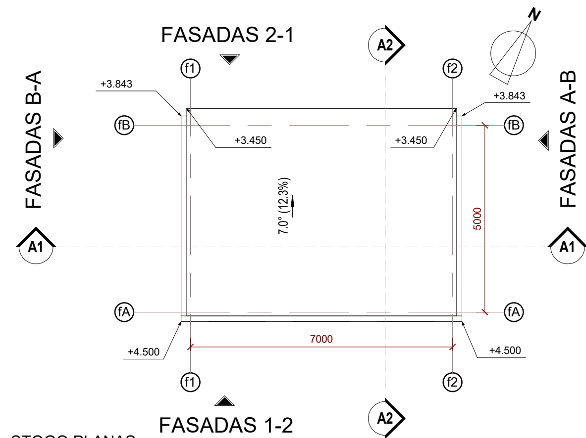
STOGO PLANAS
