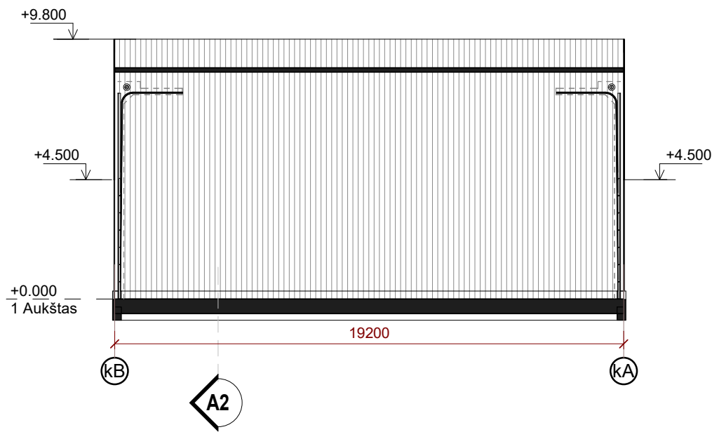
PJŪVIS A1 1 : 200
