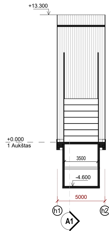
PJŪVIS A2 1 : 200
