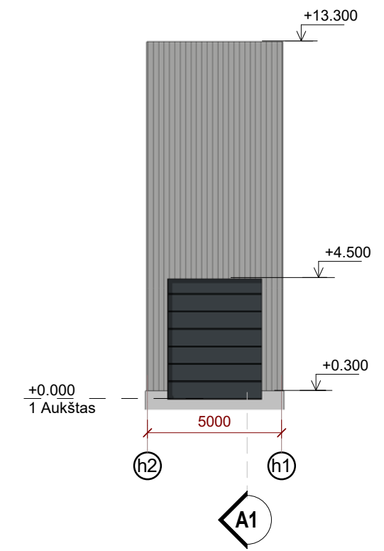
FASADAS 2-1 1 : 200
