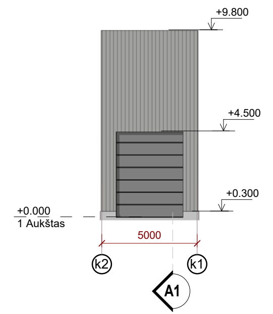
FASADAS 2-1
