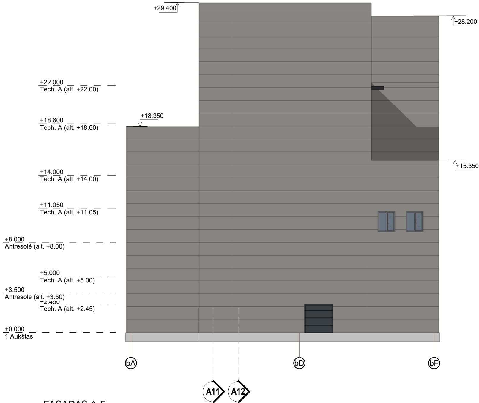
FASADAS A-F 1 : 200
