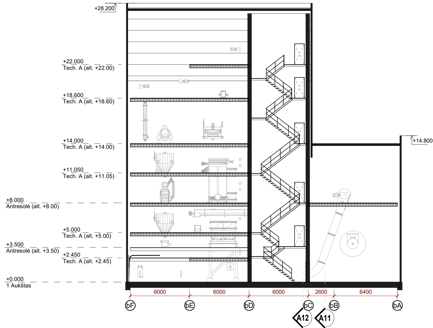
PJŪVIS A1
