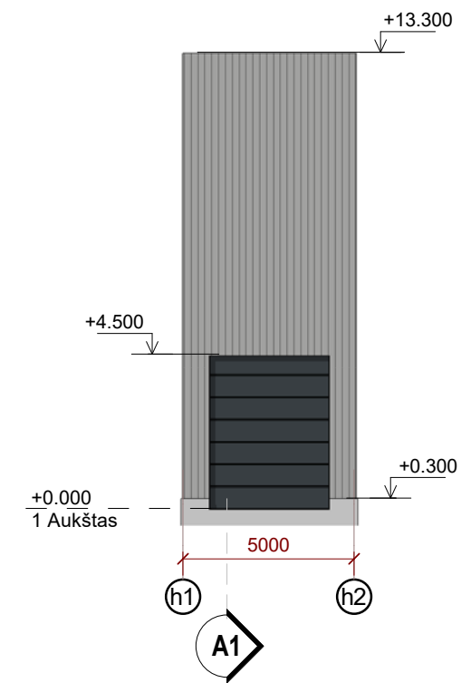
FASADAS 1-2 1 : 200
