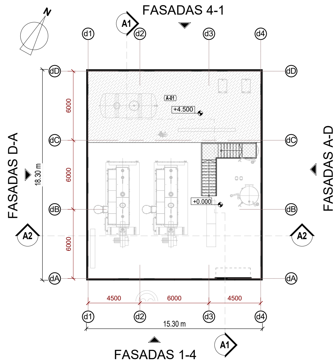
ANTRESOLĖS PLANAS
