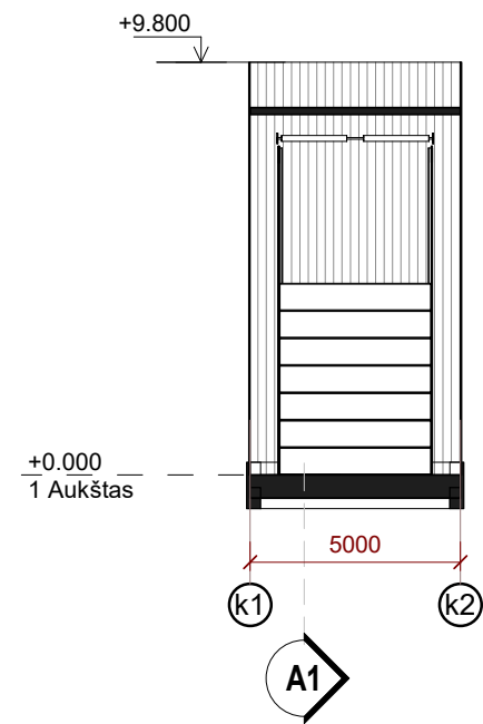
PJŪVIS A2 1 : 200
