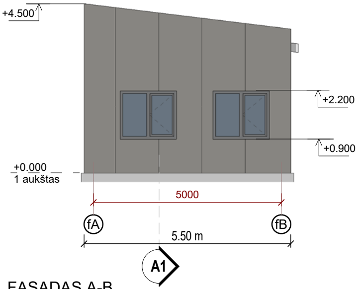
FASADAS A-B 1 : 100
