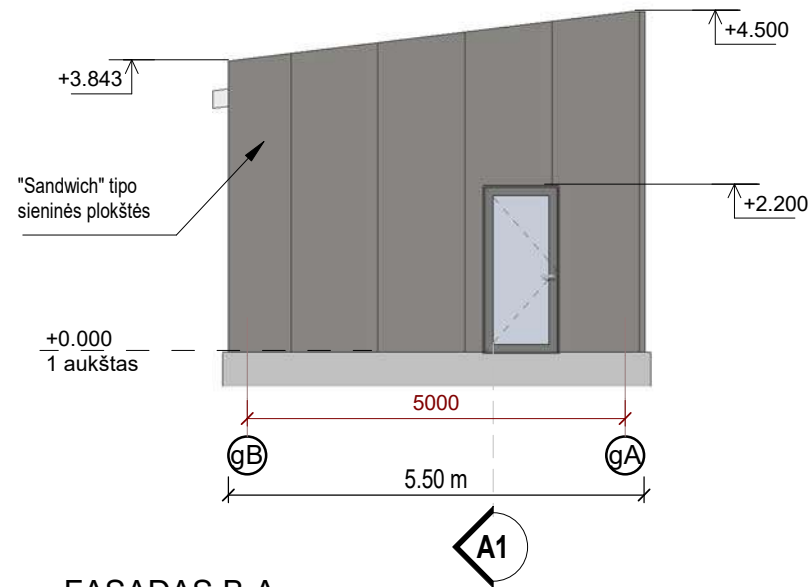
FASADAS B-A
