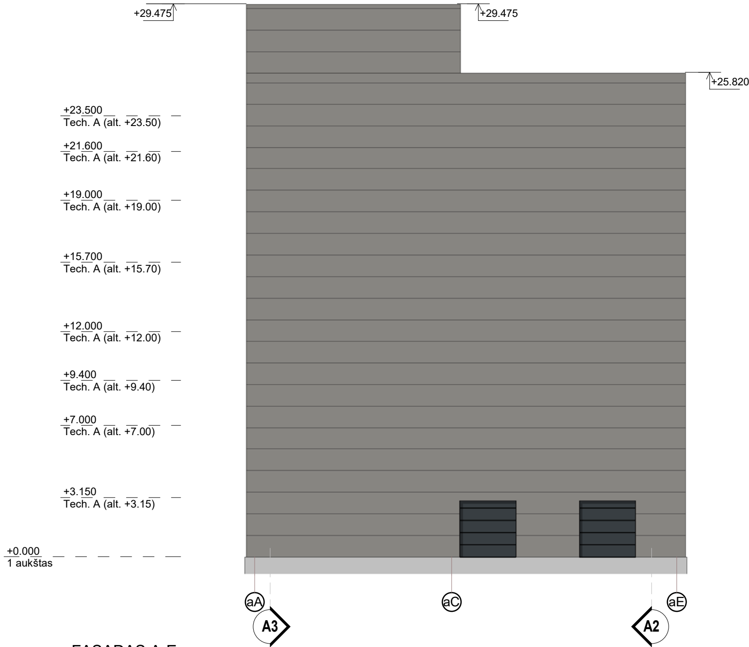
FASADAS A-E 1 : 200
