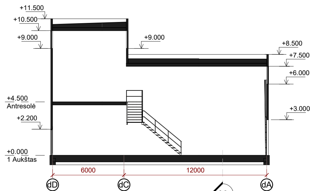
PJŪVIS A1 1 : 200
