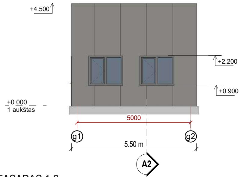
FASADAS 1-2
