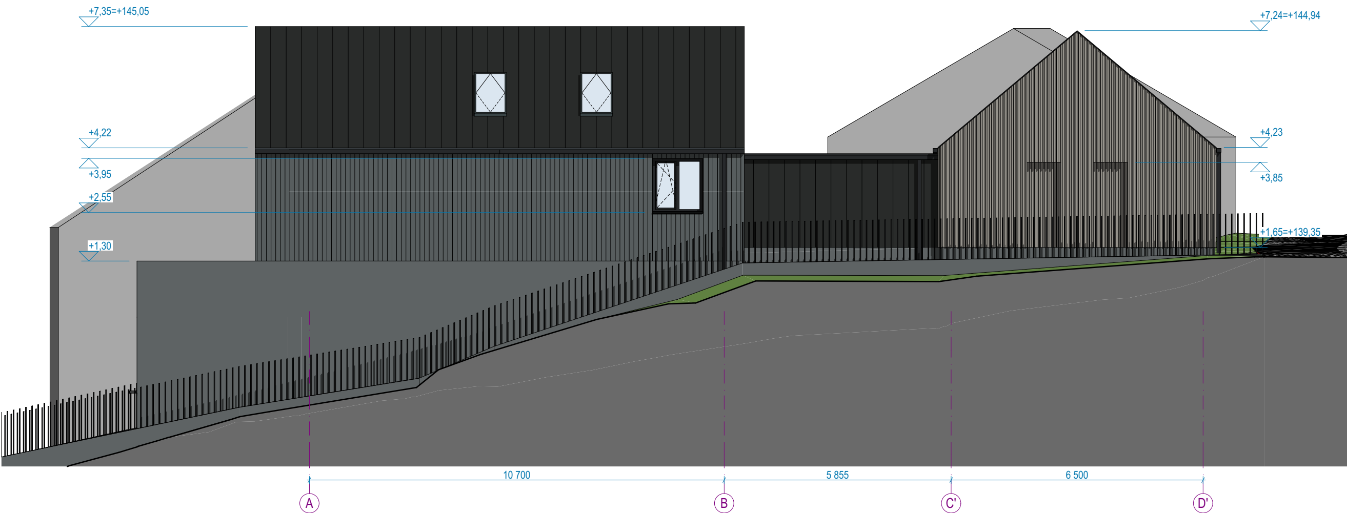
E-03 FASADAS TARP AŠIŲ A-D' 1:100
