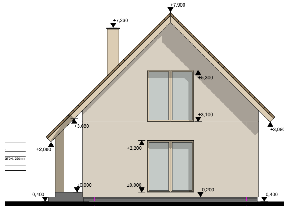
1 FASADAS AŠYSE 1-3 M 1:100
