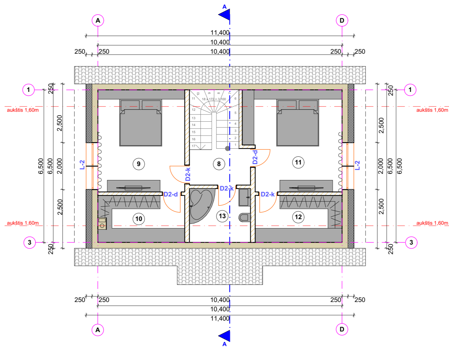
MANSARDOS PLANAS SU BALDAIS M1:100
