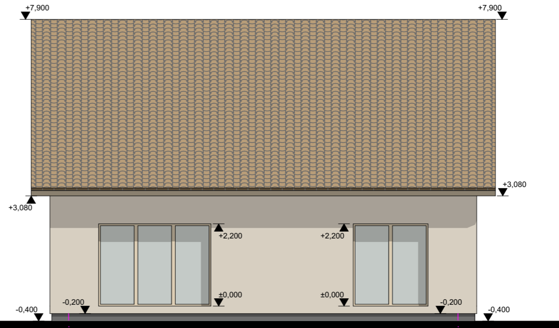
B FASADAS AŠYSE B-A M 1:100
