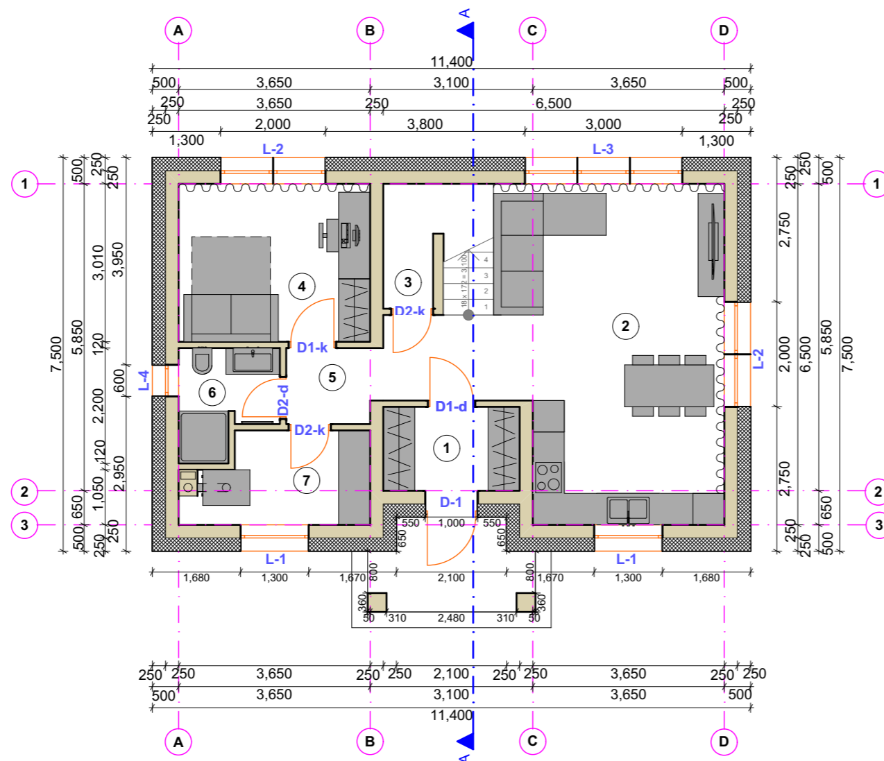
PIRMO AUKŠTO PLANAS SU BALDAIS M1:100
