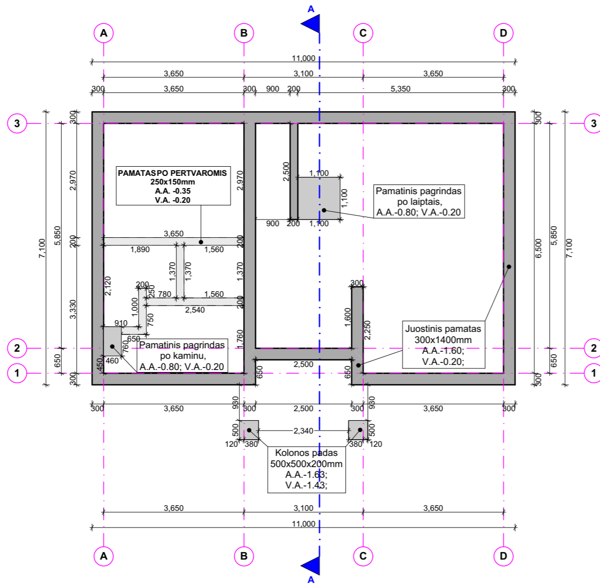
ESAMŲ PAMATO SUSITIPINIMO IR NAUJO PAMATO PLANAS M1:100
