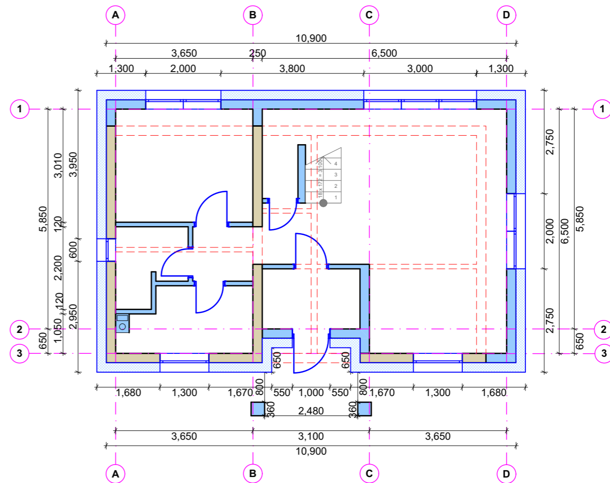
REKONSTRAVIMO SCHEMA M1:100
