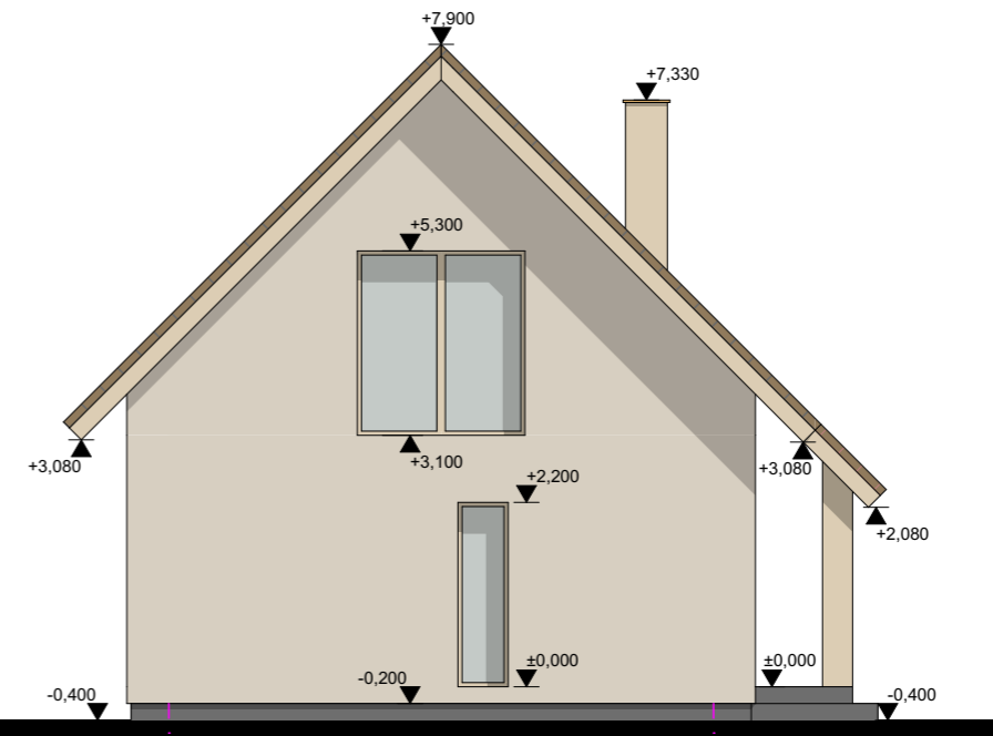
B FASADAS AŠYSE B-A M 1:100
