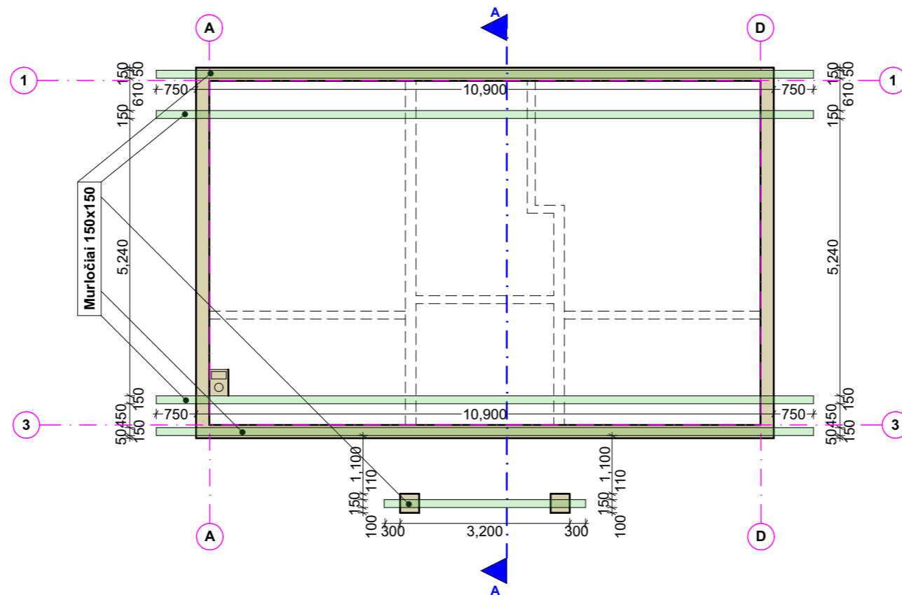
STOGO LAIKANČIŲ KONSTRUKCIJŲ PLANAS M1:100
