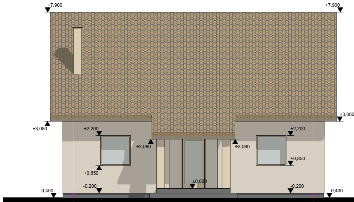
1 FASADAS AŠYSE 1-3 M 1:100
