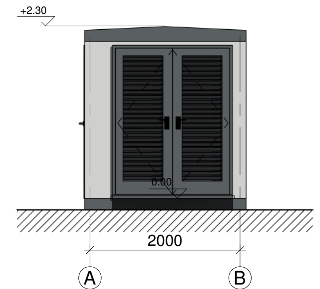
Pietvakarių fasadas 1 : 50
