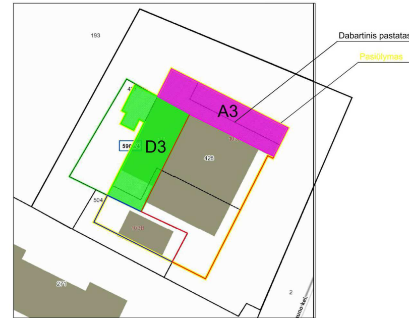
Trečio aukšto planas
