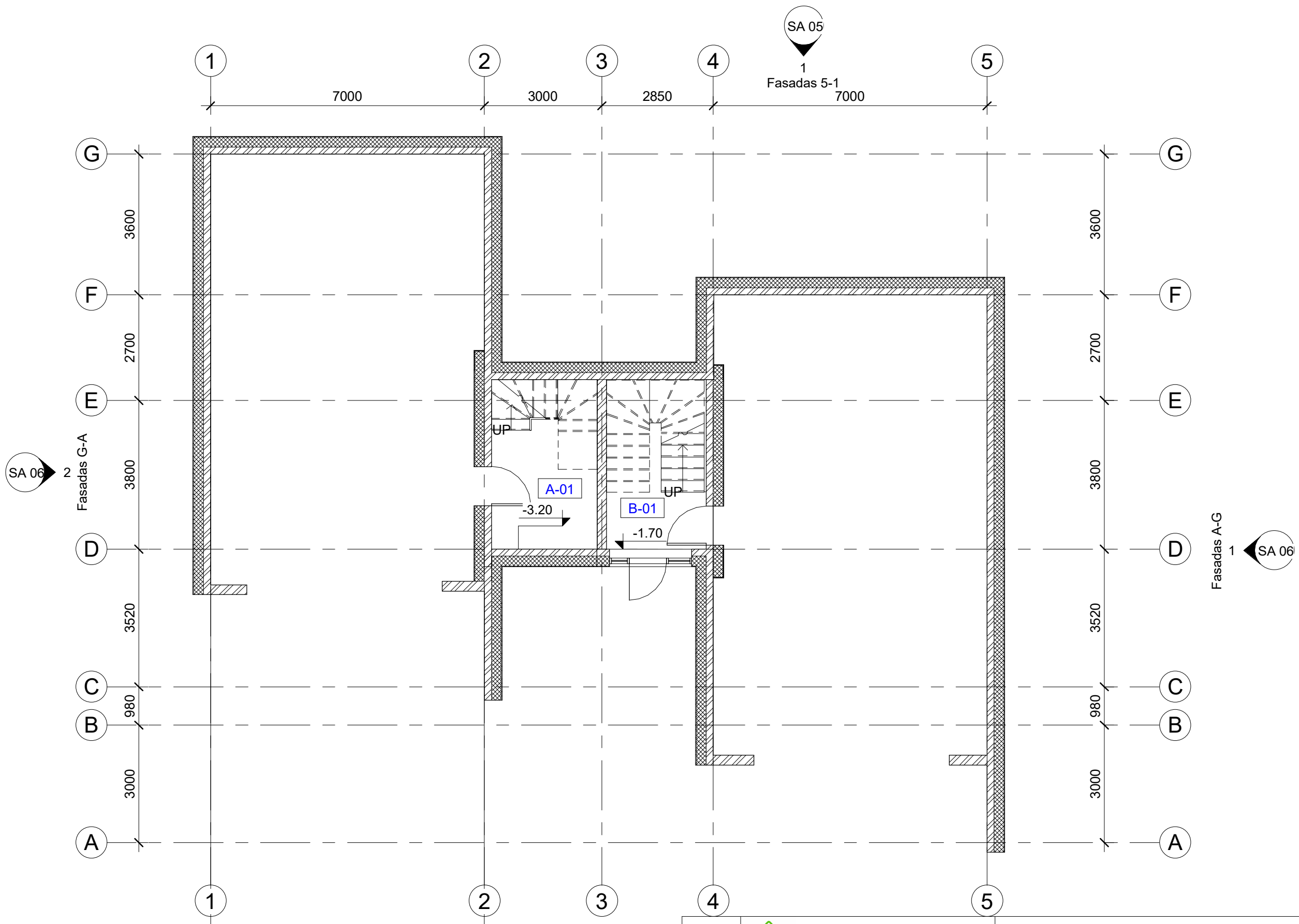
Fasadas 1-5 1 SA 04
