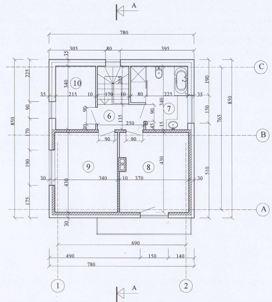
ANTRO AUKŠTO PLANAS M 1:100
