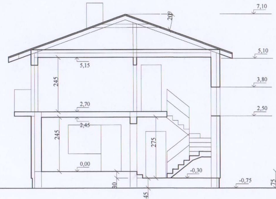
PJŪVIS A-A M 1:100
