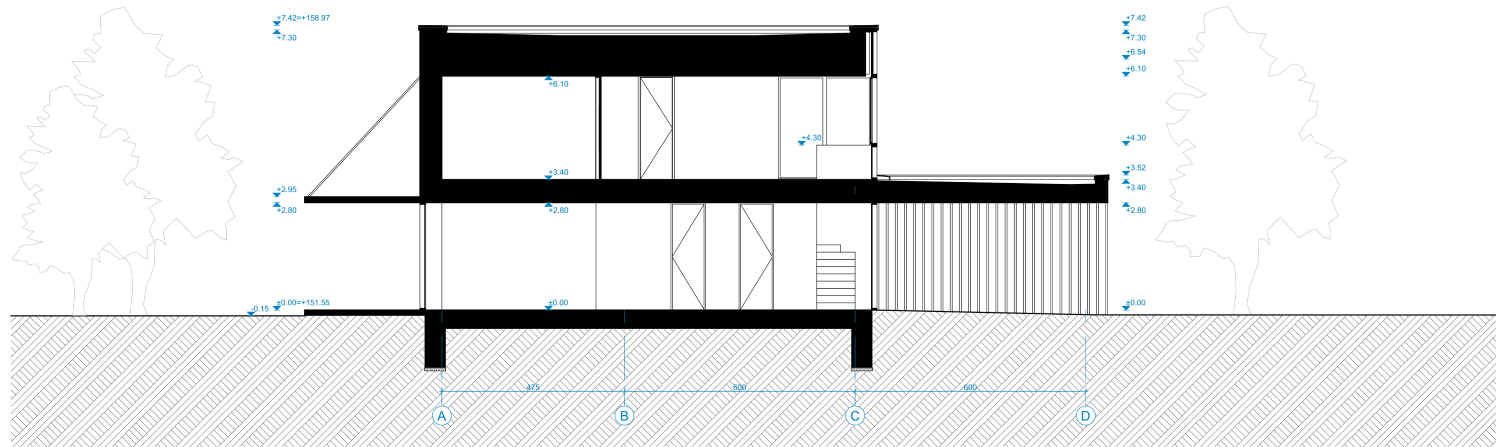
Pjūvis P2
