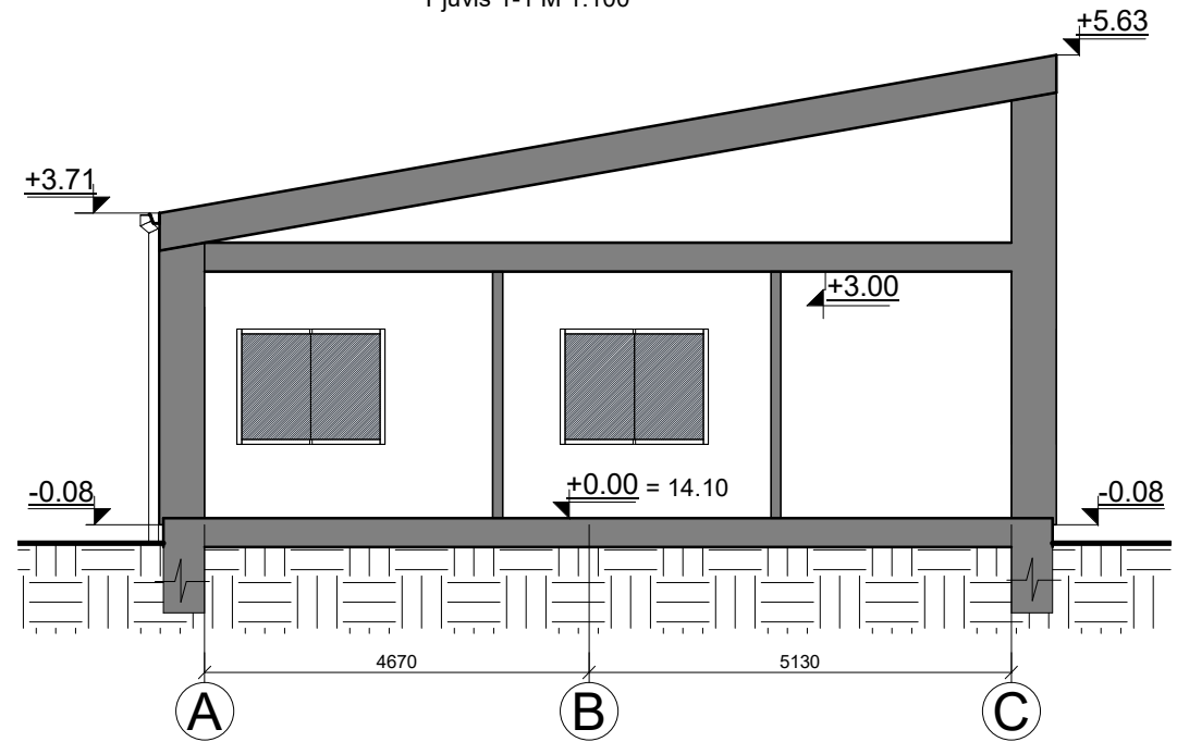
Pjūvis 1-1 M 1:100
