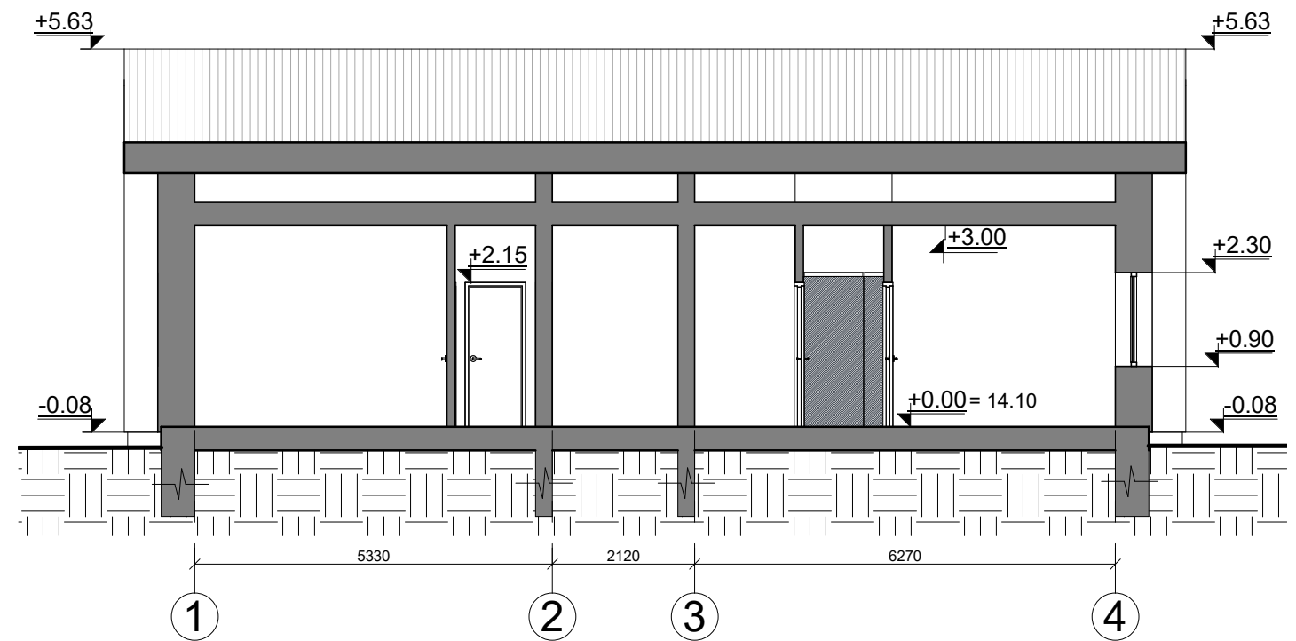
Pjūvis 2-2 M 1:100
