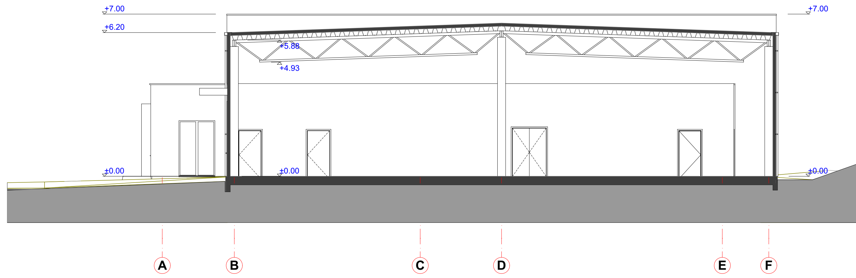
Pjūvis 2-2
