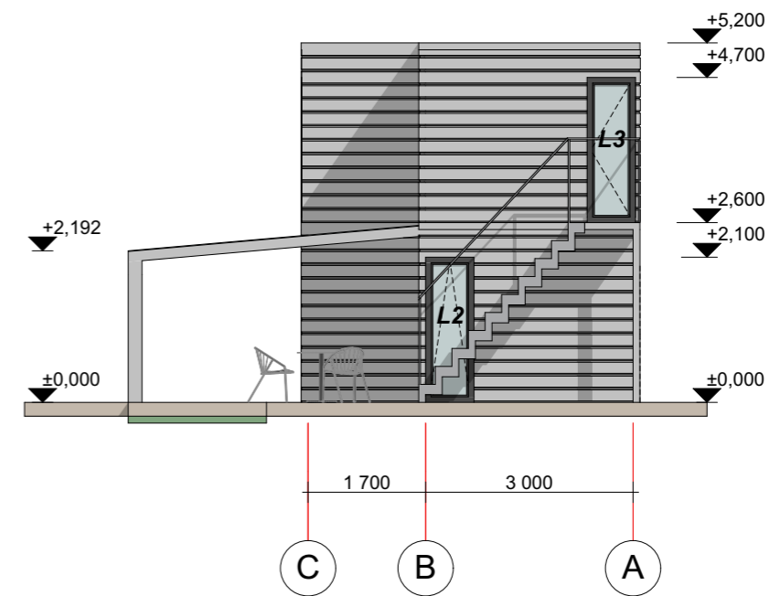
FASADAS C-A
