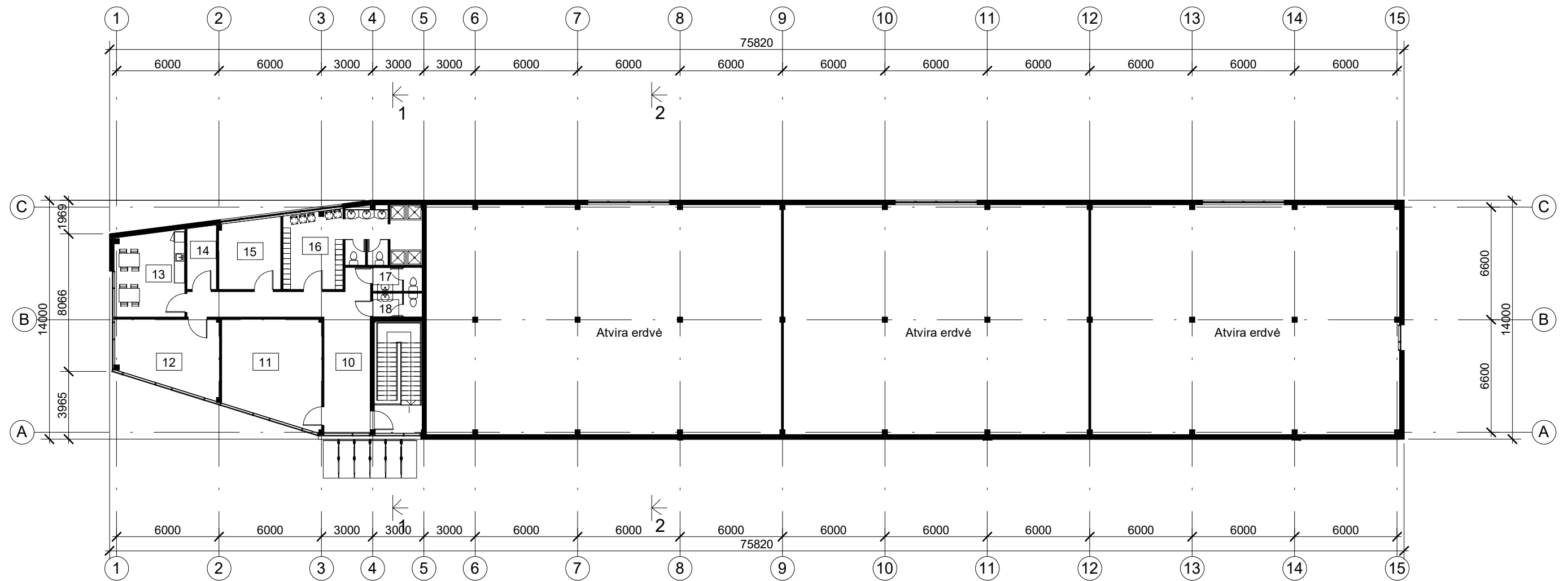
ANTRO AUKŠTO PLANAS M 1:250
