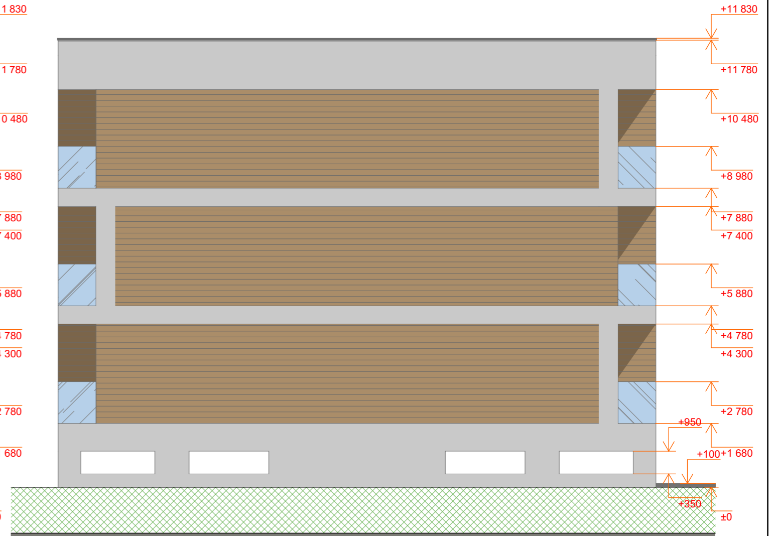
FASADAS TARP AŠIŲ 5-1 M 1:100
