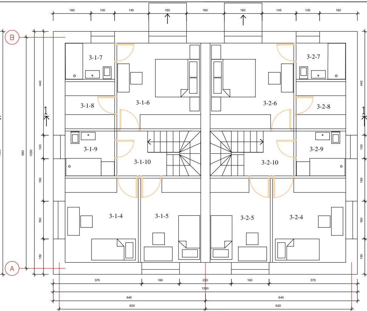
1 Dvibučio Nr.3 2-o aukšto planas 2 3
