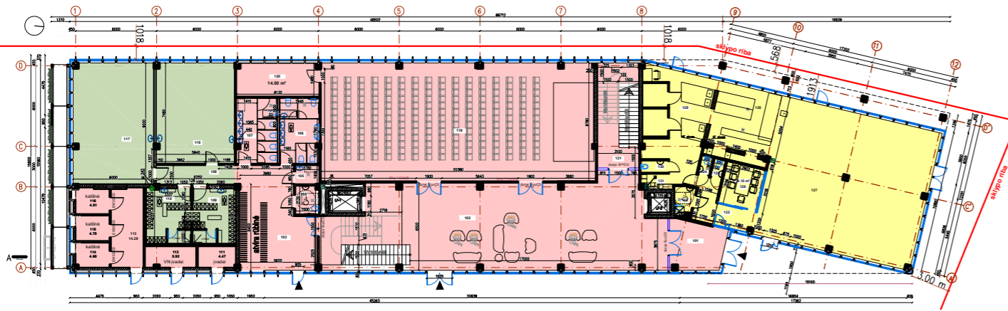
PIRMO AUKŠTO PLANAS-SCHEMA
