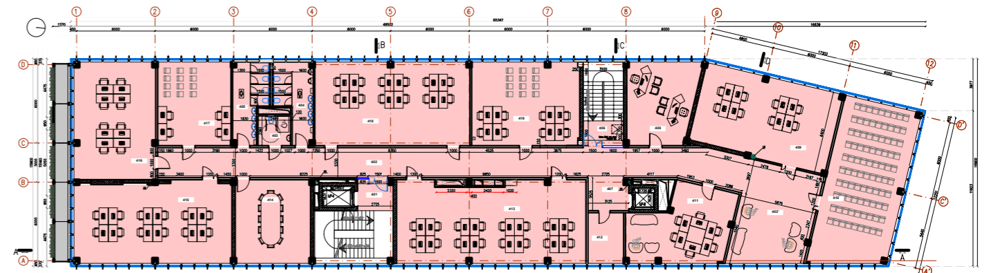
KETVIRTO AUKŠTO PLANAS-SCHEMA
