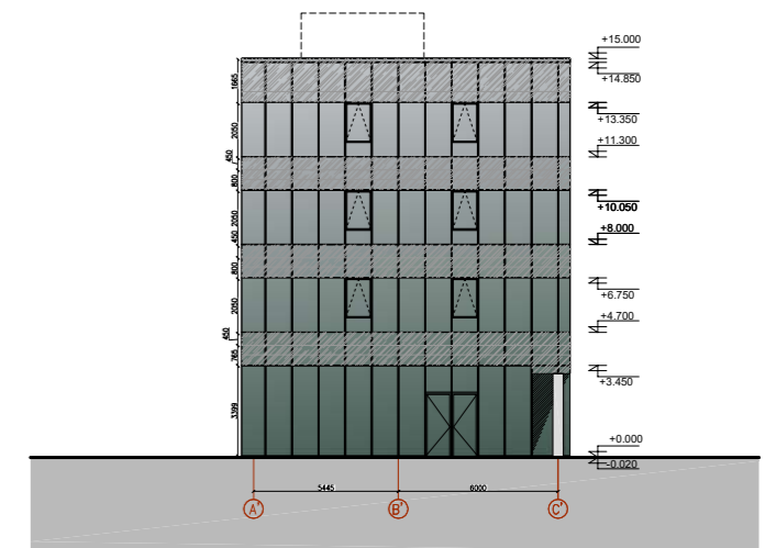
FASADAS IŠ ŠIAURĖS (Europos pr.)
