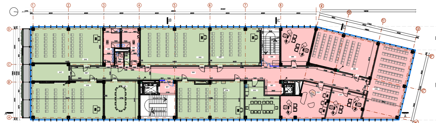
TREČIO AUKŠTO PLANAS-SCHEMA
