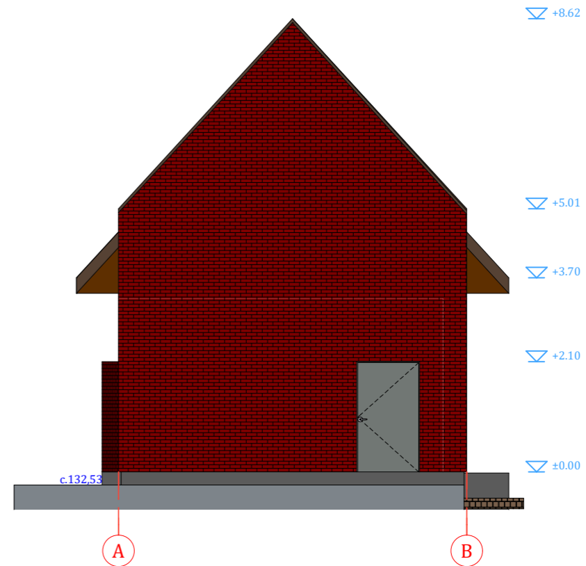
FASADAS AŠYSE A - B M 1 : 100
