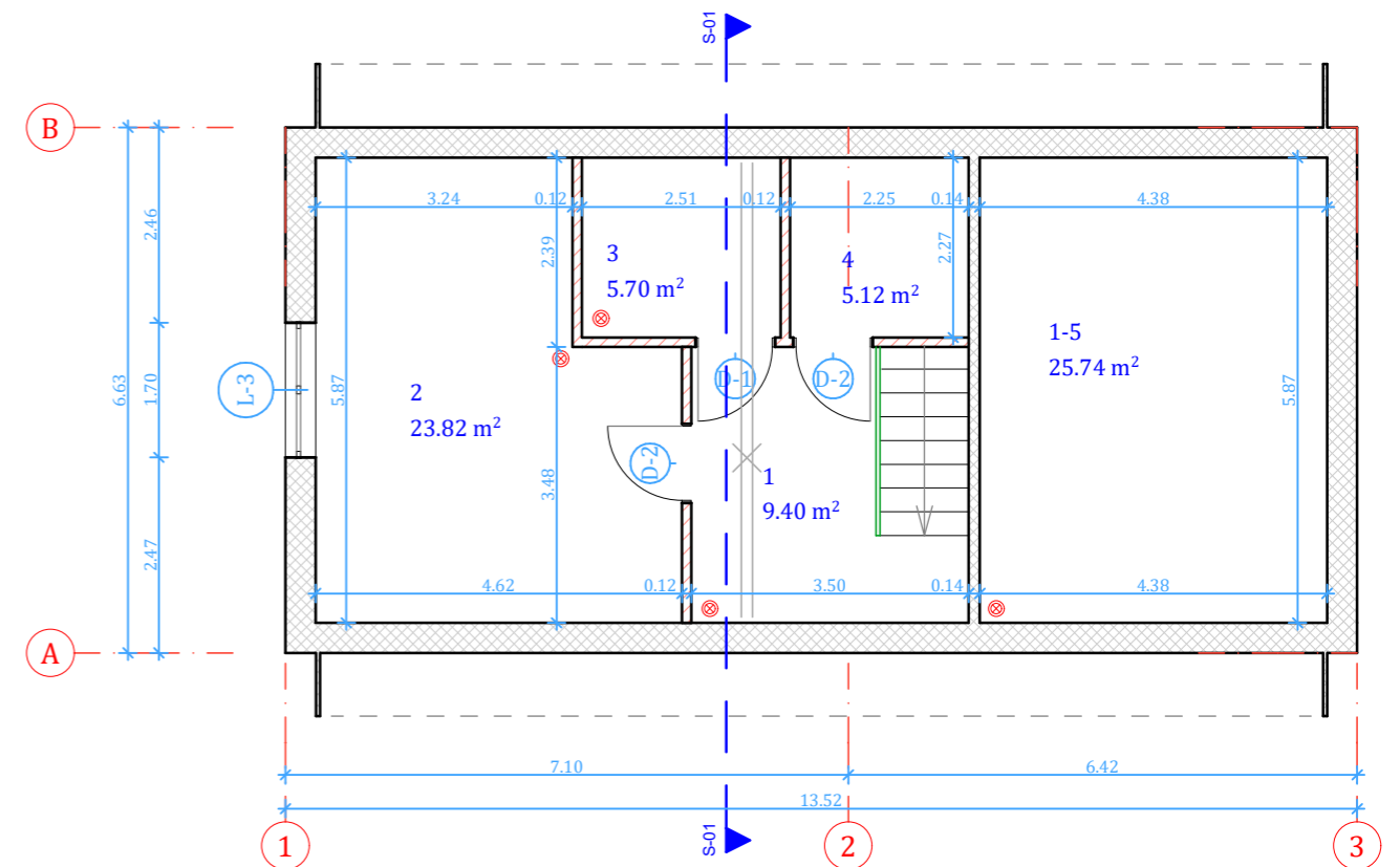
MANSARDOS PLANAS 1 : 100
