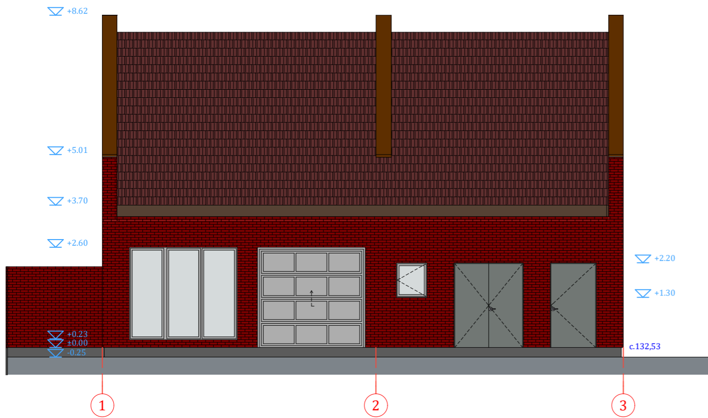
FASADAS AŠYSE B - A M 1 : 100
