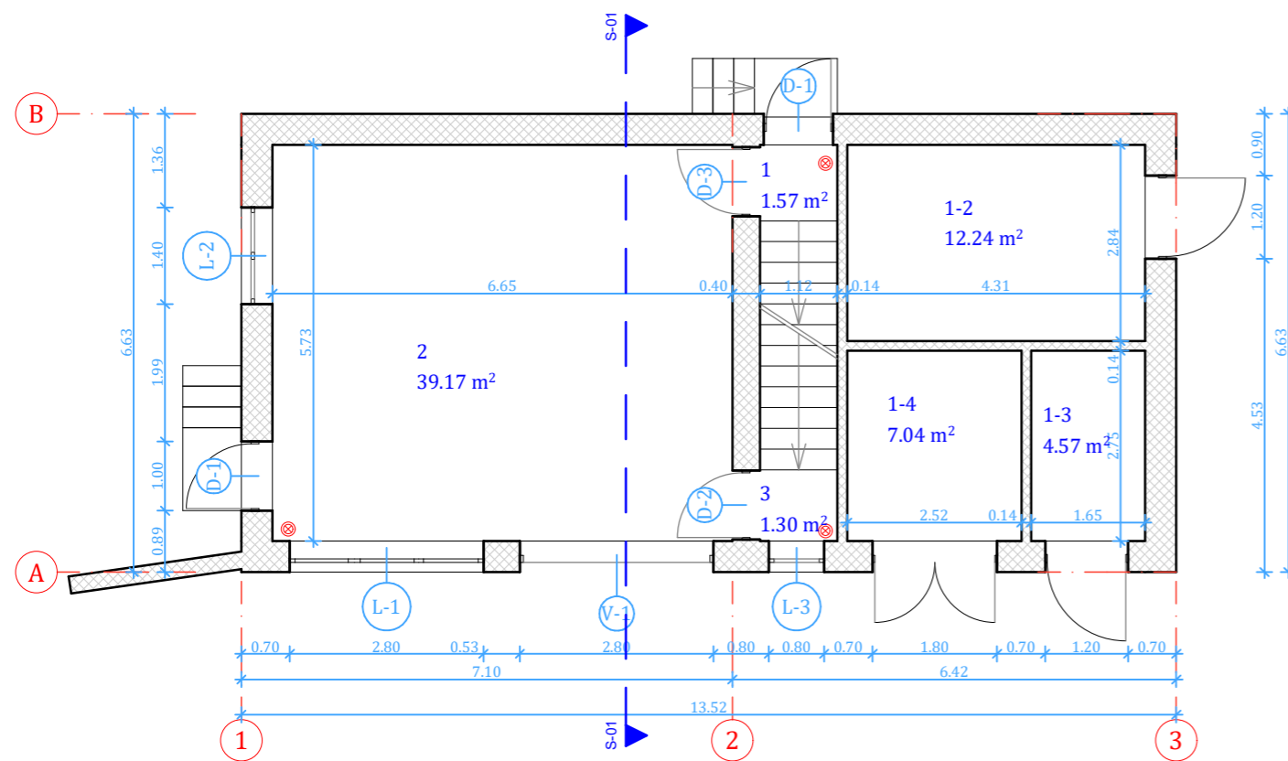
AUKŠTO PLANAS 1 : 100
