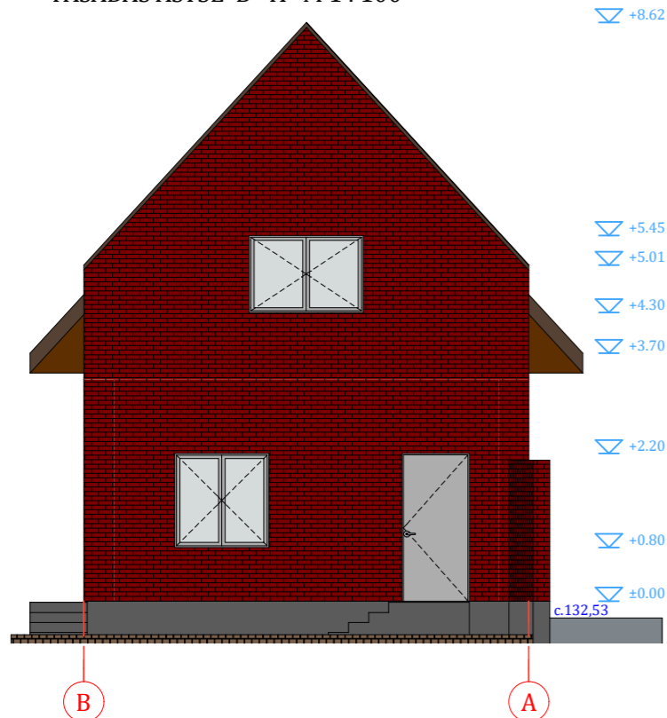
FASADAS AŠYSE B - A M 1 : 100
