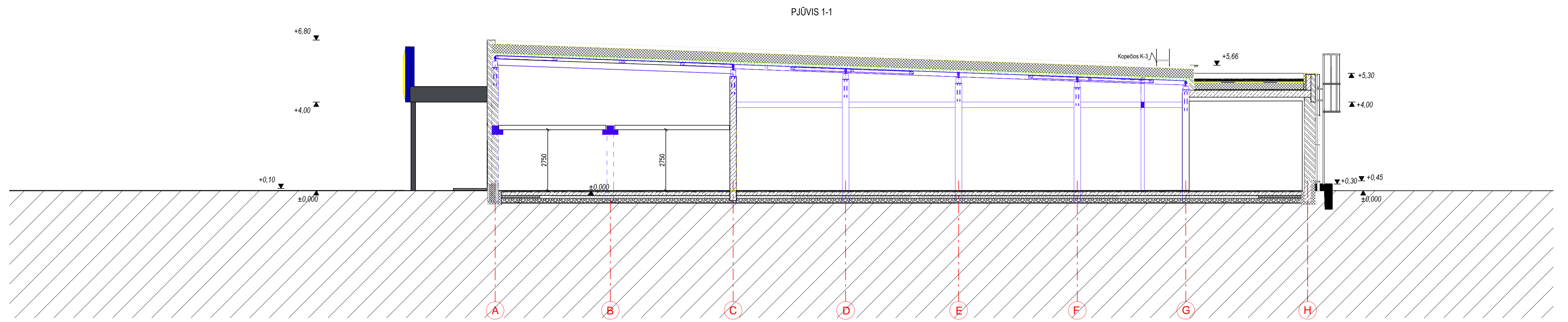
1 | Pjūvis 1-1 1:100
