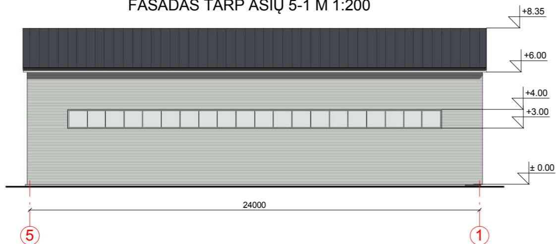
FASADAS TARP AŠIŲ 5-1 M 1:200
