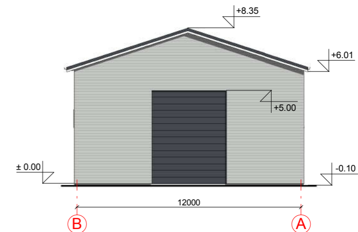
FASADAS TARP AŠIŲ B-A M 1:200
