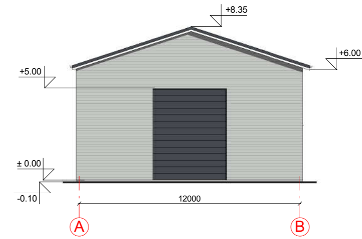
FASADAS TARP AŠIŲ A-B M 1:200
