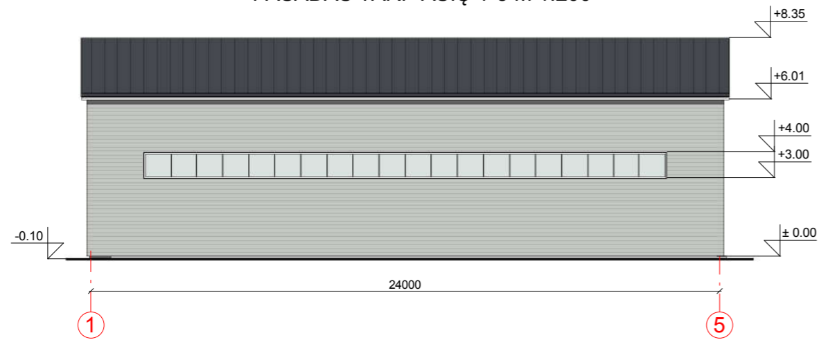
FASADAS TARP AŠIŲ 1-5 M 1:200
