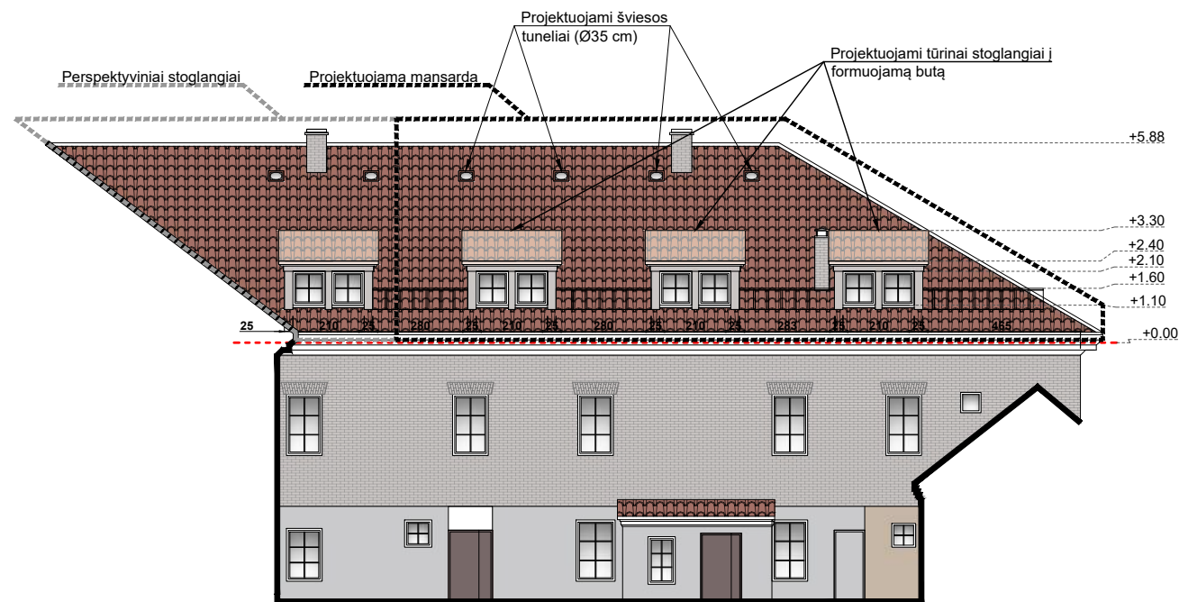
KIEMO FASADAS 2, M 1:200
