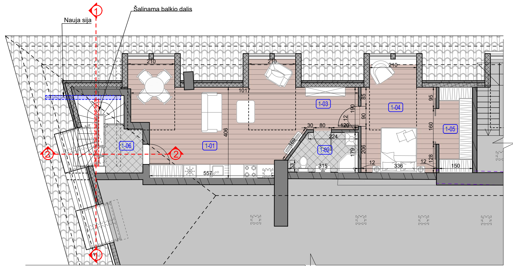
MANSARDINIO AUKŠTO BUTO PLANAS, M 1:100
