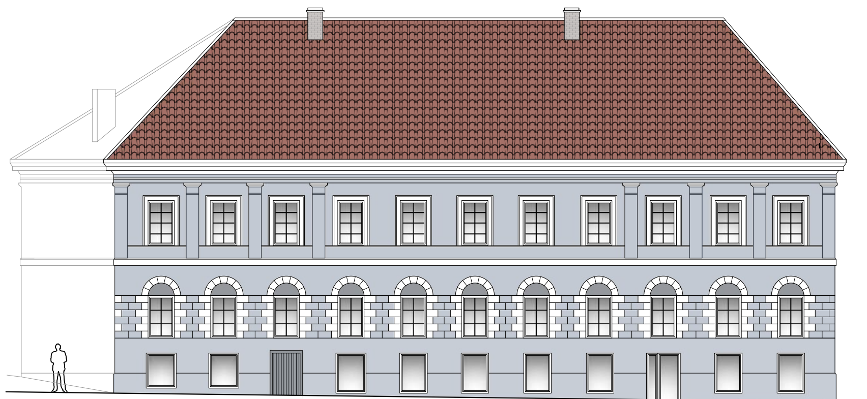
M. DAUKŠOS GATVĖS FASADAS, M 1:150
