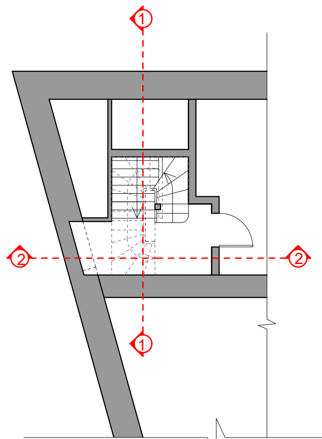
ANTRO AUKŠTO PLANO IŠTRAUKA, M 1:100
