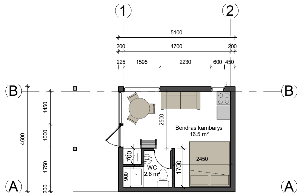
1 Aukšto planas.
