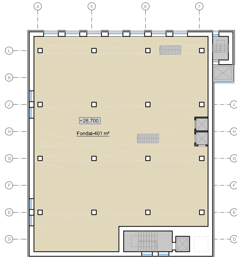
SEPTINTO AUKŠTO PUSAUKŠČIO PLANO SCHEMA
