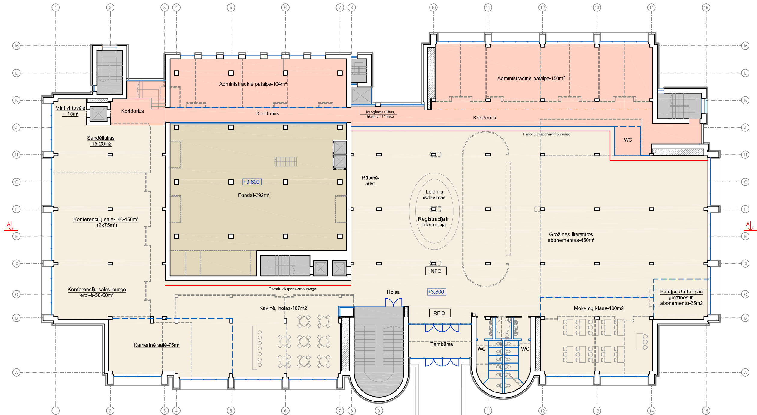
ANTRO AUKŠTO PLANO SCHEMA
