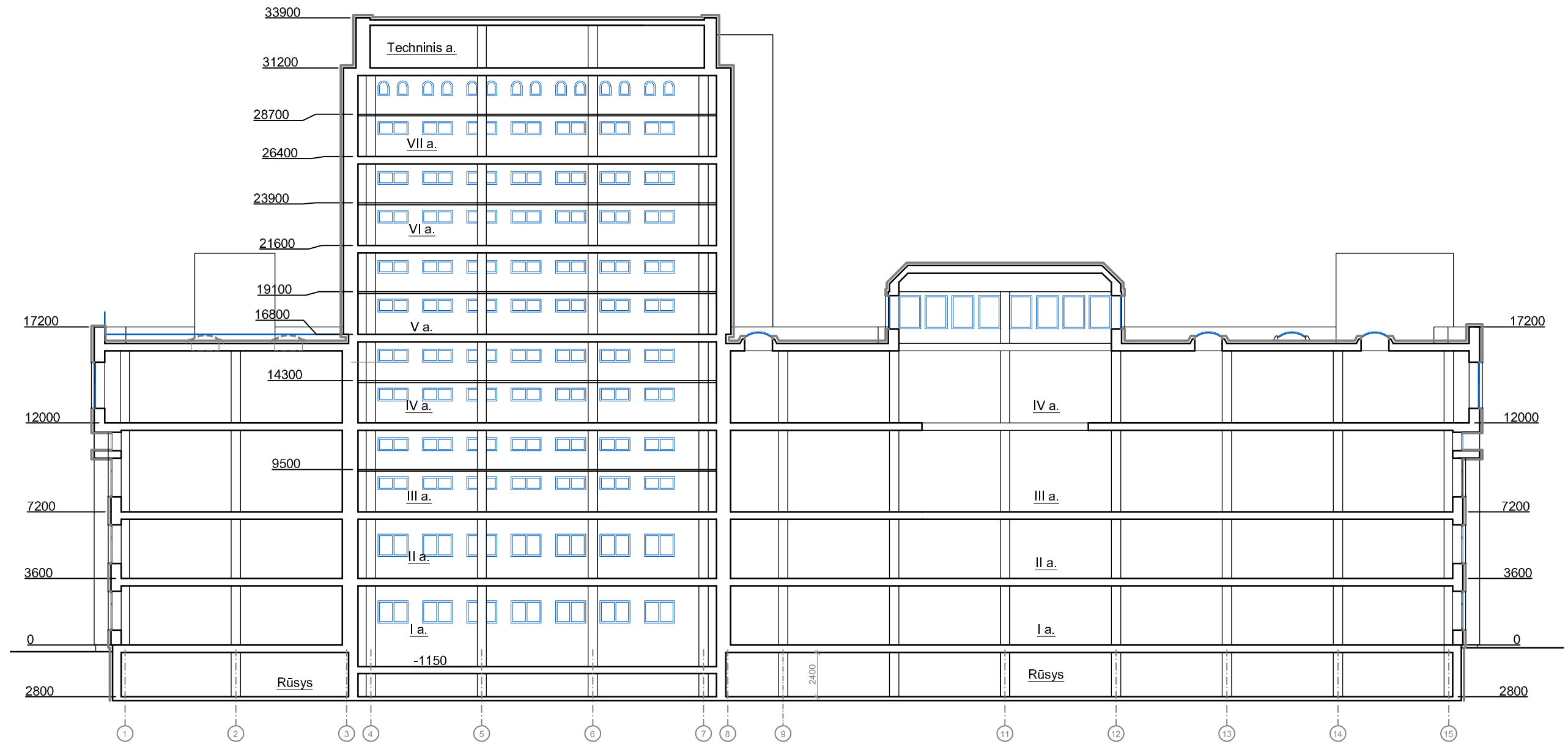
PJŪVIS A-A
