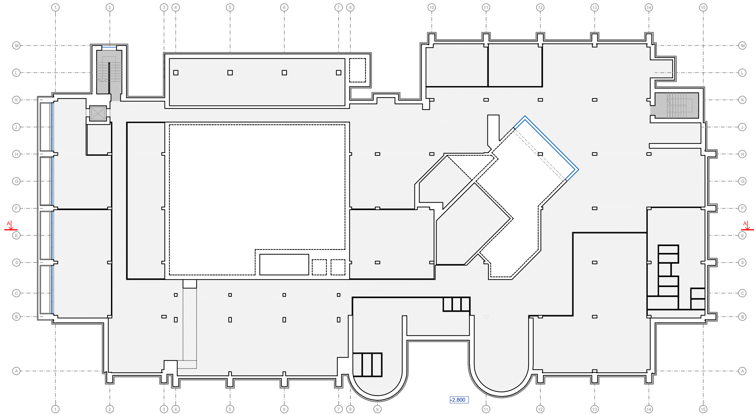
RŪSIO AUKŠTO PLANO SCHEMA
