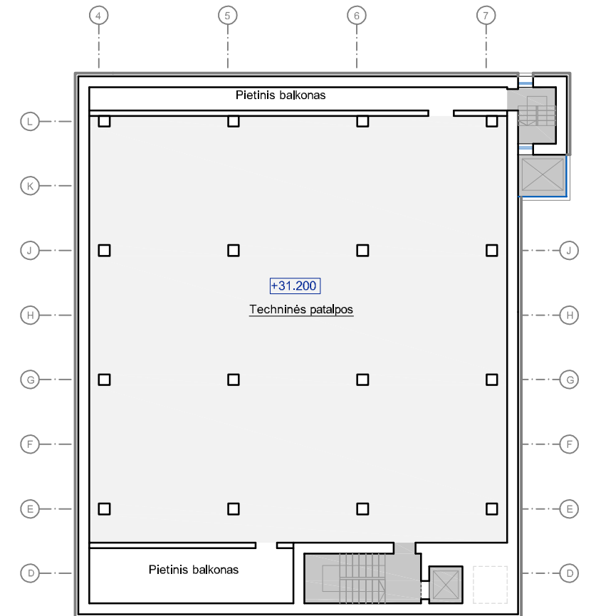
AŠTUNTO AUKŠTO PLANO SCHEMA
