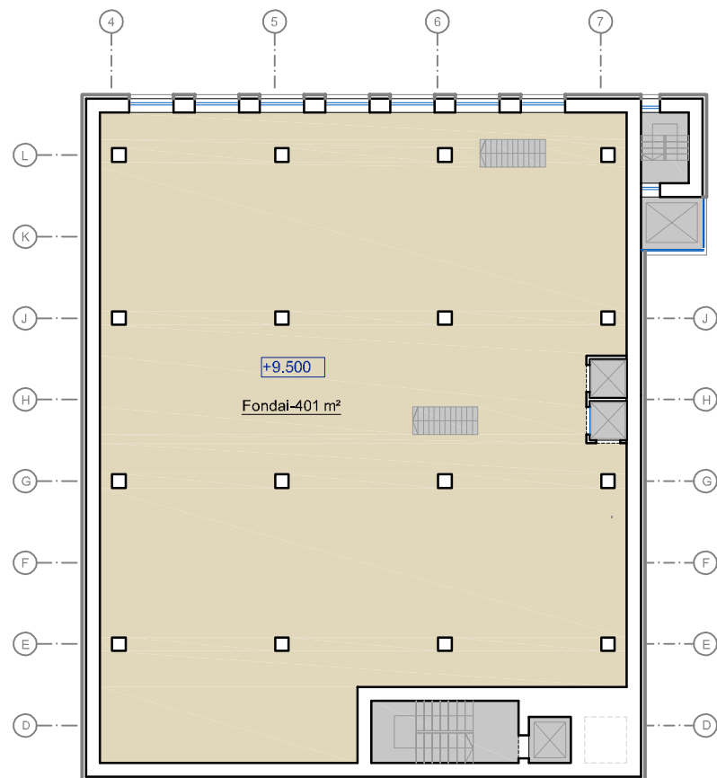
KETVIRTO AUKŠTO PUSAUKŠČIO PLANO SCHEMA
