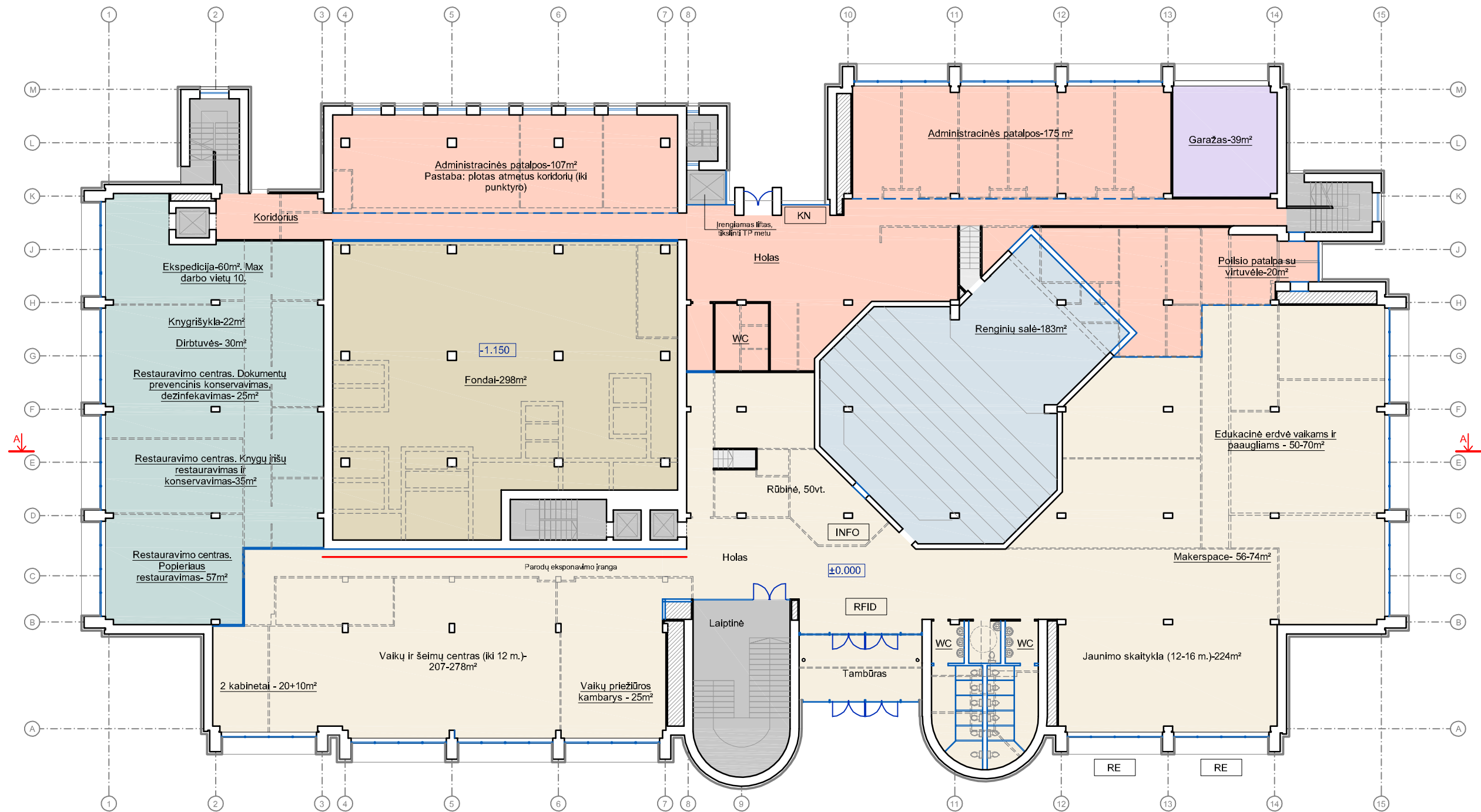
PIRMO AUKŠTO PLANO SCHEMA
