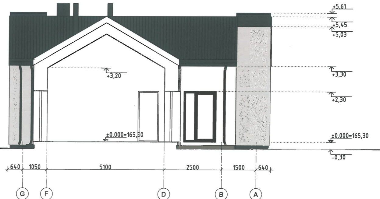
PJŪVIS 4-4
