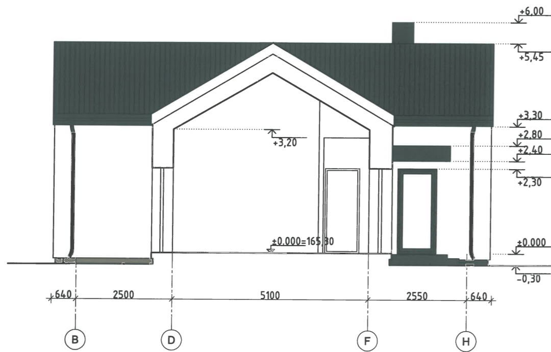
PJŪVIS 3-3
