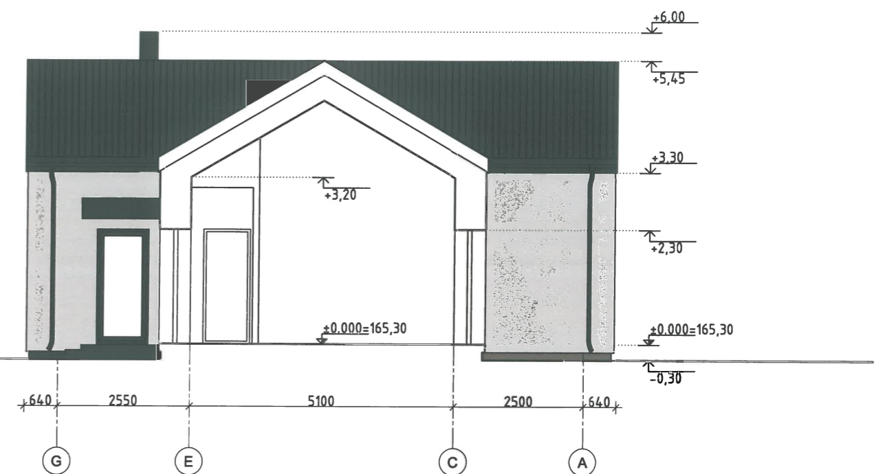
PJŪVIS 2-2
