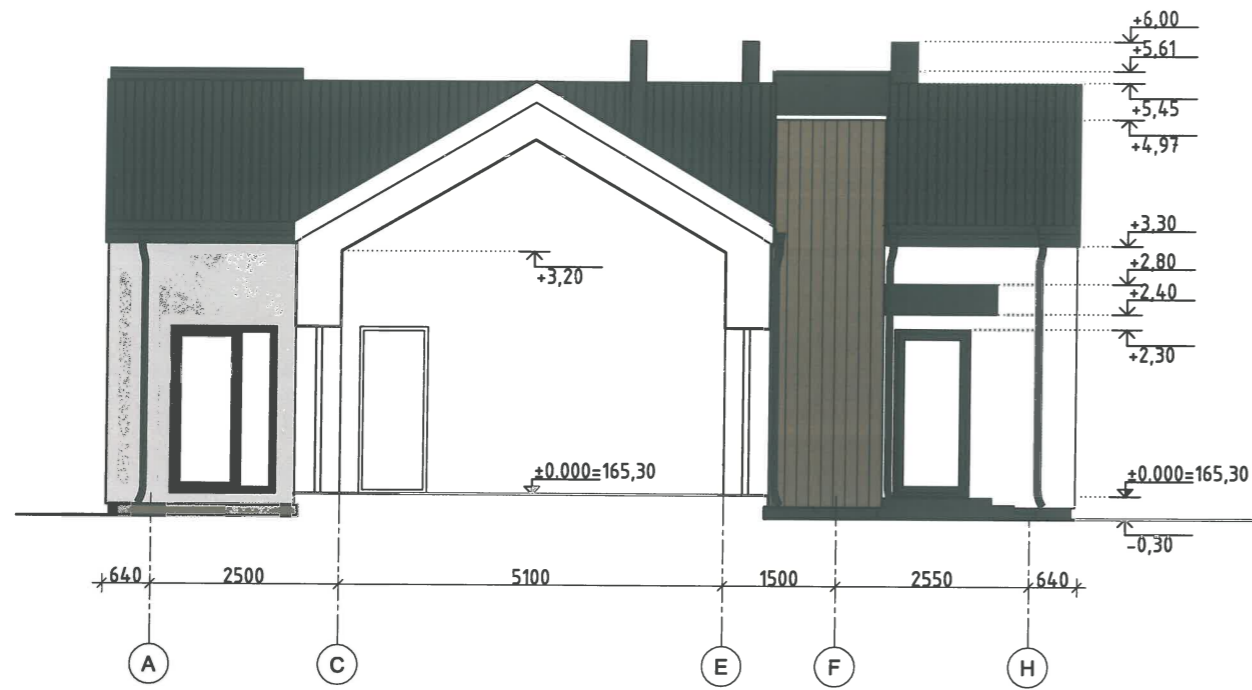
PJŪVIS 1-1
