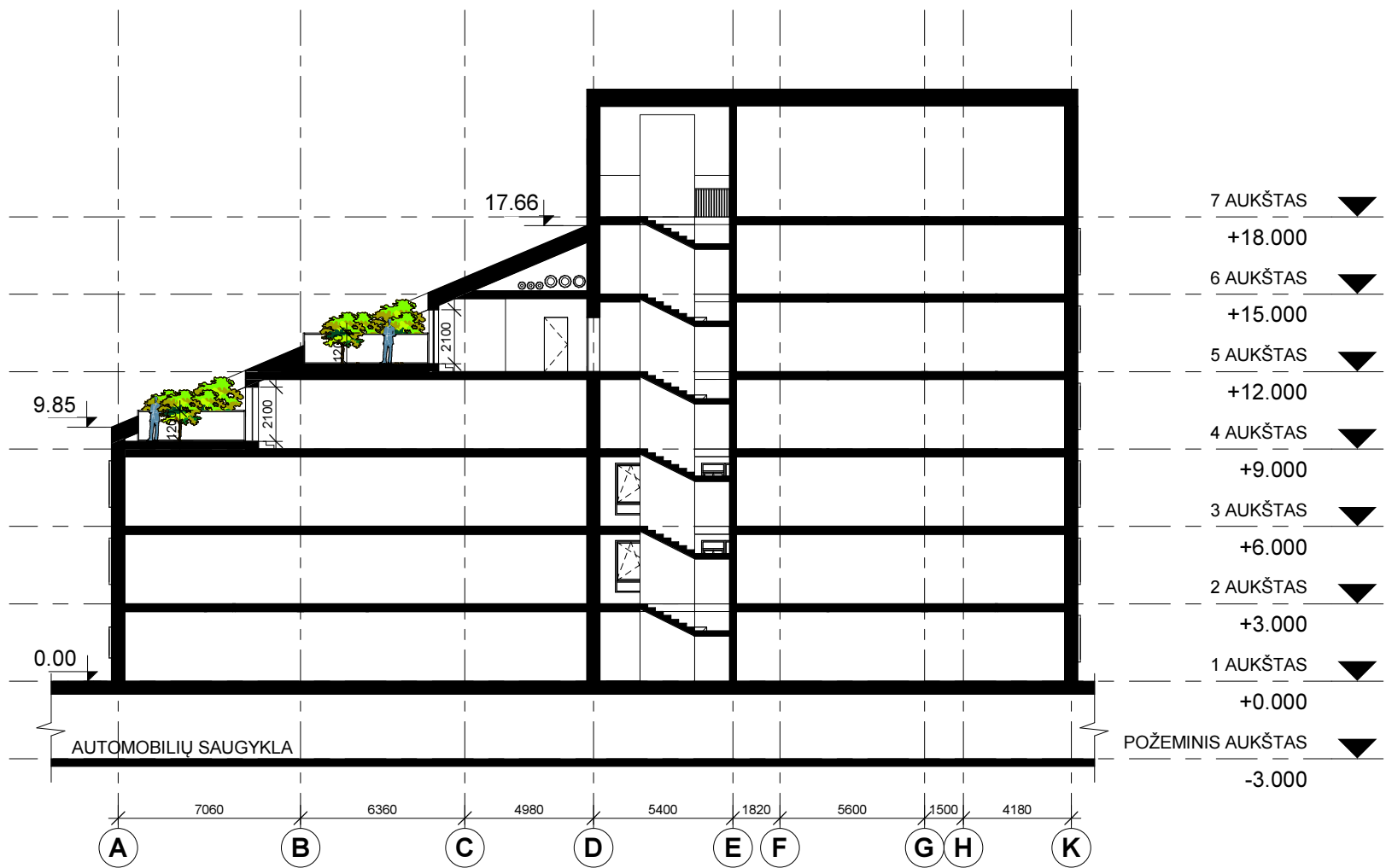
PJŪVIS 1-1 1 : 250
