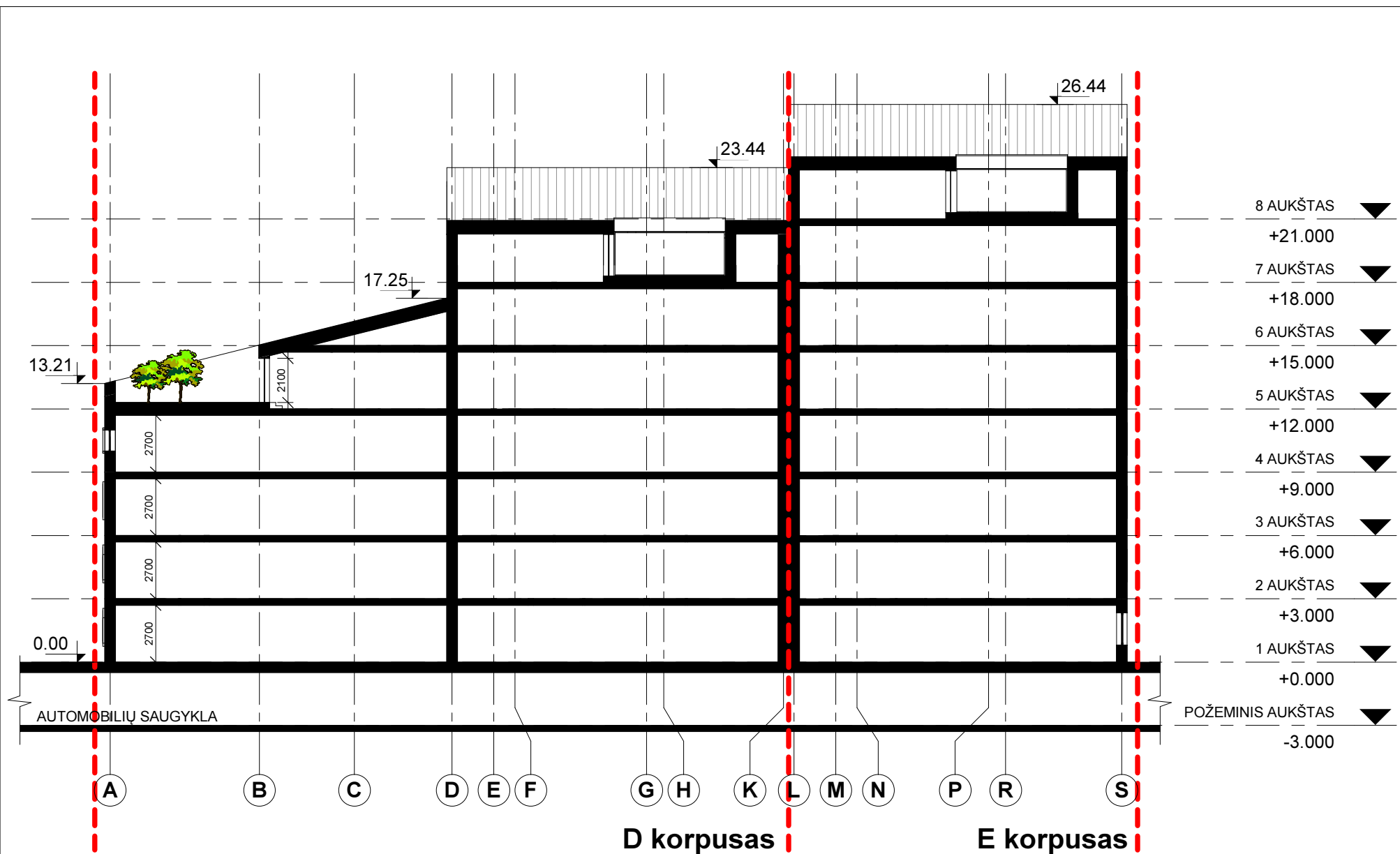
PJŪVIS 1-1 1 : 250
