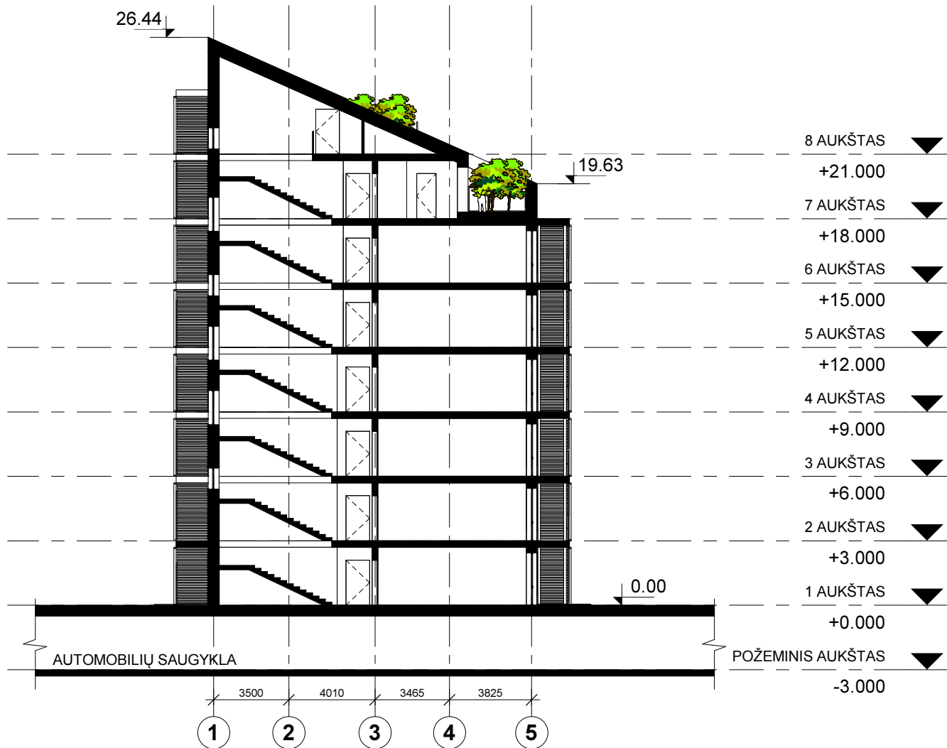
PJŪVIS 2-2 1 : 250
