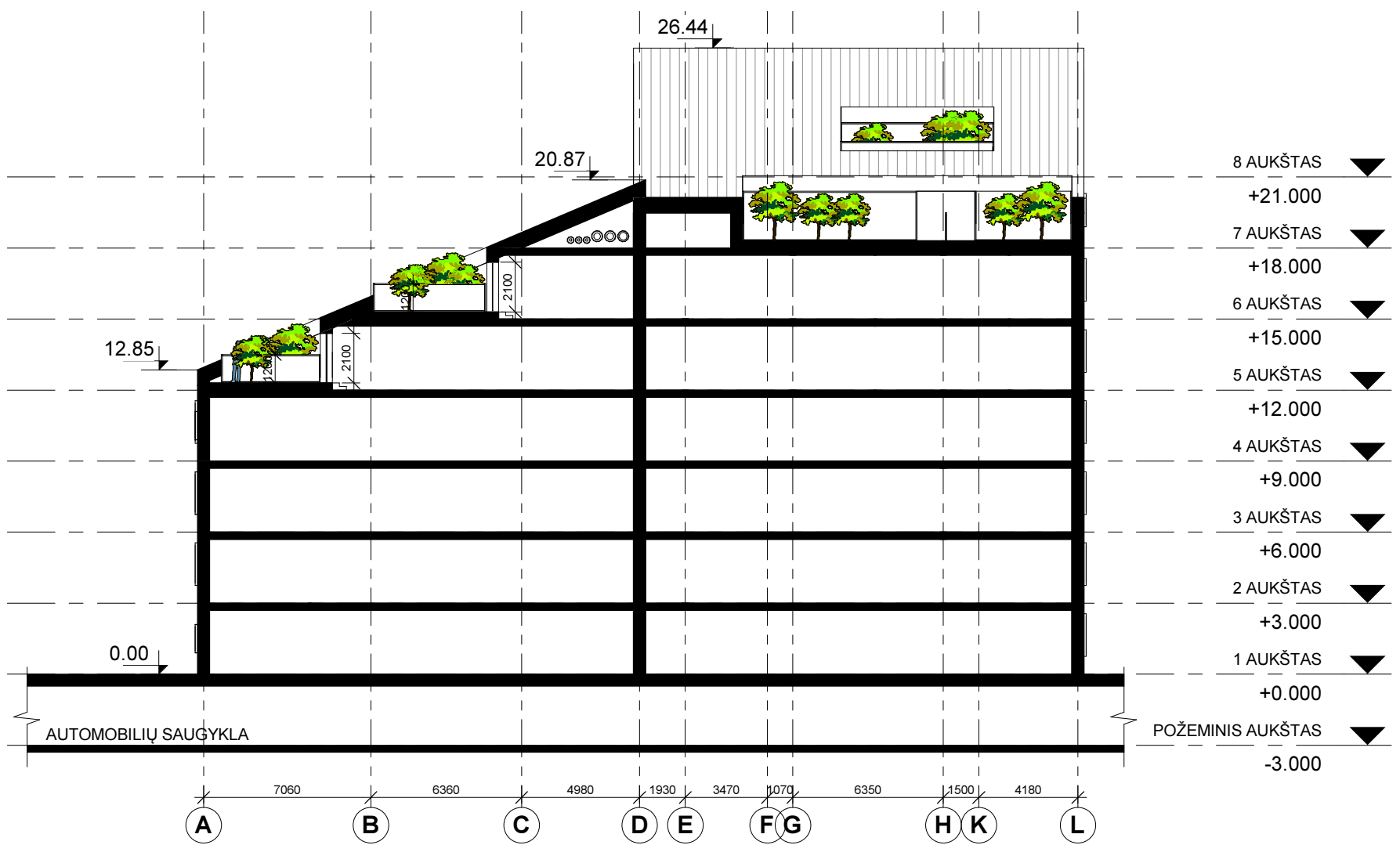
PJŪVIS 1-1 1 : 250
