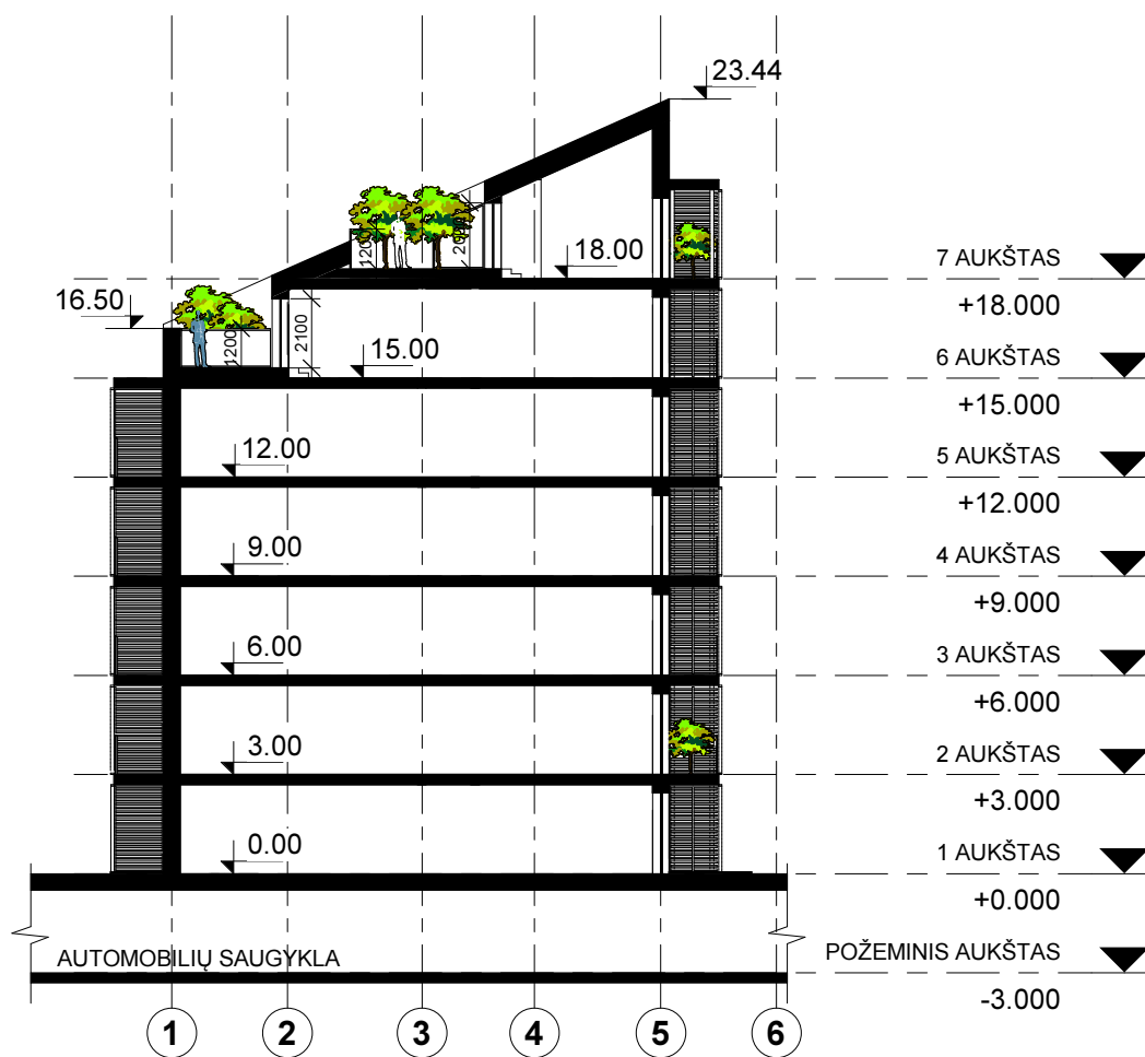
PJŪVIS 2-2 1 : 250
