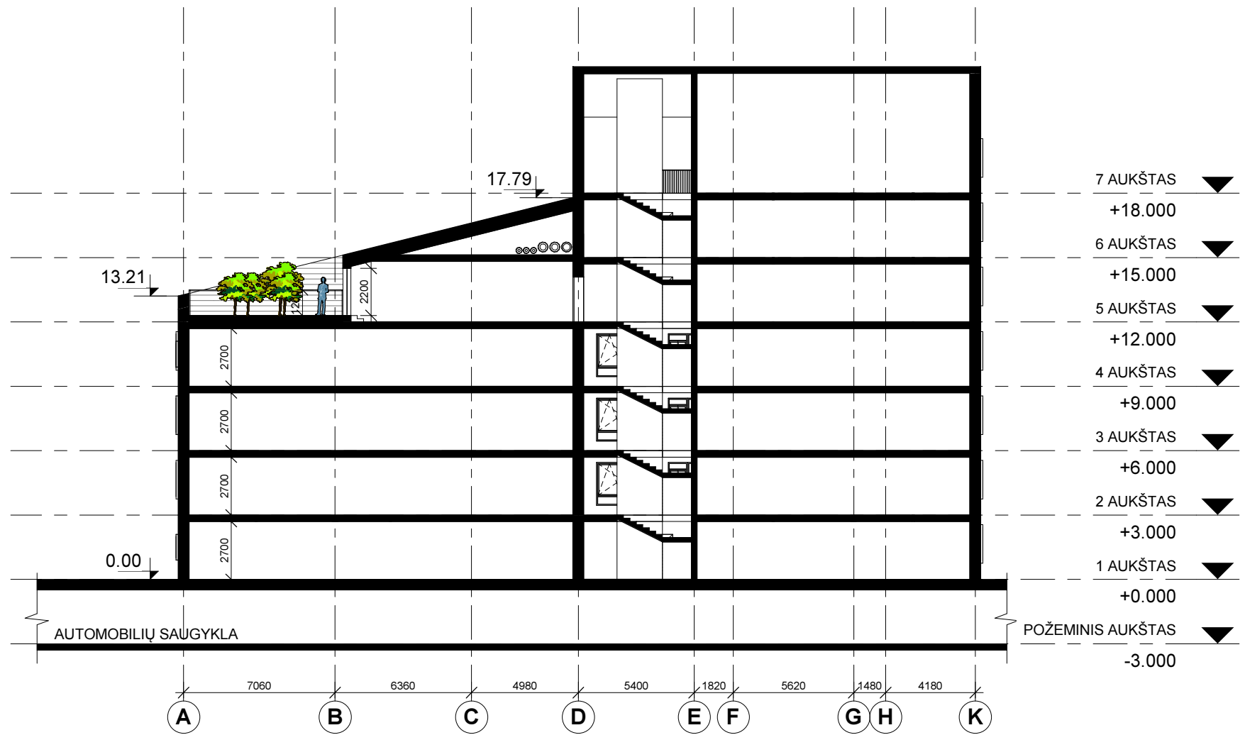
PJŪVIS 1-1 1 : 250
