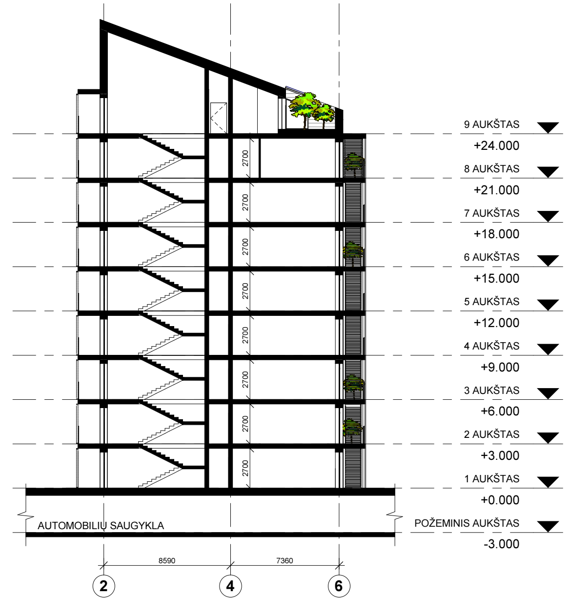
PJŪVIS 2-2 1 : 250
