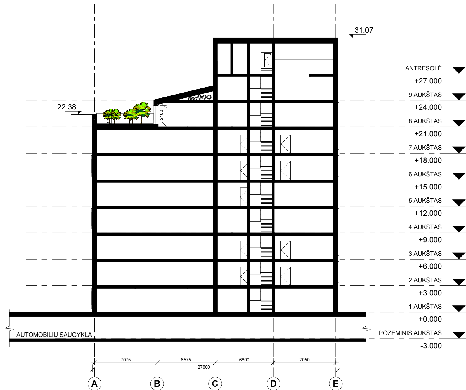
PJŪVIS 1-1 1 : 250
