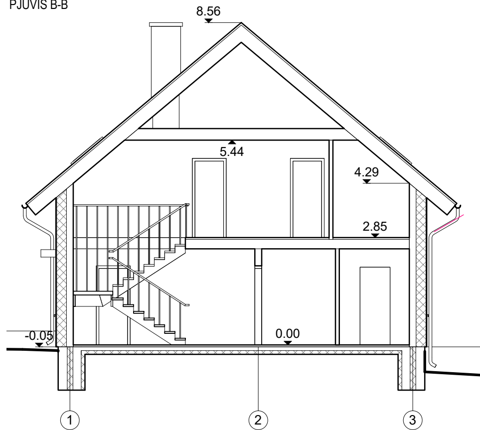
PJŪVIS B-B
