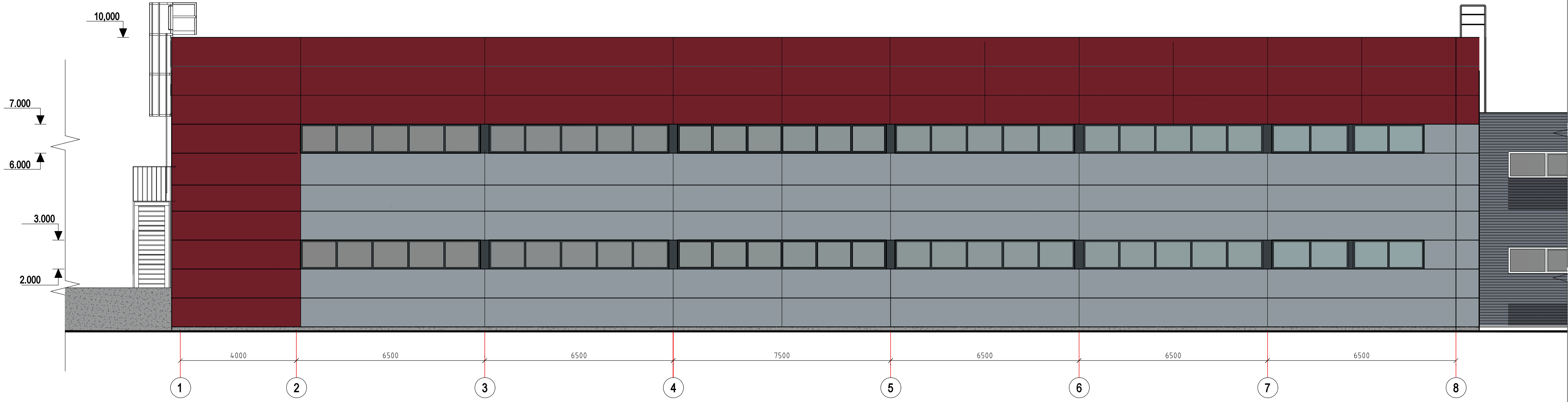
Fasadas 1-8 M1:100
