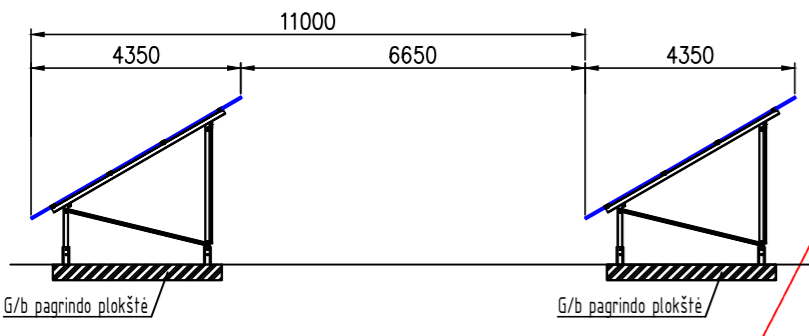
Saulės modulių tipinė pastatymo schema
