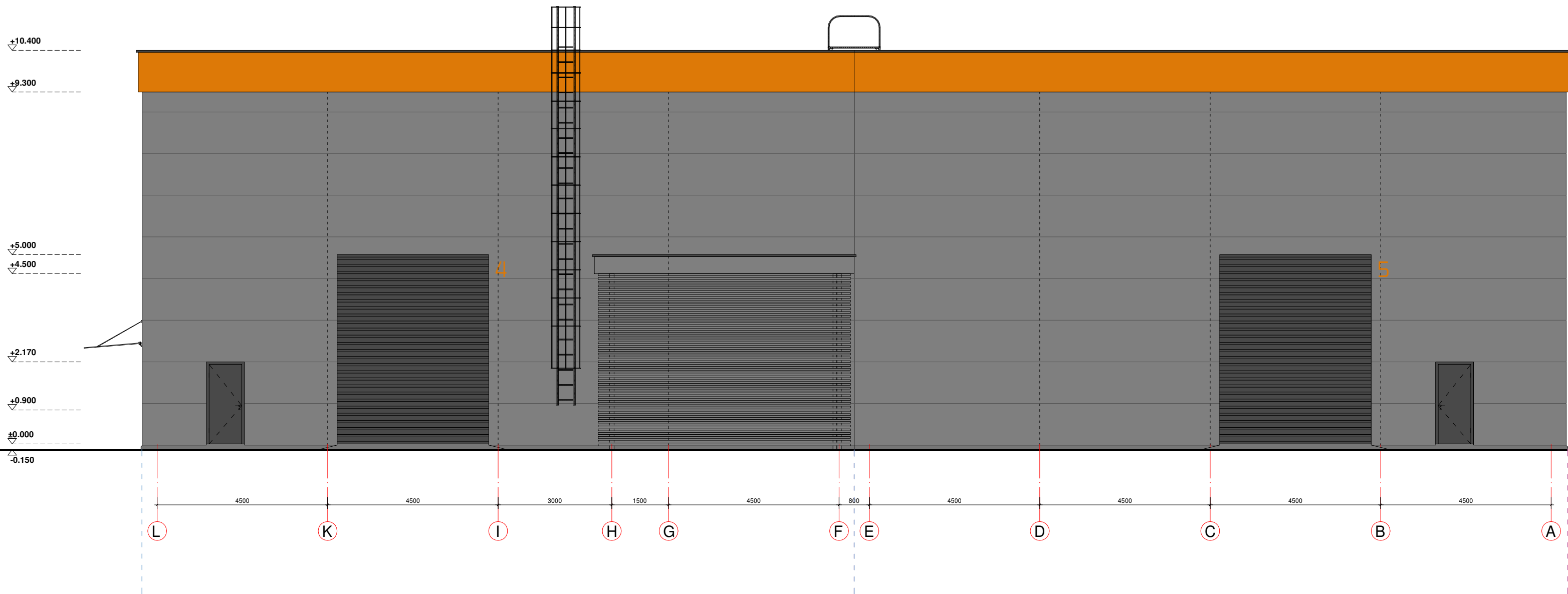
I ETAPAS TARP AŠIŲ L-F/1-11
