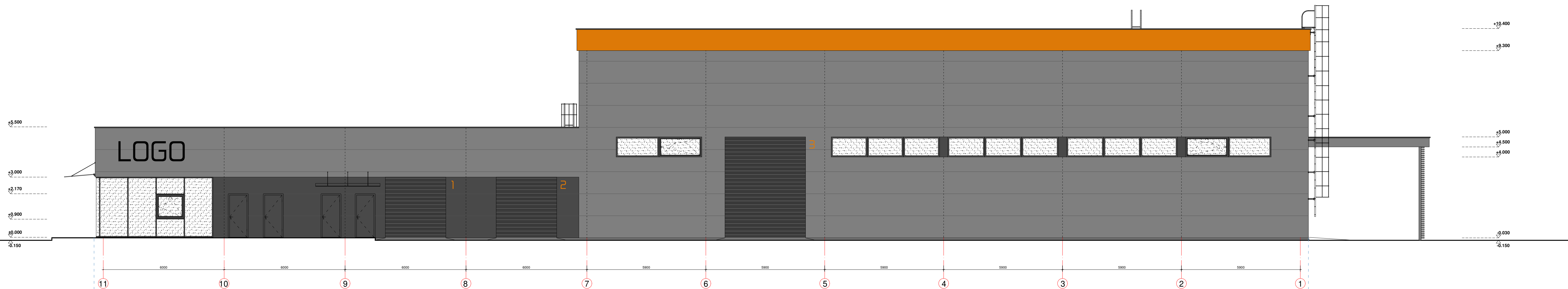
ŠIAURĒS FASADAS 11-1 M1:100
