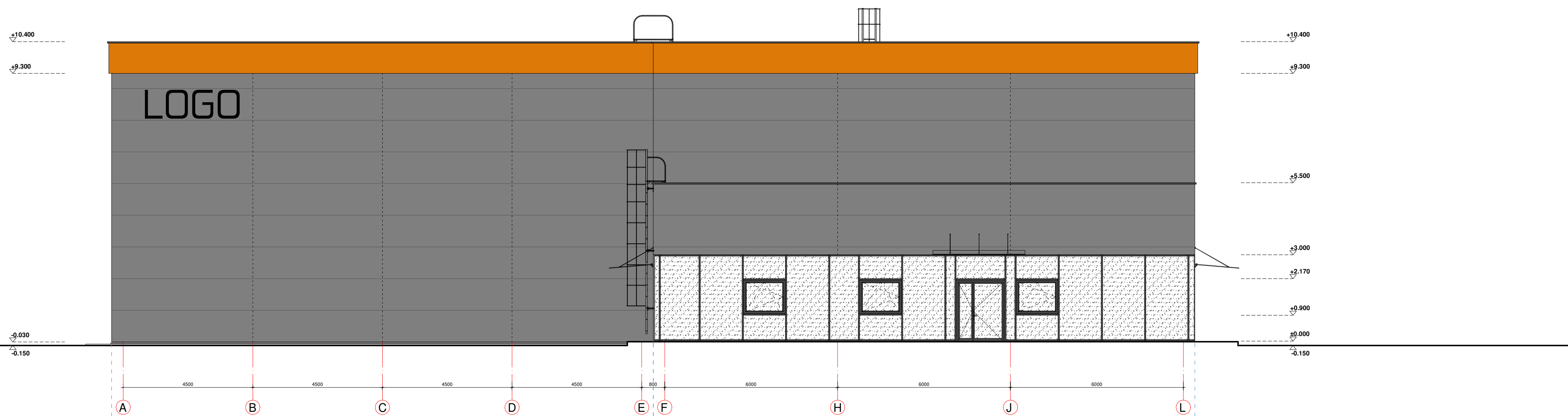
RYTŲ FASADAS A-L M1:100
