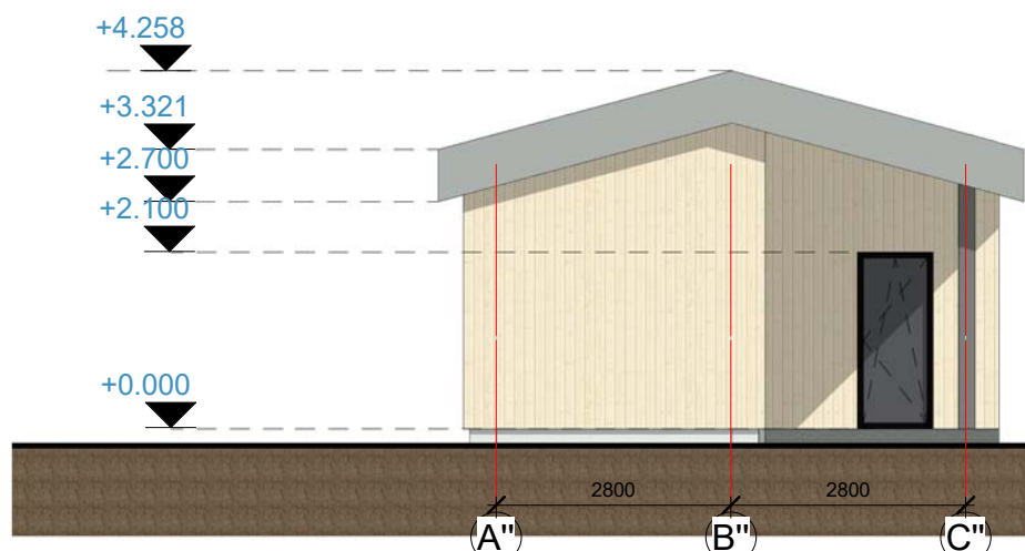
PIETINIS FASADAS M 1:100
