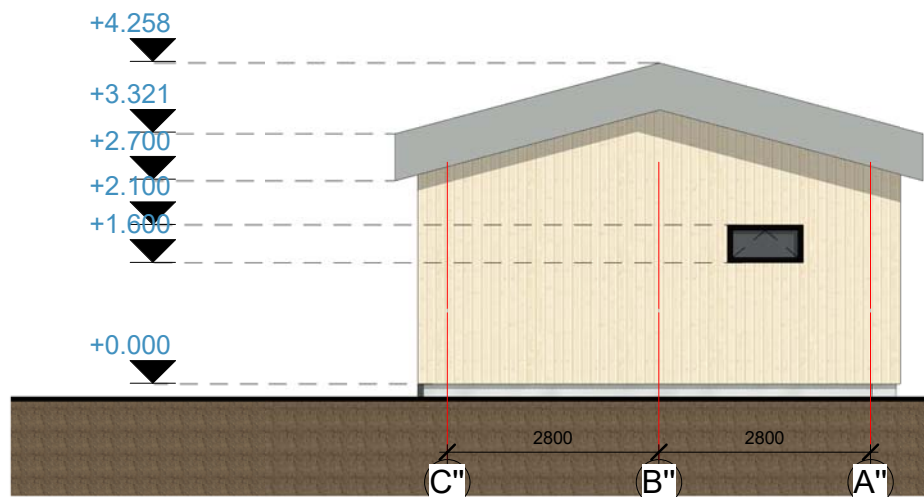
ŠIAURINIS FASADAS M 1:100
