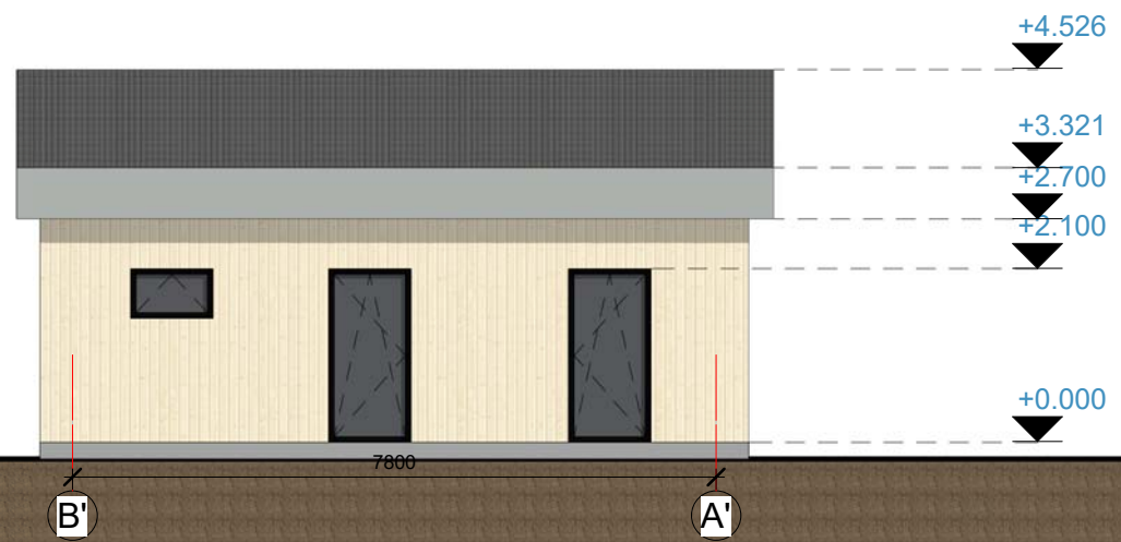
VAKARINIS FASADAS M 1:100
