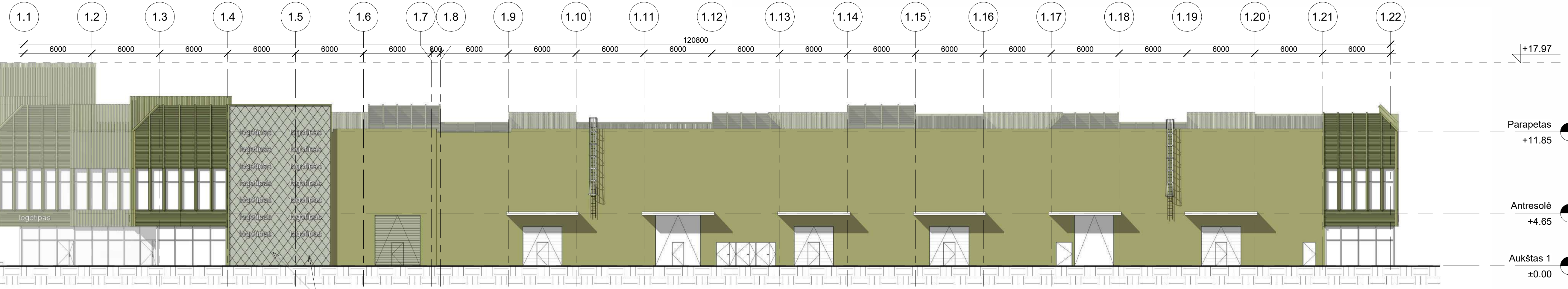
3 Pietryčių fasadas 1 : 200
