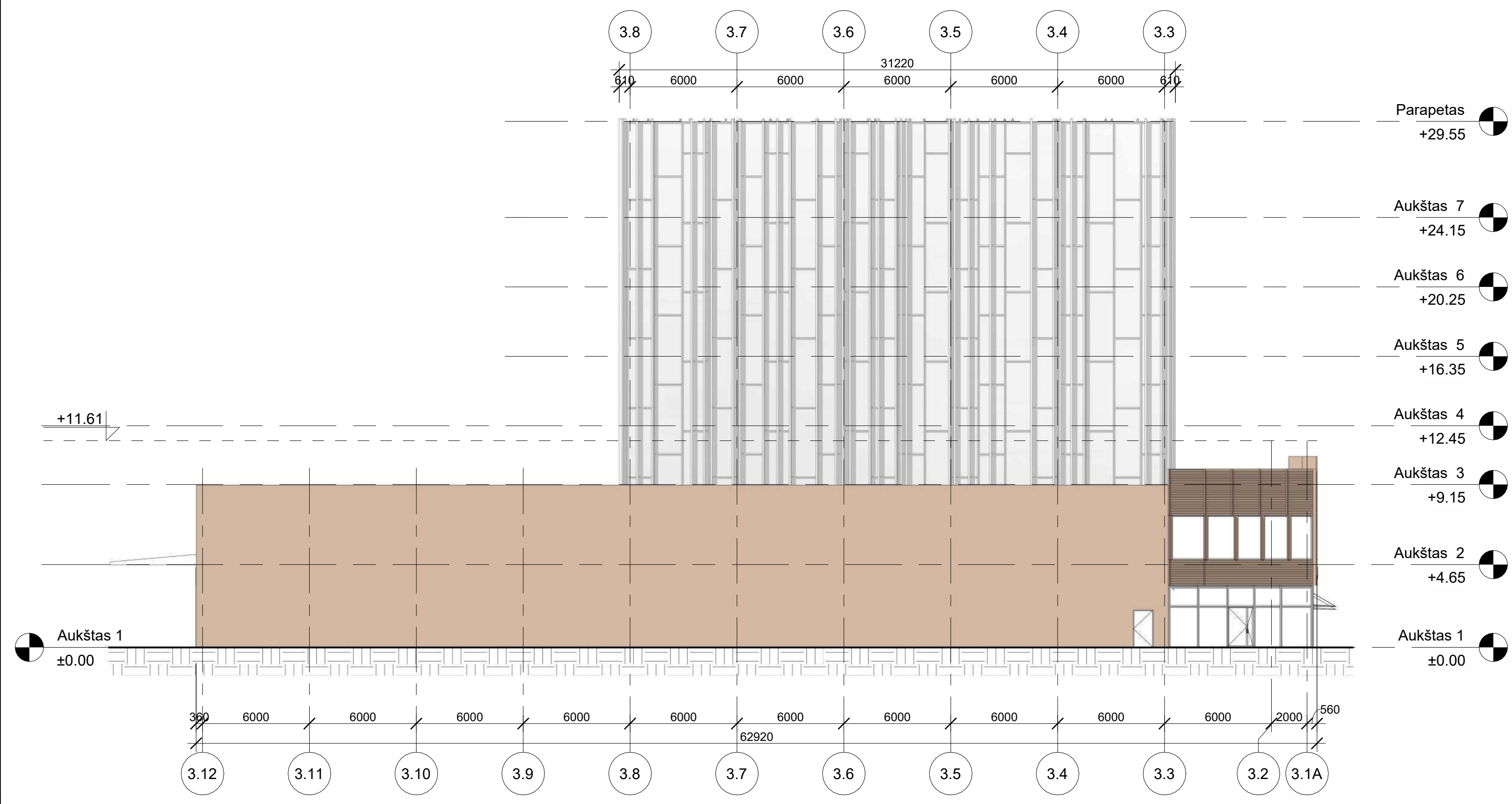
3 Šiaurės-vakarų fasadas 1:200
