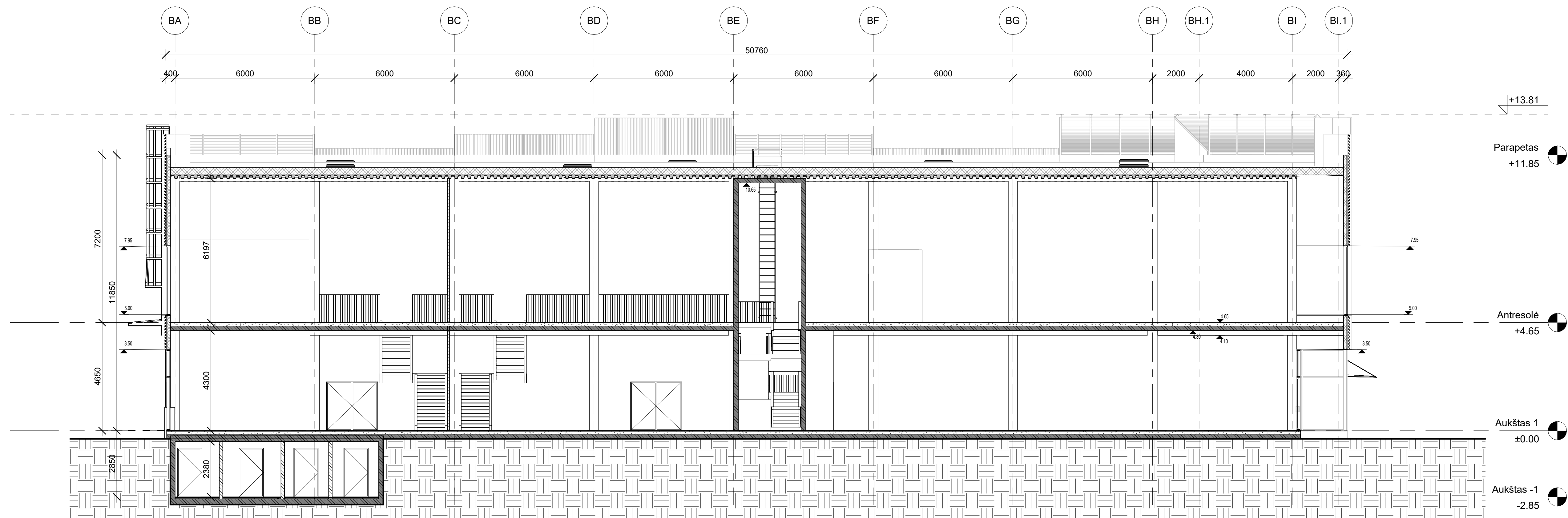
1 | Pastatas 2B - Pjūvis 1-1 1 : 100
