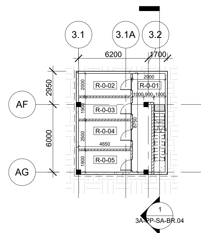
1 Pastatas 3A - Pirmo aukšto planas
