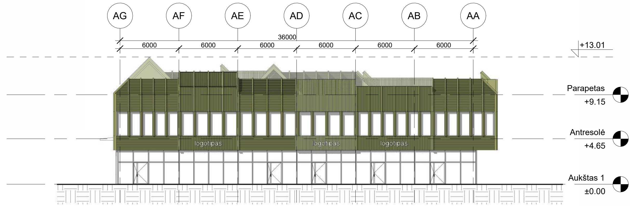
2 Šiaurės-rytų fasadas 1 : 200
