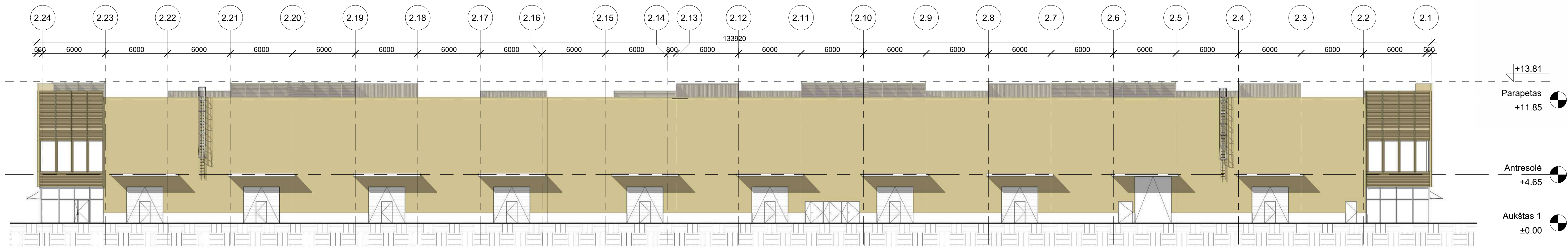
1 | Šiaurės-vakarų fasadas 1 : 200
