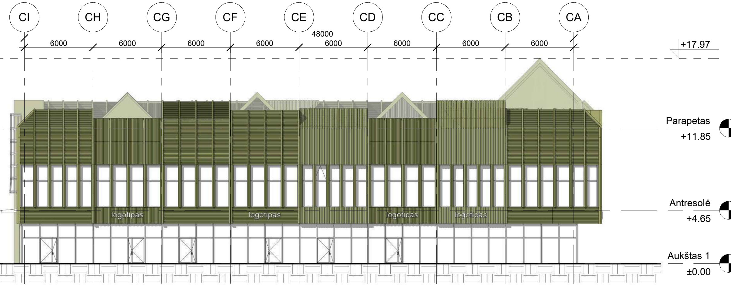
2 Šiaurės-rytų fasadas 1 : 200
