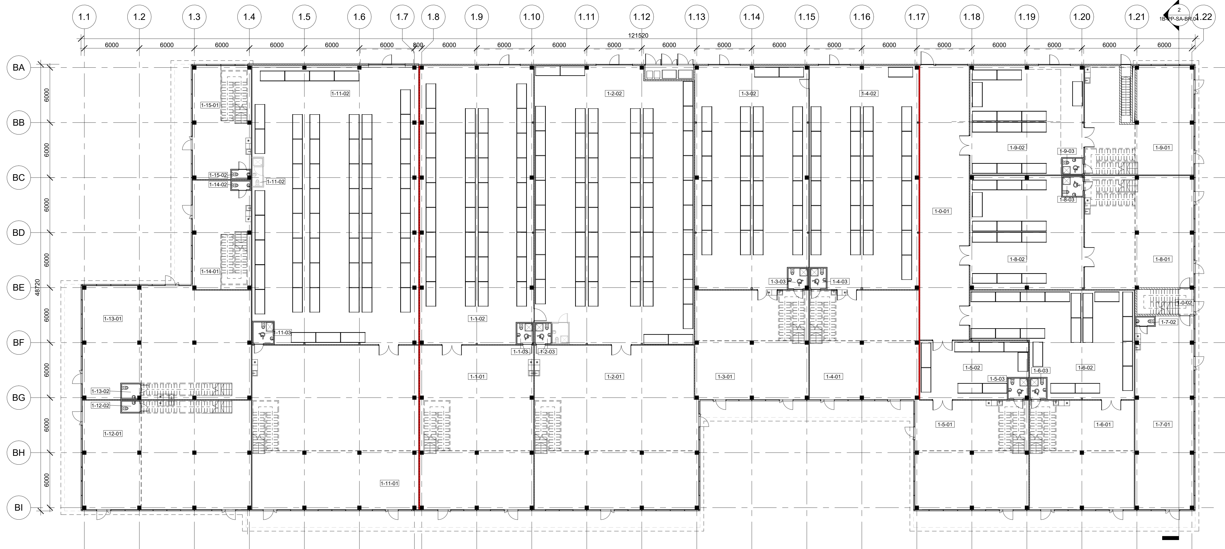
1 Pastatas 1B - Pirmo aukšto planas 1 : 200
