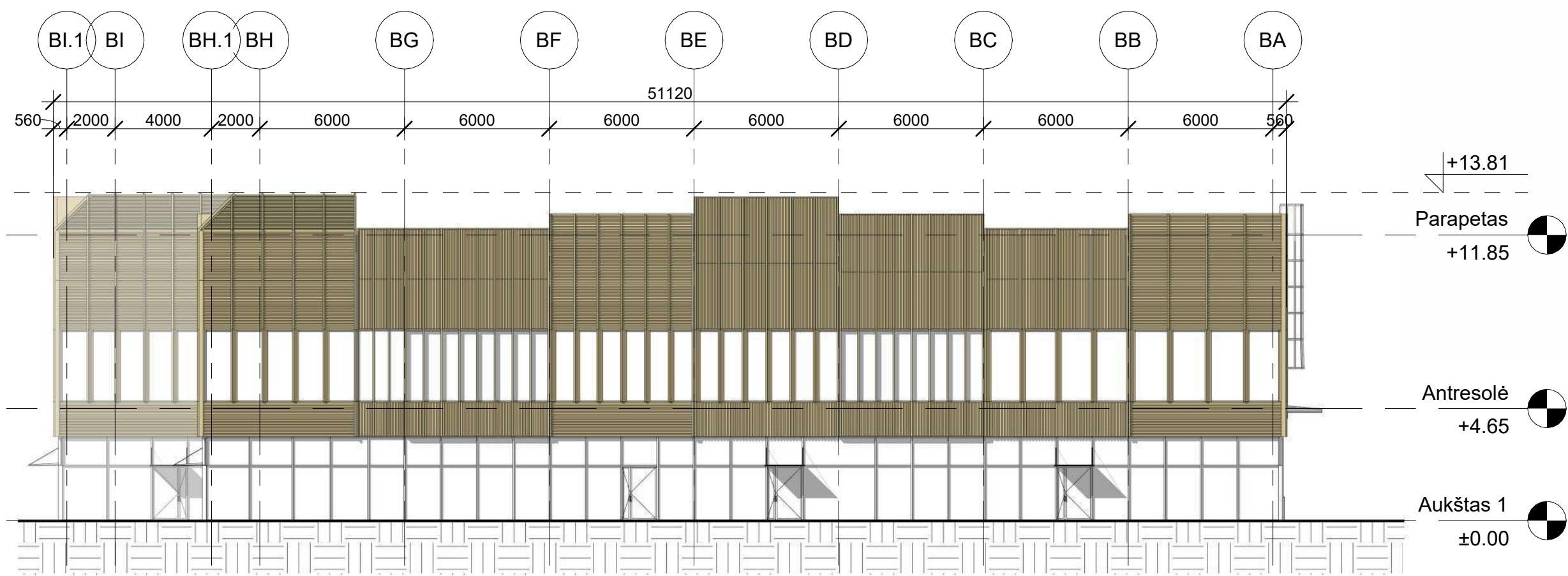
2 | Šiaurės-rytų fasadas 1 : 200
