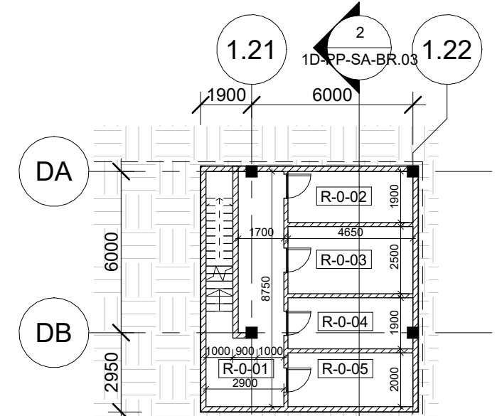
Pastatas 1D - Rūsio planas 1 : 200
