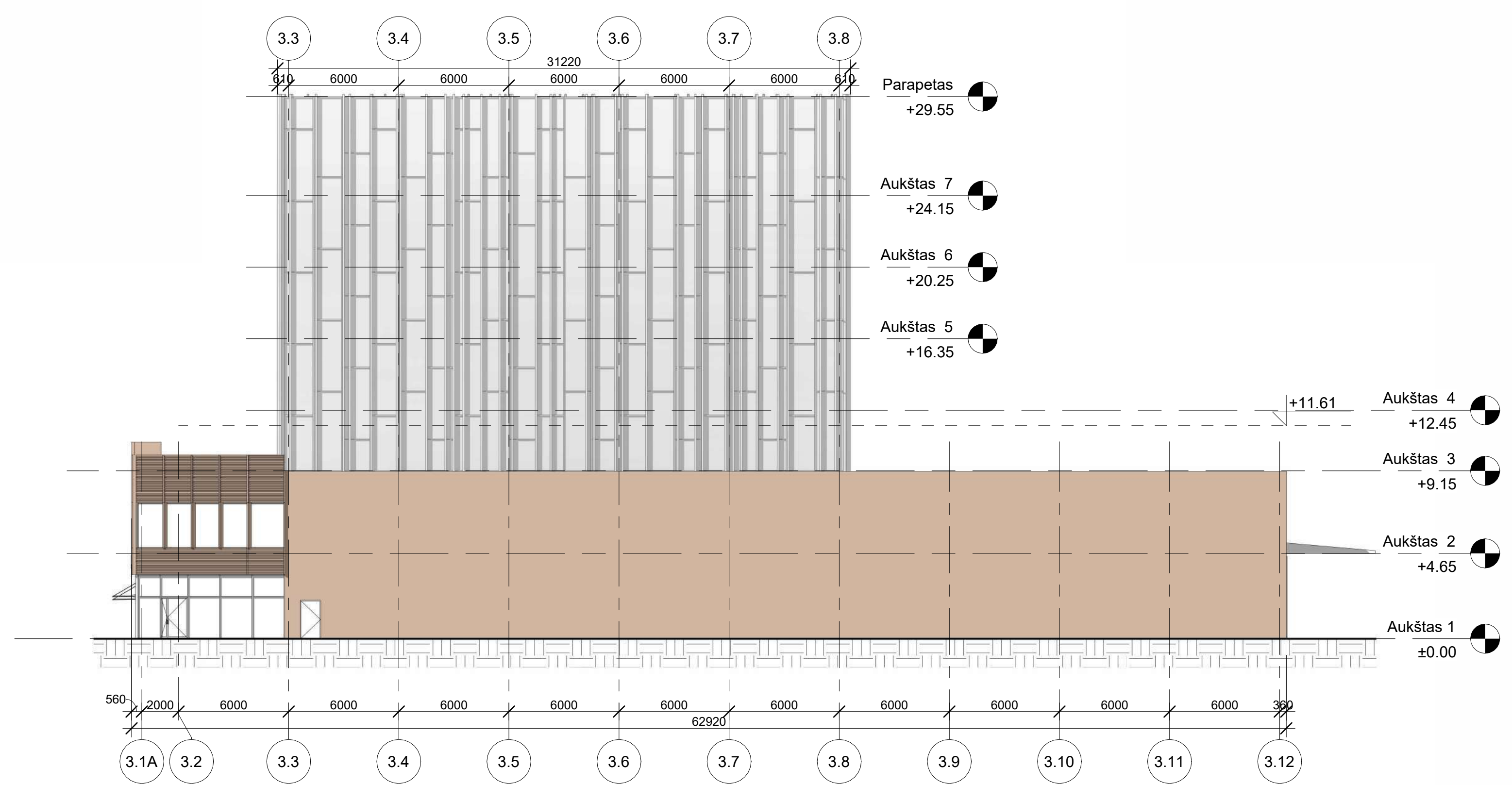
3 | Pastatas 3B - Pietryčių fasadas 1 : 200
