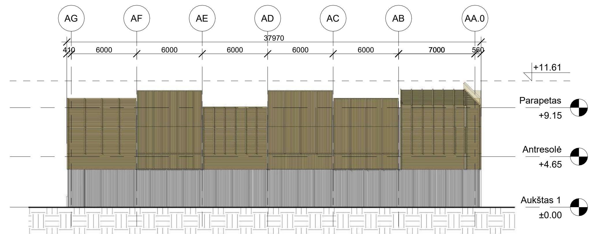
2 | Šiaurės-rytų fasadas 1 : 200
