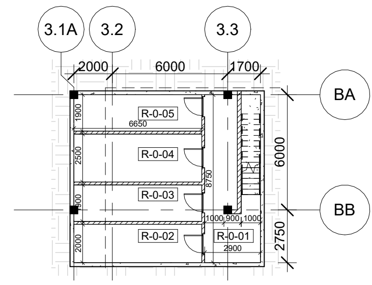
R | Pastatas 3B - Rūsio planas 1 : 200
