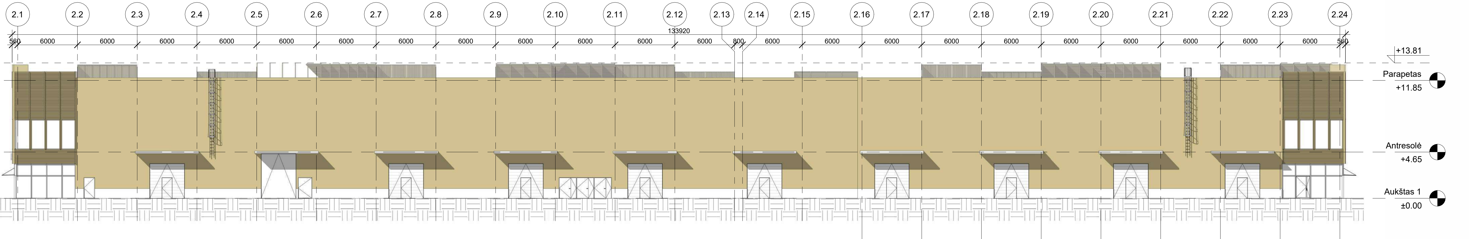
2 Šiaurės-rytų fasadas 1 : 200
