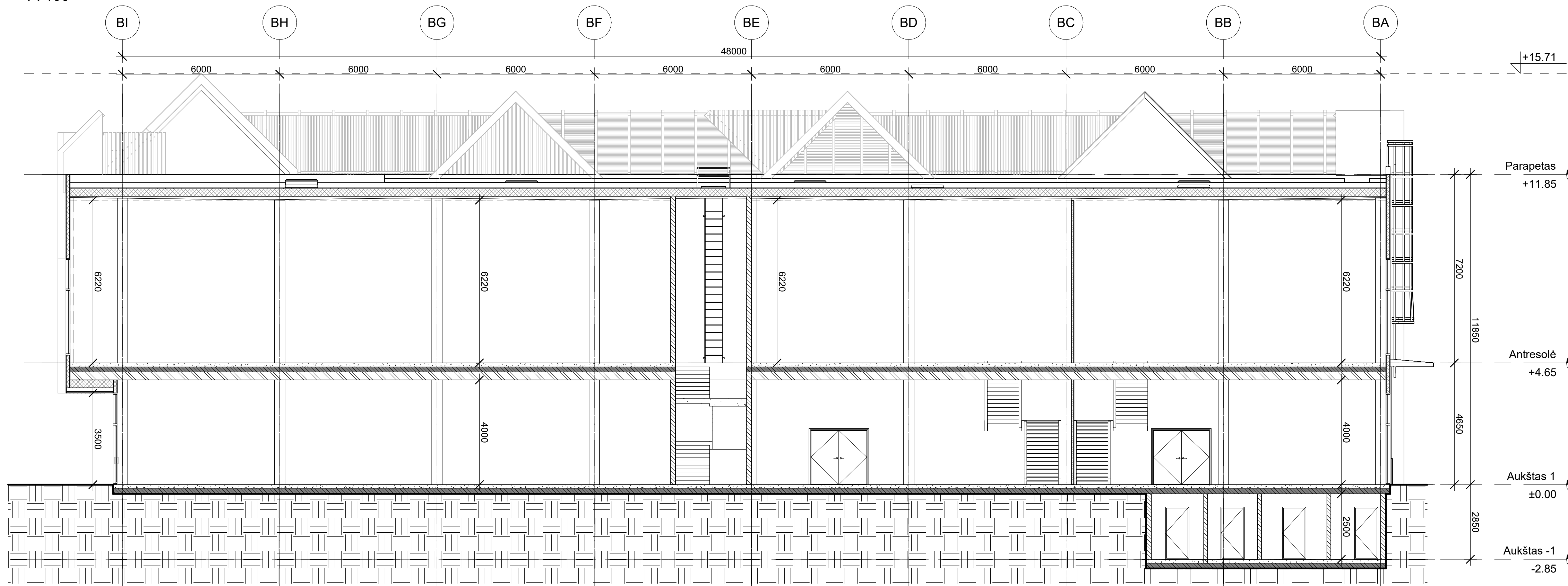
2 Pastatas 1B - Pjūvis 2-2 1 : 100
