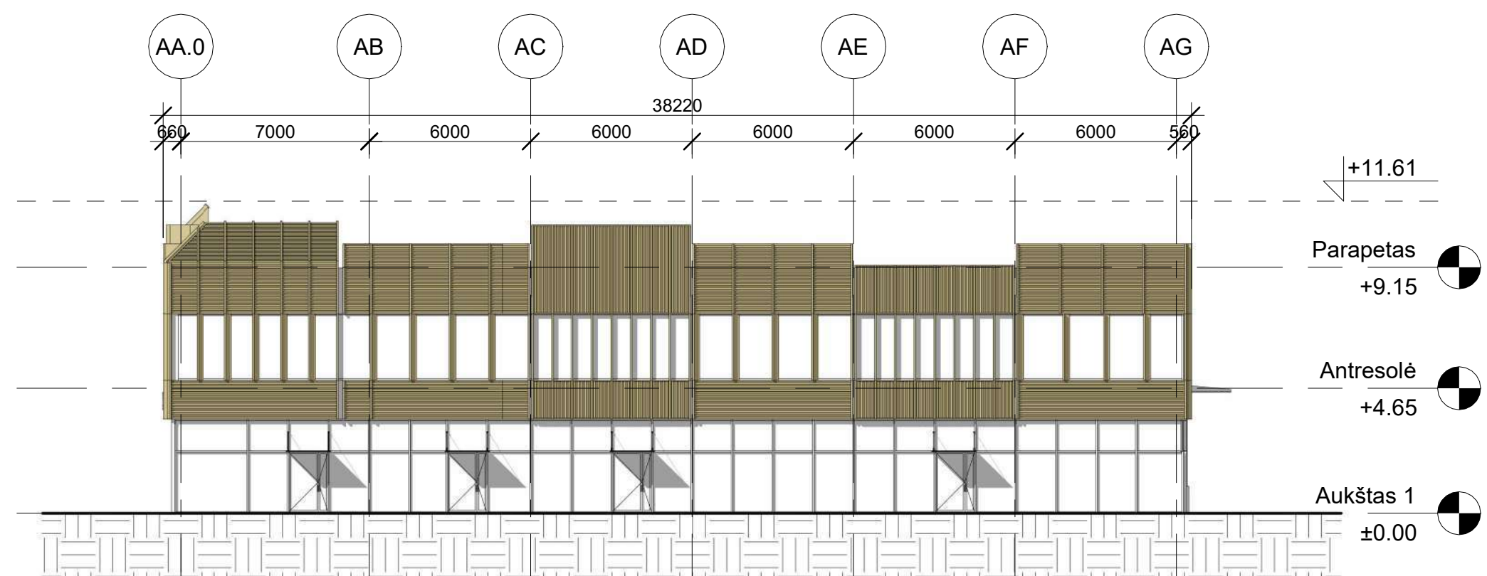
4 | Pietvakarių fasadas 1 : 200
