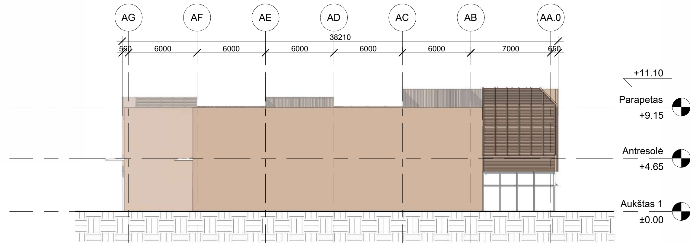
1 | Šiaurės-vakarų fasadas 1 : 200
