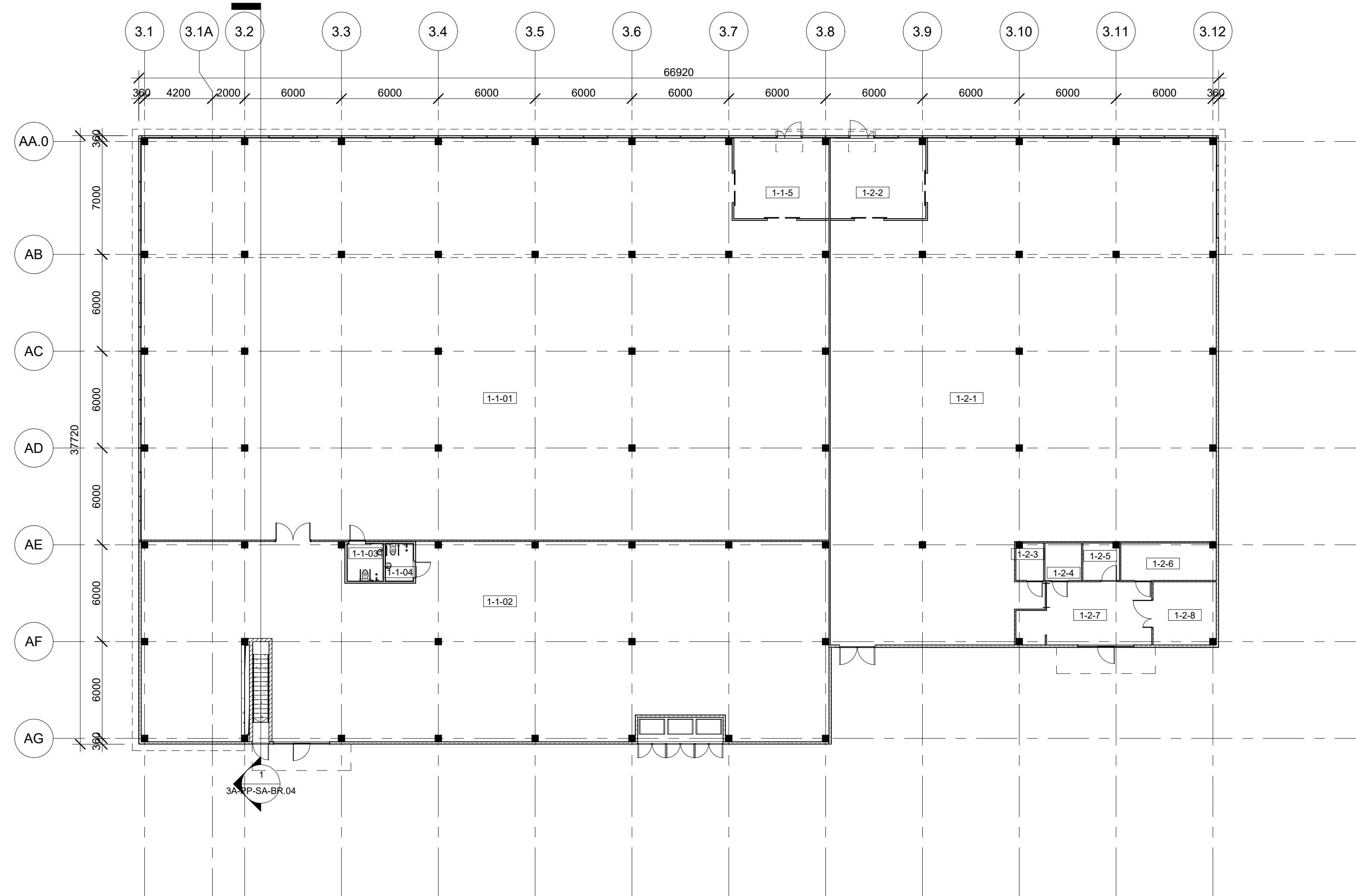
1 Pastatas 3A - Pirmo aukšto planas
