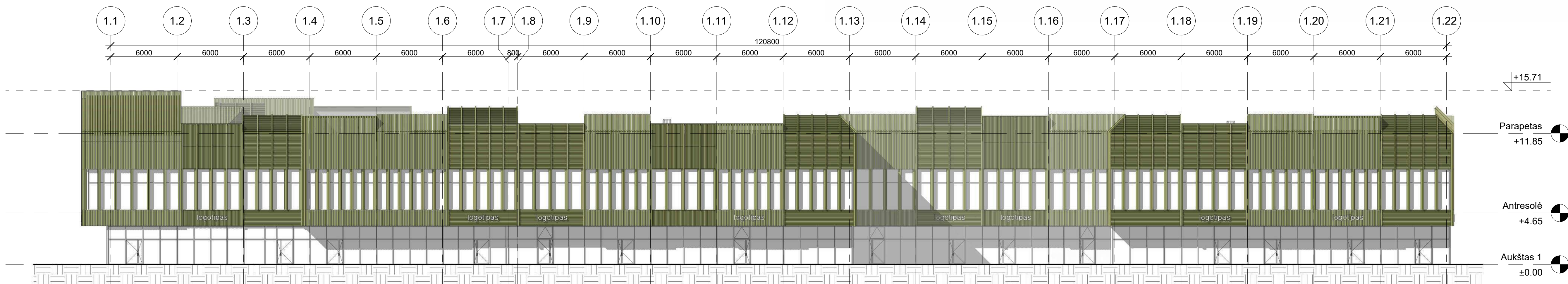
3 Pietryčių fasadas 1 : 200
