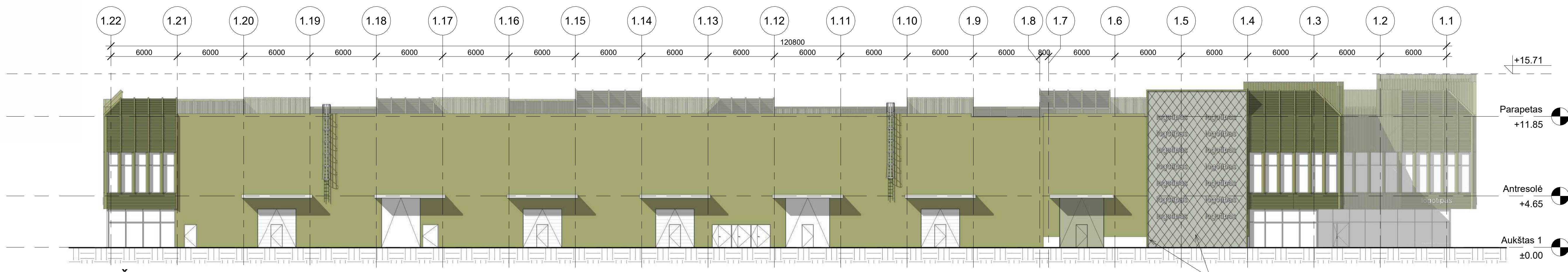
1 Šiaurės-vakarų fasadas 1 : 200
