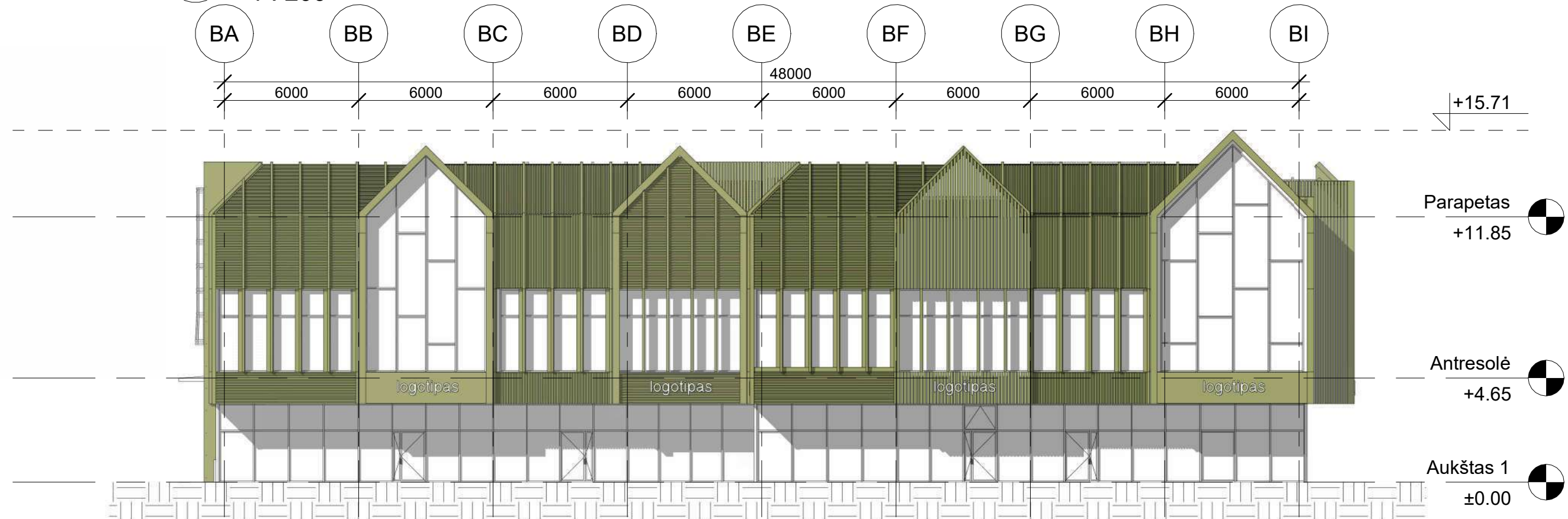
4 Pietvakarių fasadas 1 : 200
