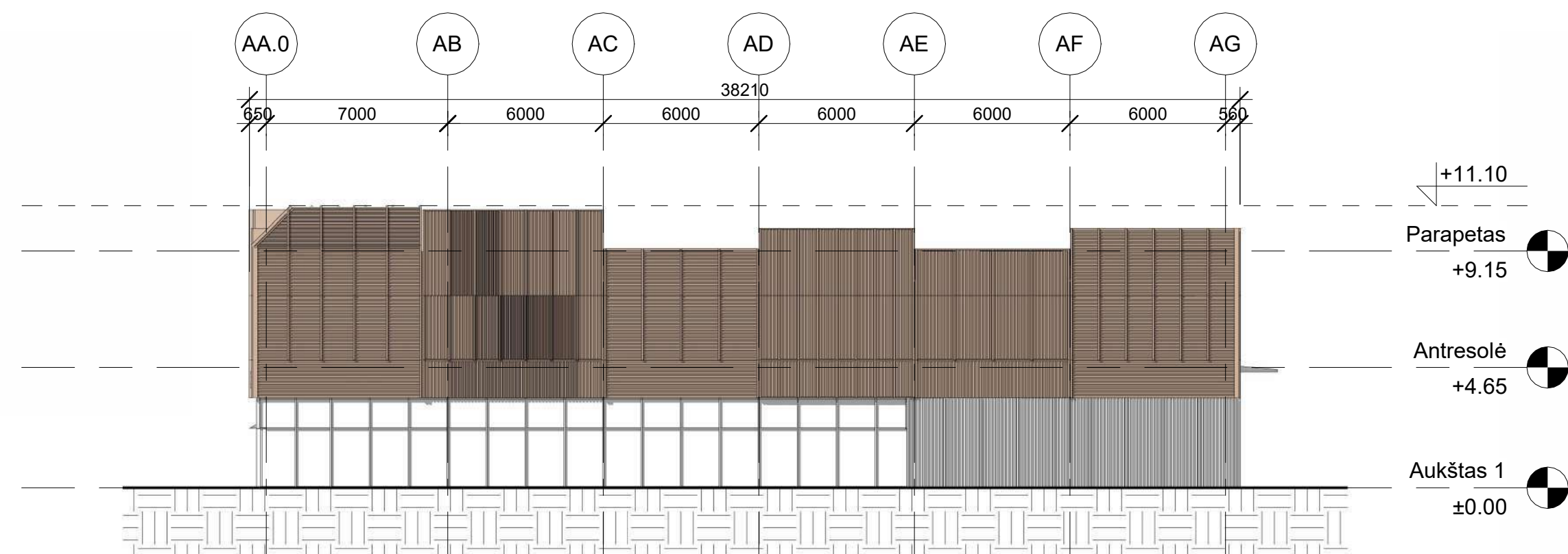
4 | Pietvakarių fasadas 1 : 200
