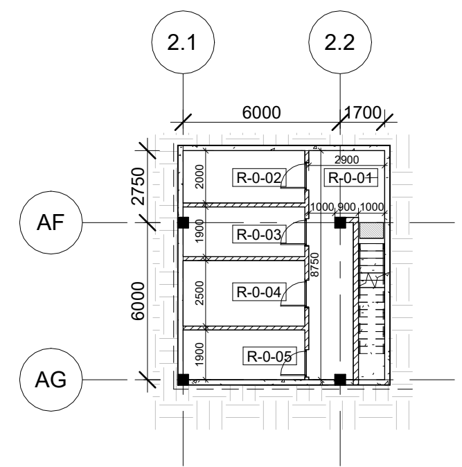
R1 | Pastatas 2A - Rūšio planas 1 : 200
