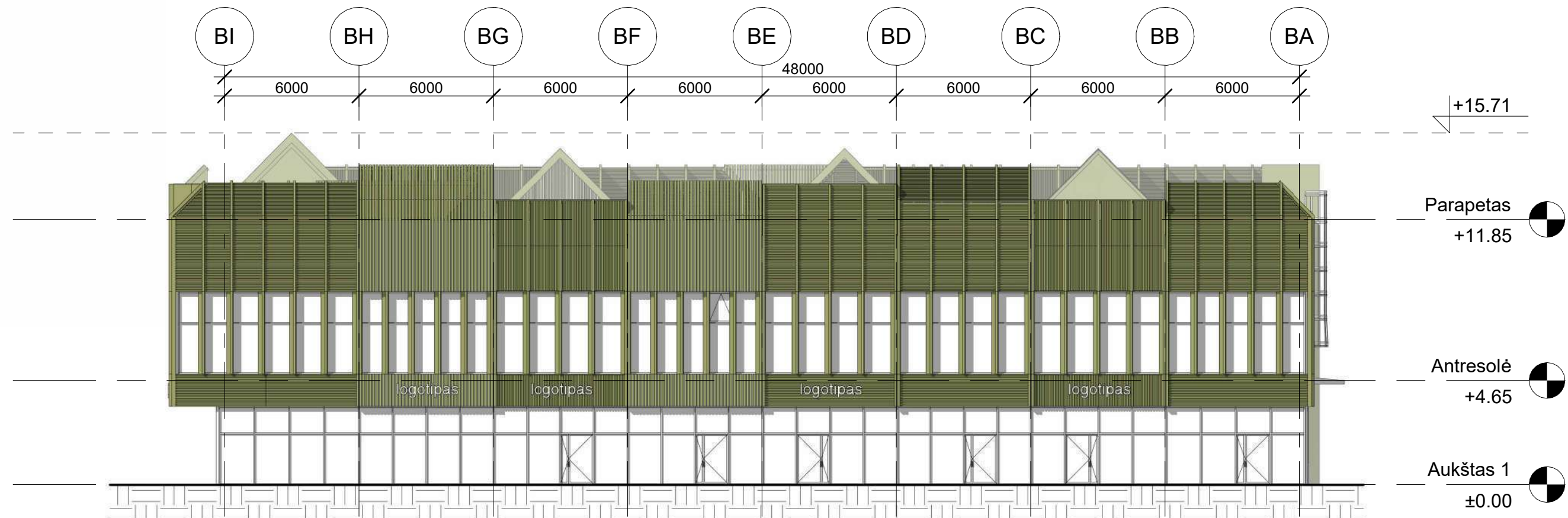
2 Šiaurės-rytų fasadas 1 : 200
