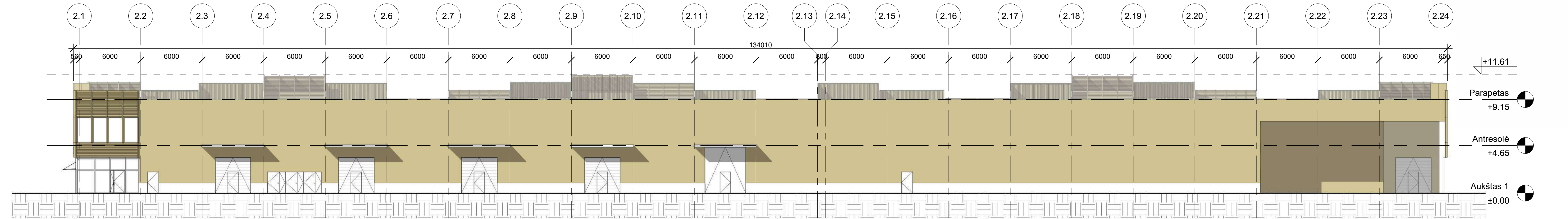
3 | Pietryčių fasadas 1 : 200
