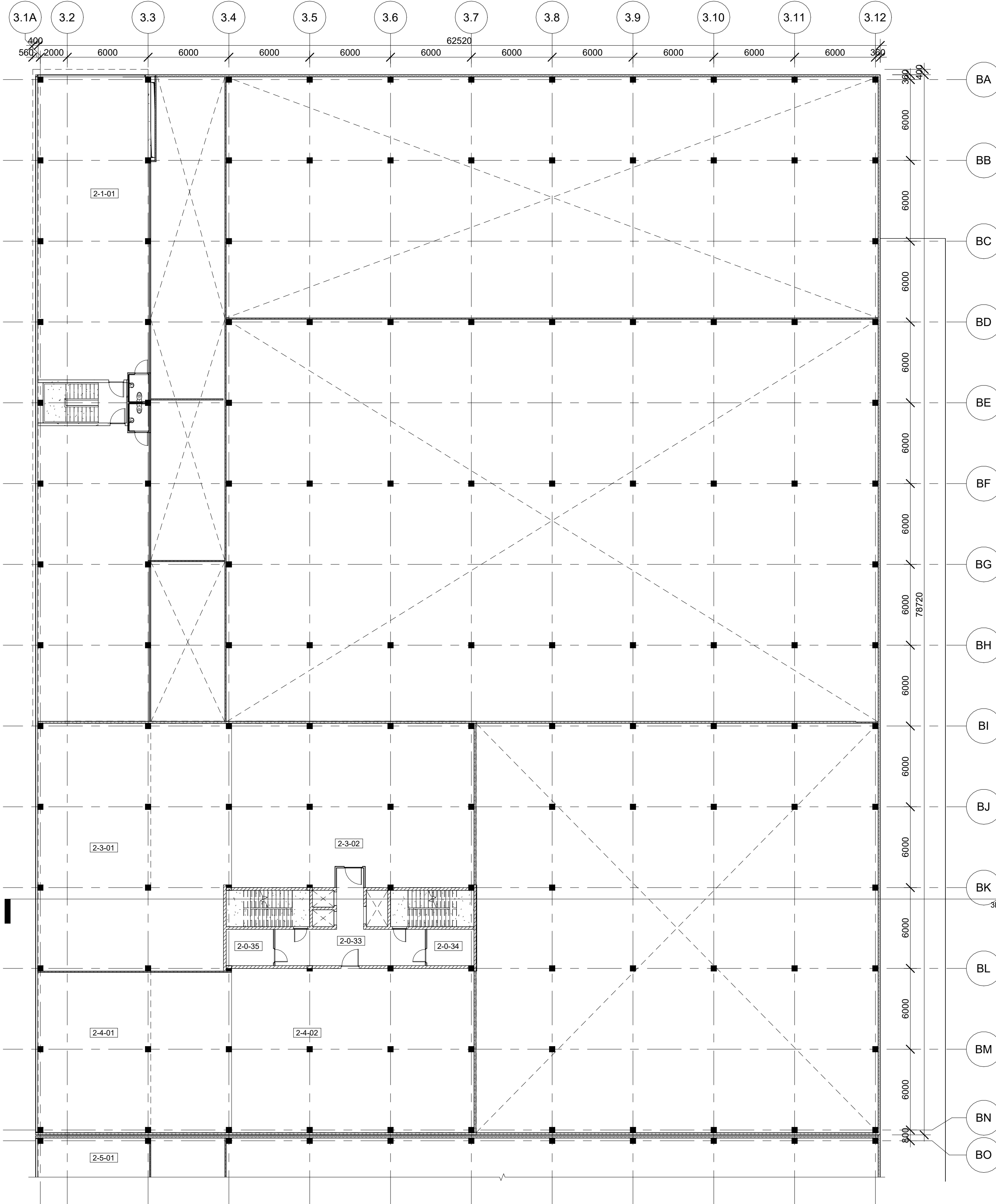
1 Pastatas 3B - Antro aukšto planas 1 : 200
