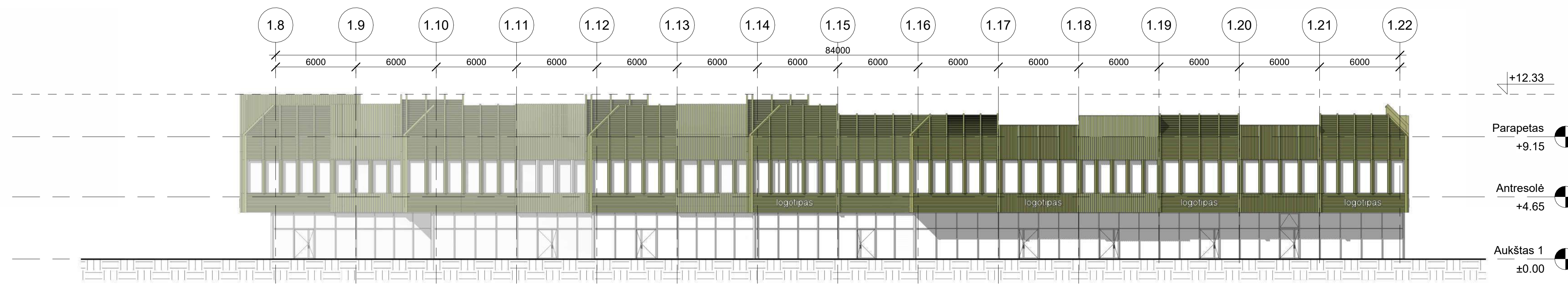
3 Pietryčių fasadas 1 : 200
