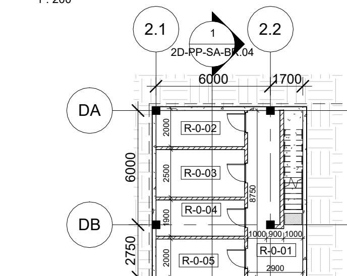
R1 Pastatas 2D - Rūsio planas
