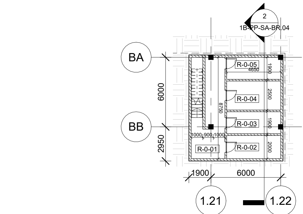
R Pastatas 1B - Rūsio planas 1 : 200
