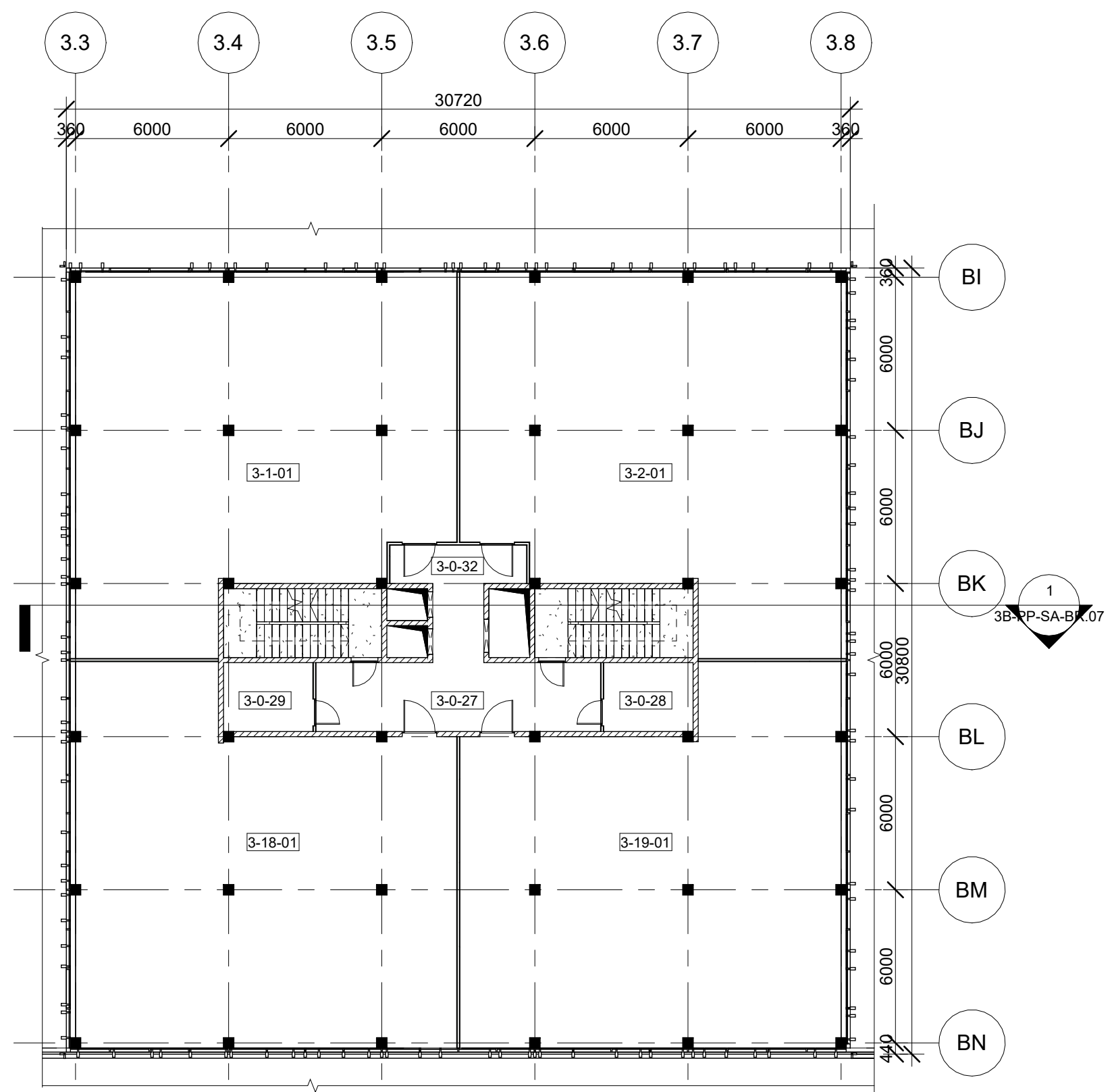
2 Pastatas 3B - Trečio-septinto aukšto planas 1 : 200
