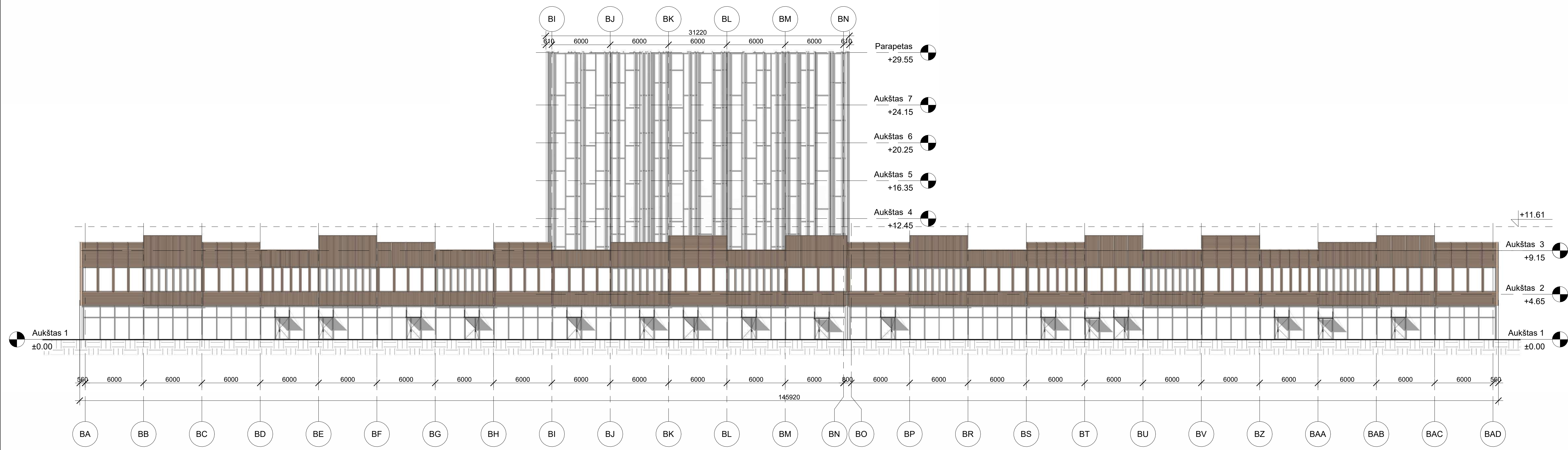
4 | Pietvakarių fasadas 1 : 200
