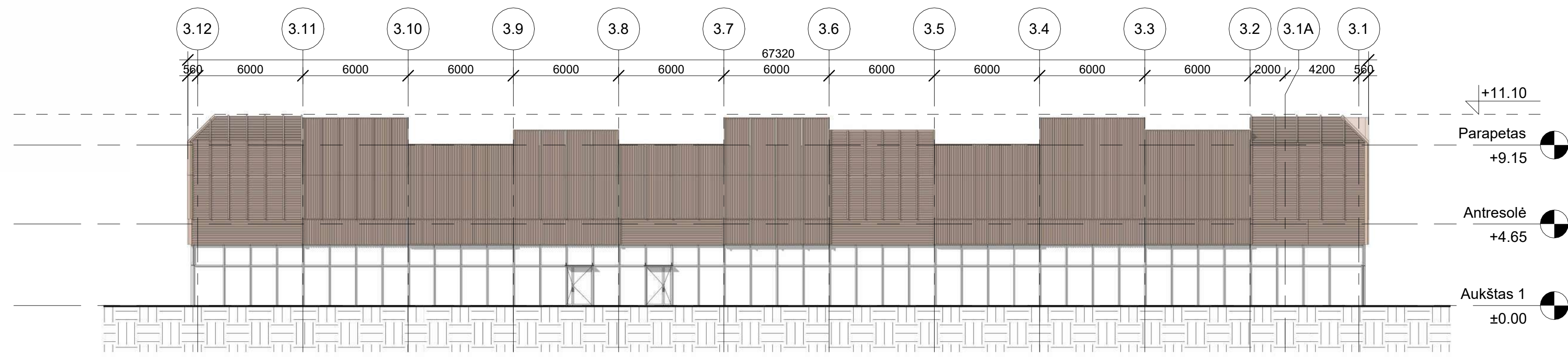
1 | Šiaurės-vakarų fasadas 1 : 200
