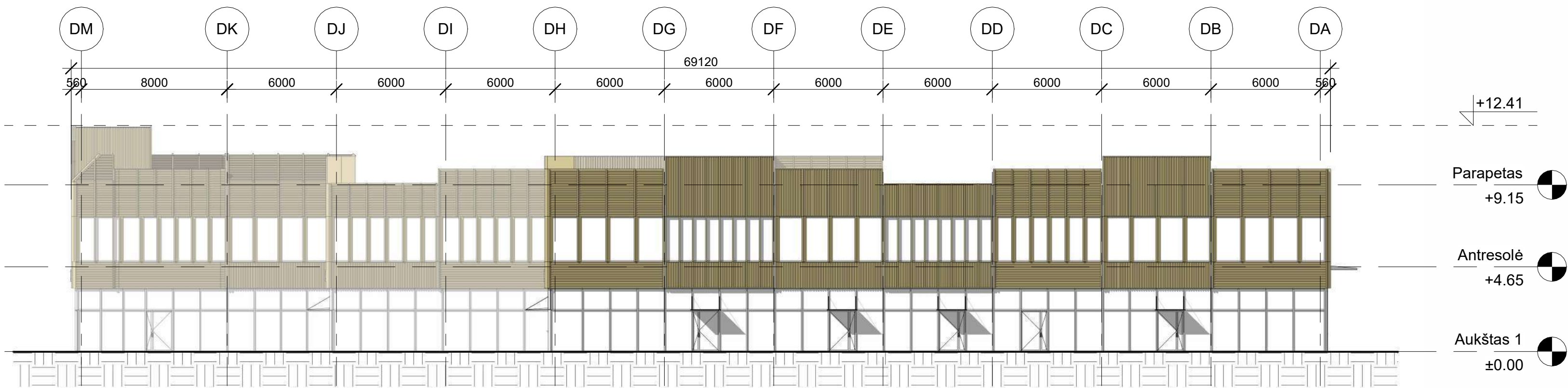
2 Šiaurės-rytų fasadas 1 : 200
