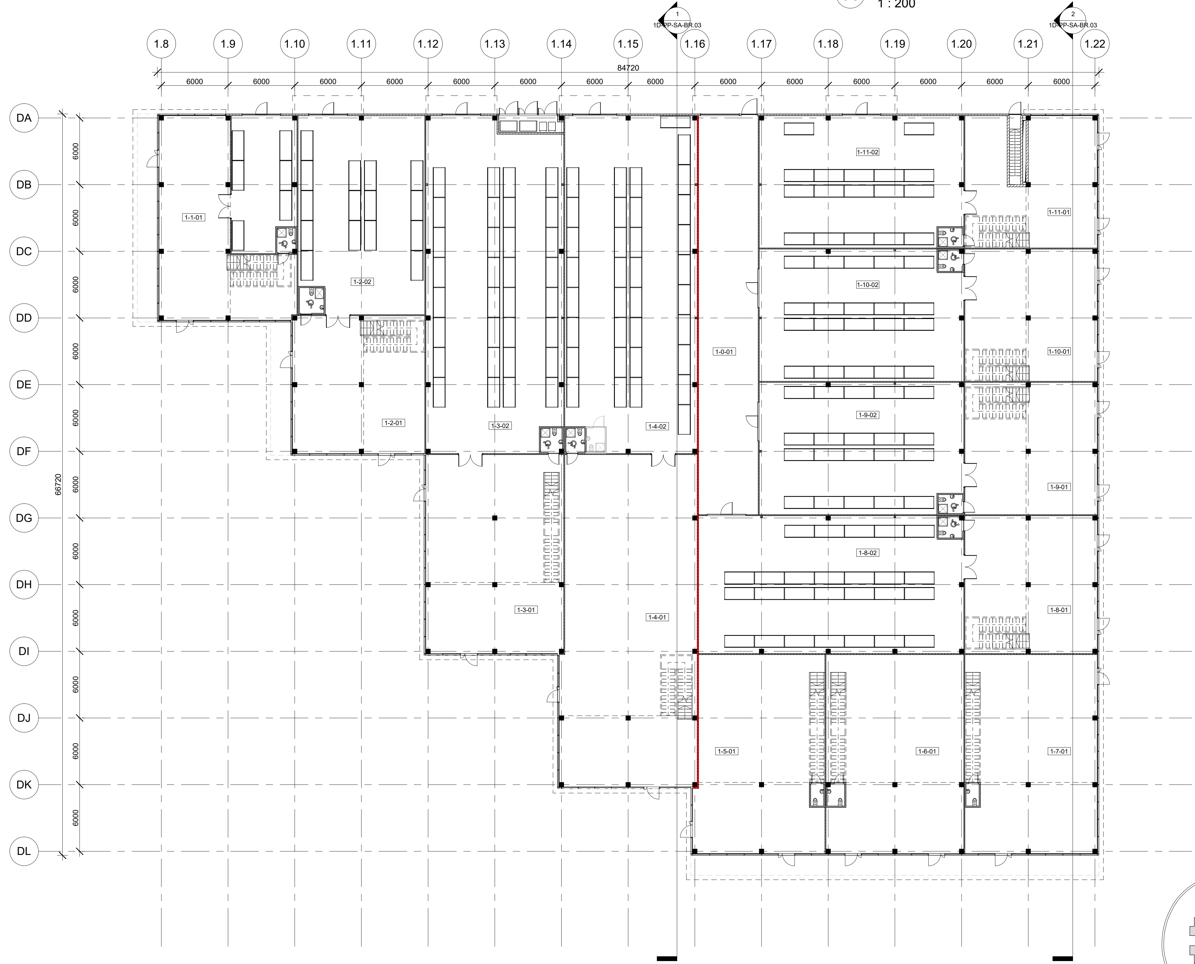
Pastatas 1D - Pirmo aukšto planas 1 : 200
