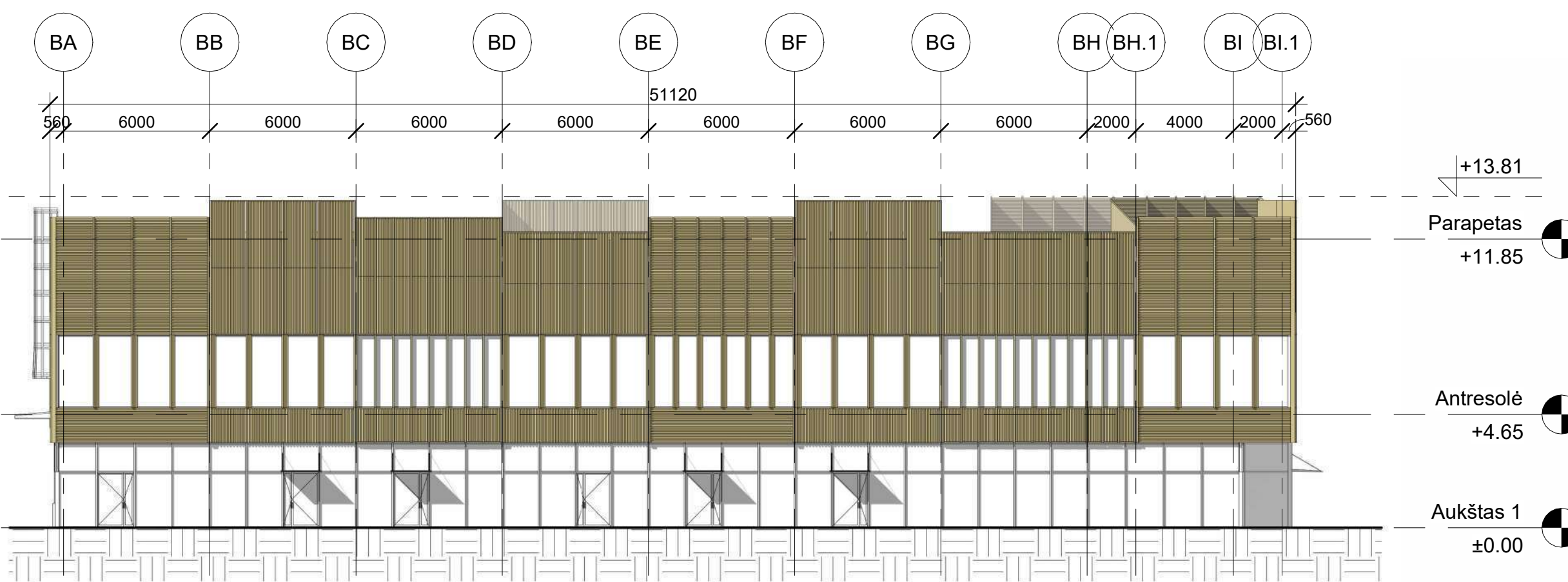
4 | Pietvakarių fasadas 1 : 200
