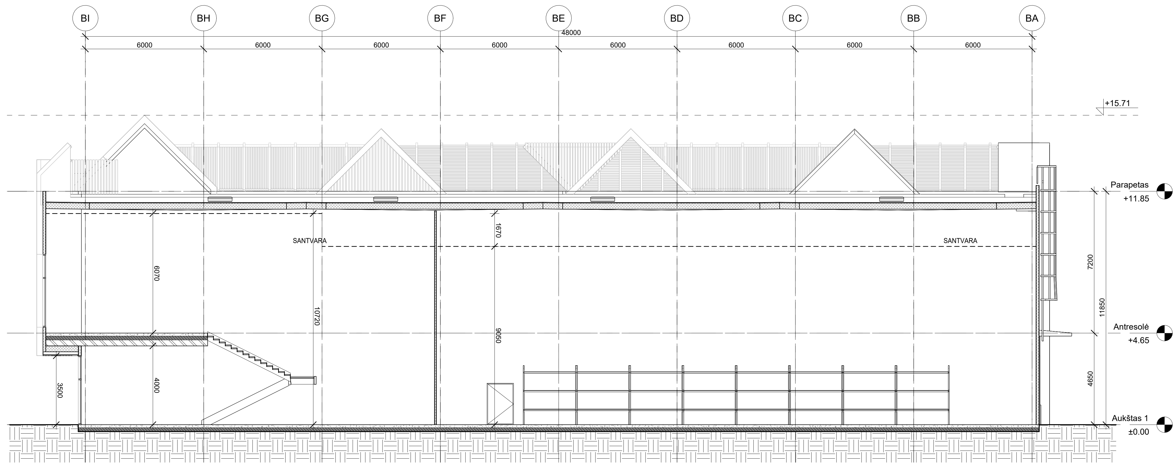
1 Pastatas 1B - Pjūvis 1-1 1 : 100
