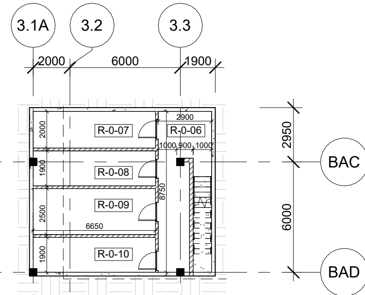
1 Pastatas 3B - Pirmo aukšto planas
