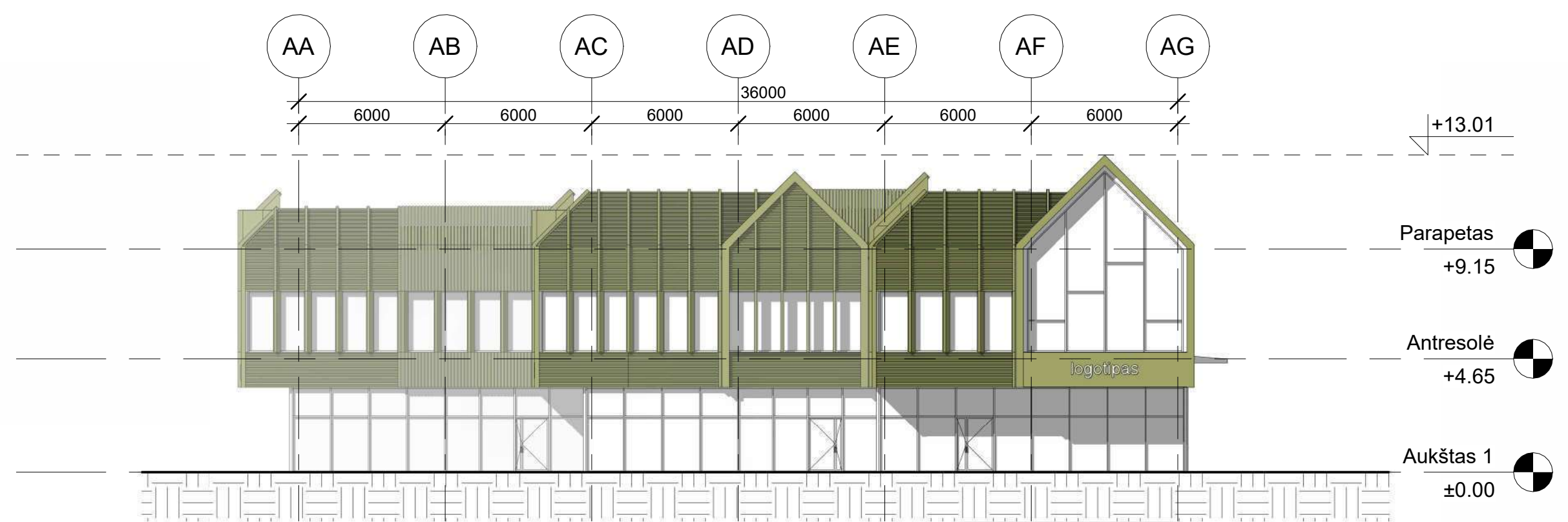
4 Pietvakarių fasadas 1 : 200
