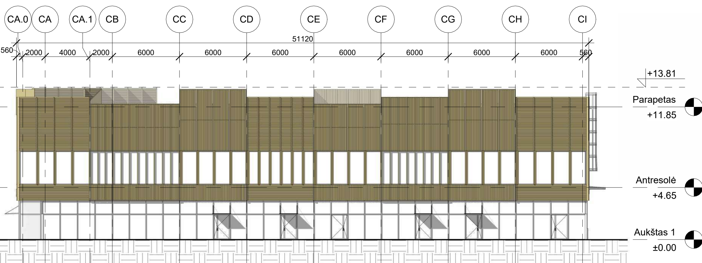
3 Pietryčių fasadas 1 : 200
