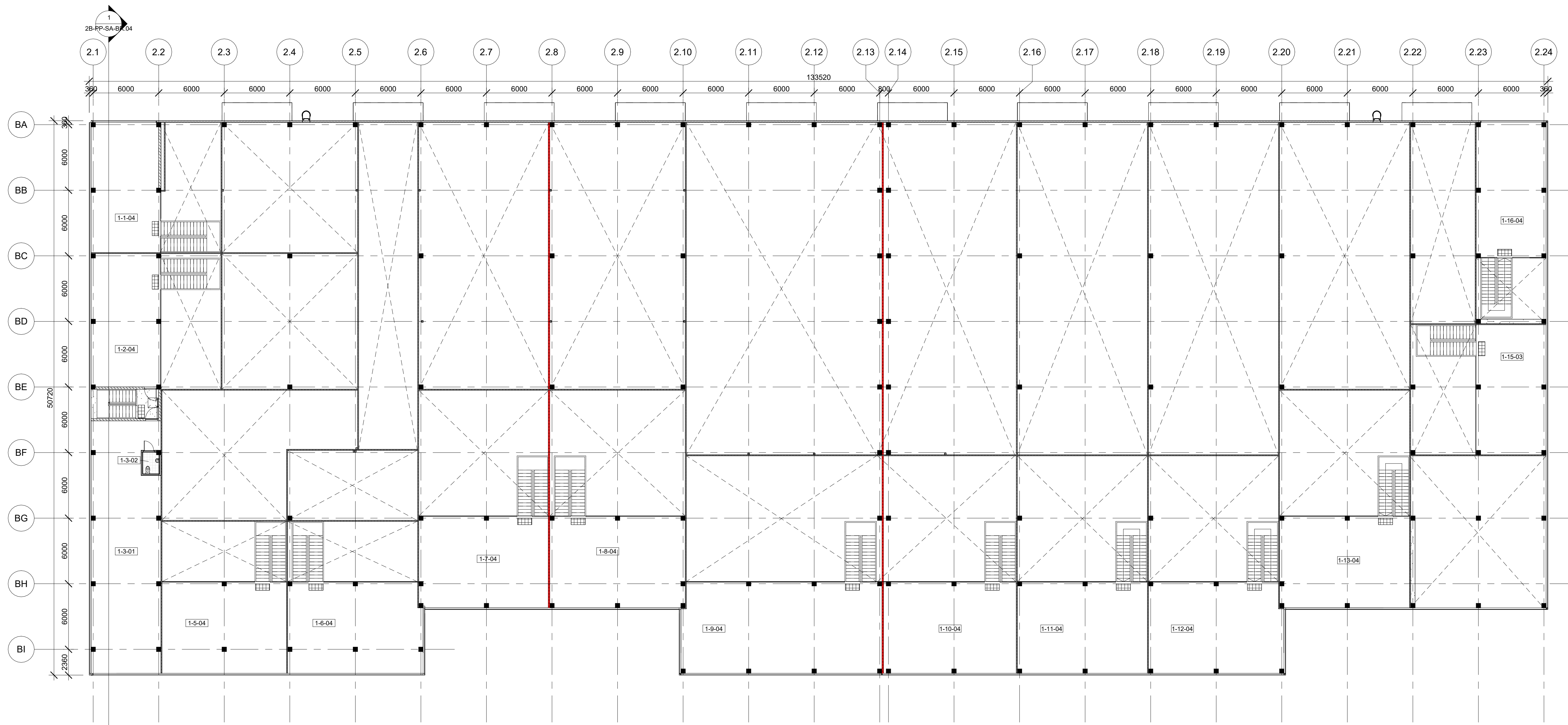
1 Pastatas 2B - Antresolės planas 1 : 200
