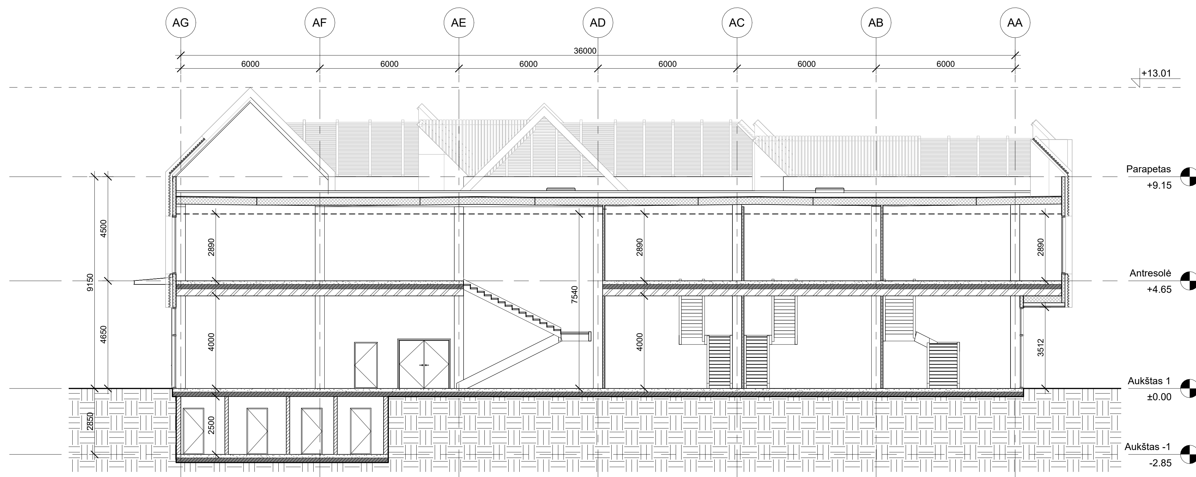
2 Pastatas 1A - Pjūvis 2-2 1 : 100
