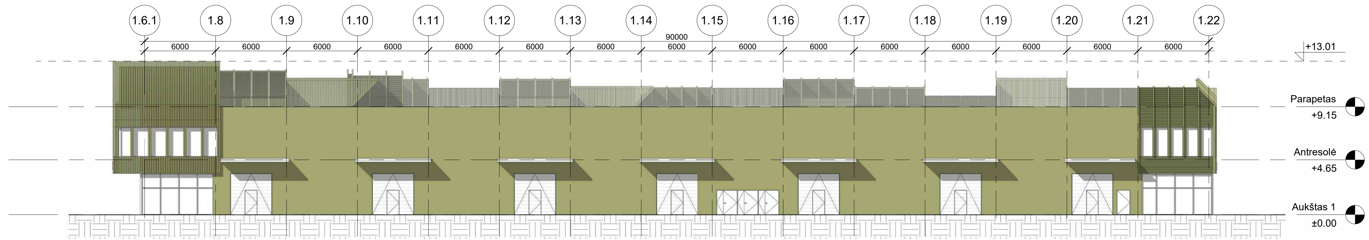
3 Pietryčių fasadas 1 : 200
