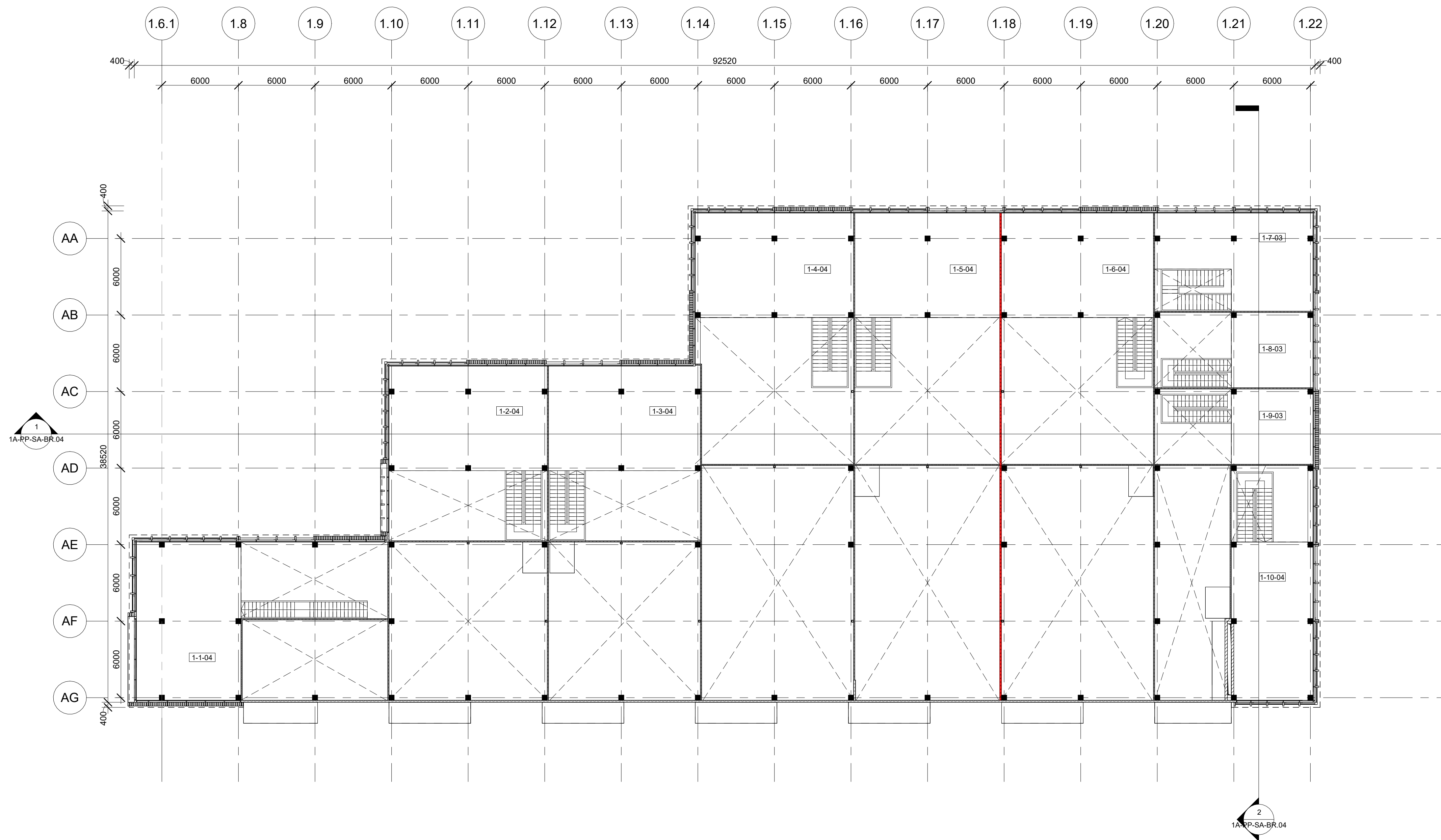
1 Pastatas 1A - Antresolės planas 1 : 200
