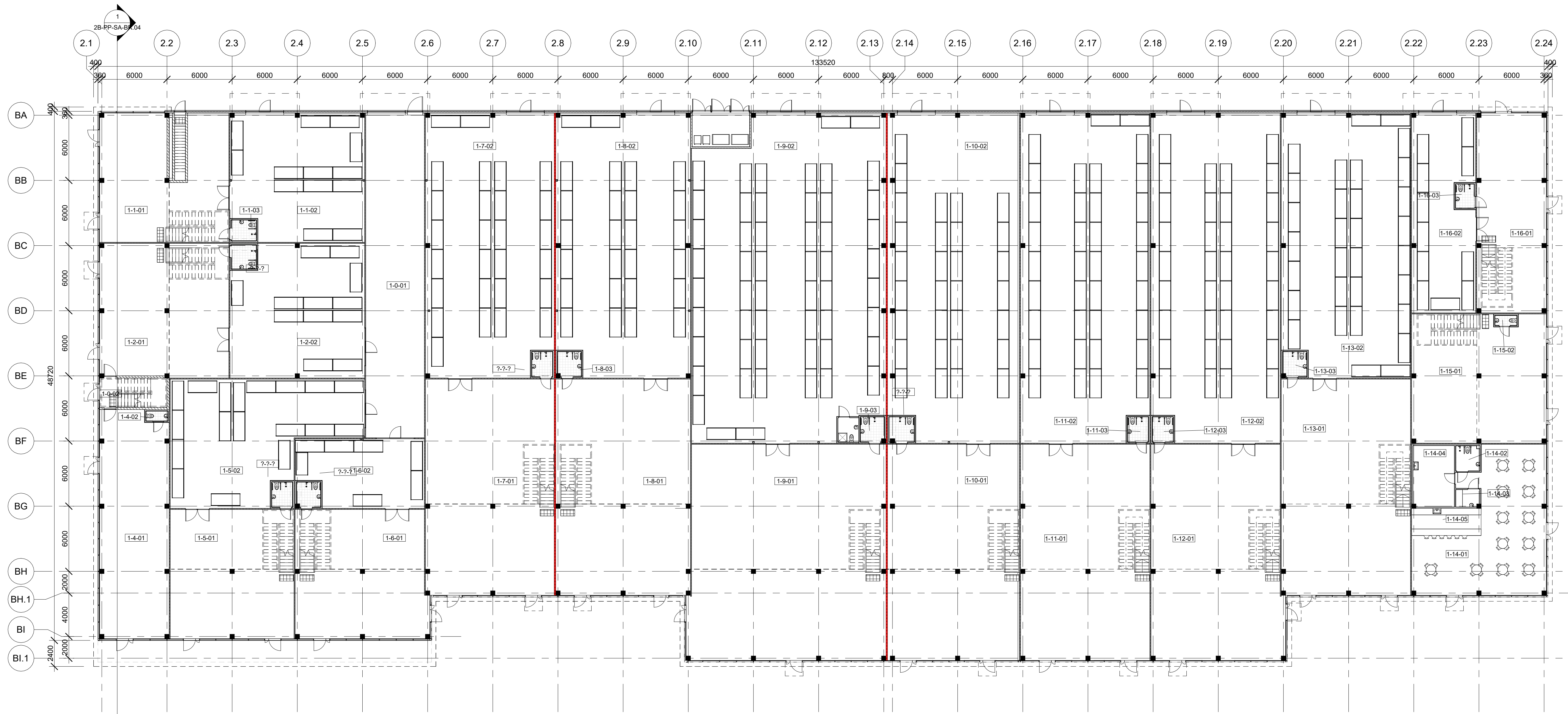
1 Pastatas 2B - Pirmo aukšto planas 1 : 200
