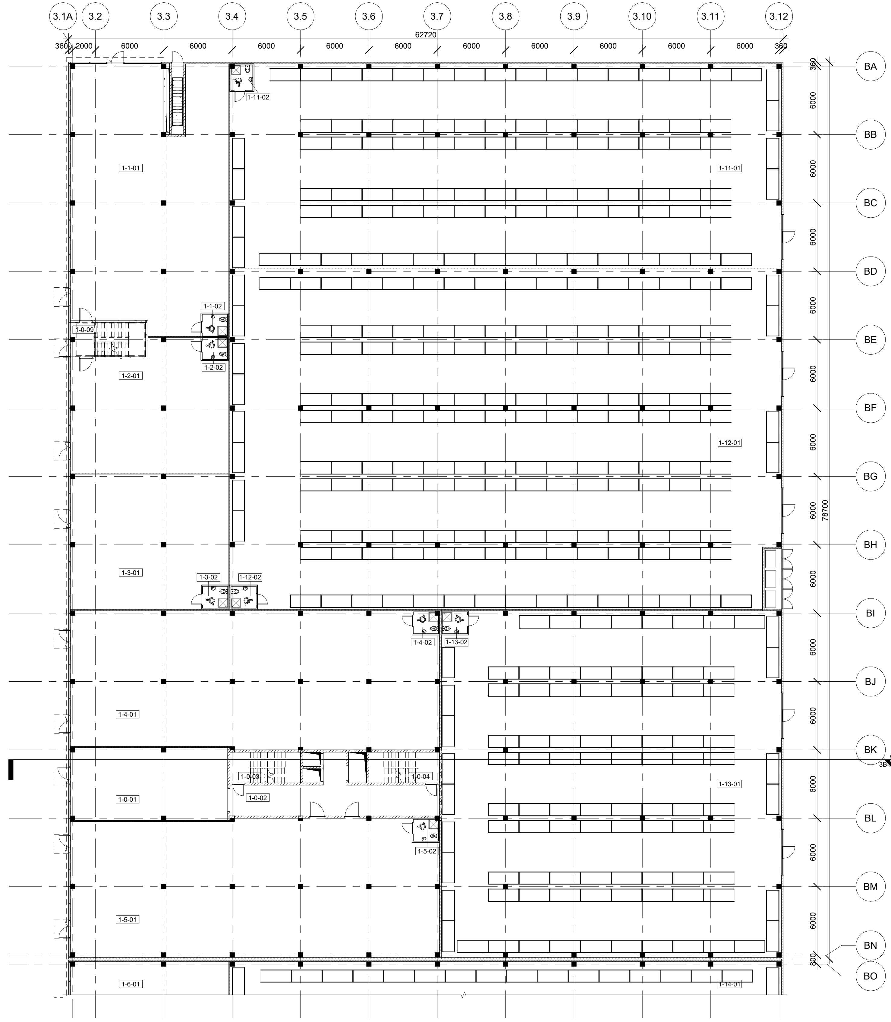
1 | Pastatas 3B - Pirmo aukšto planas 1 : 200
