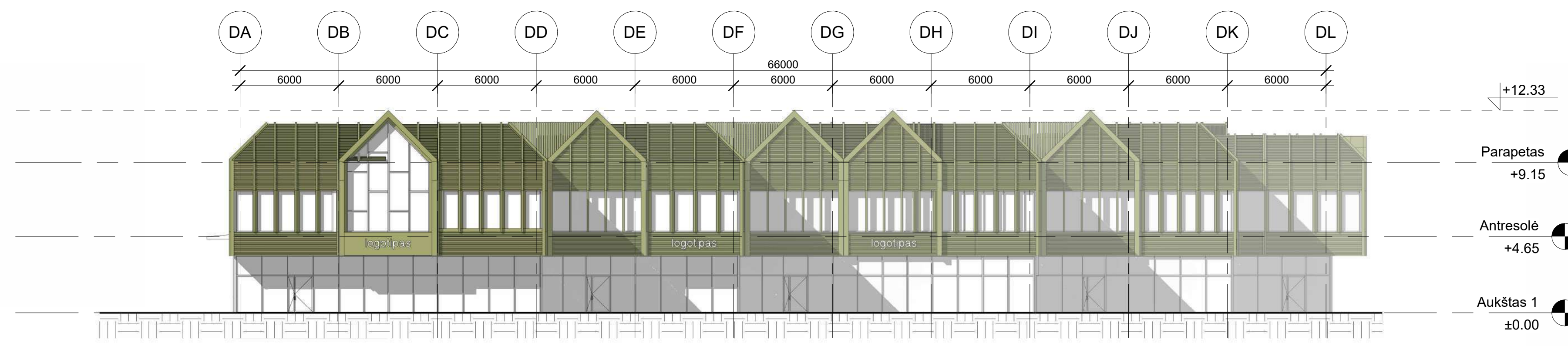
4 Pietvakarių fasadas 1 : 200
