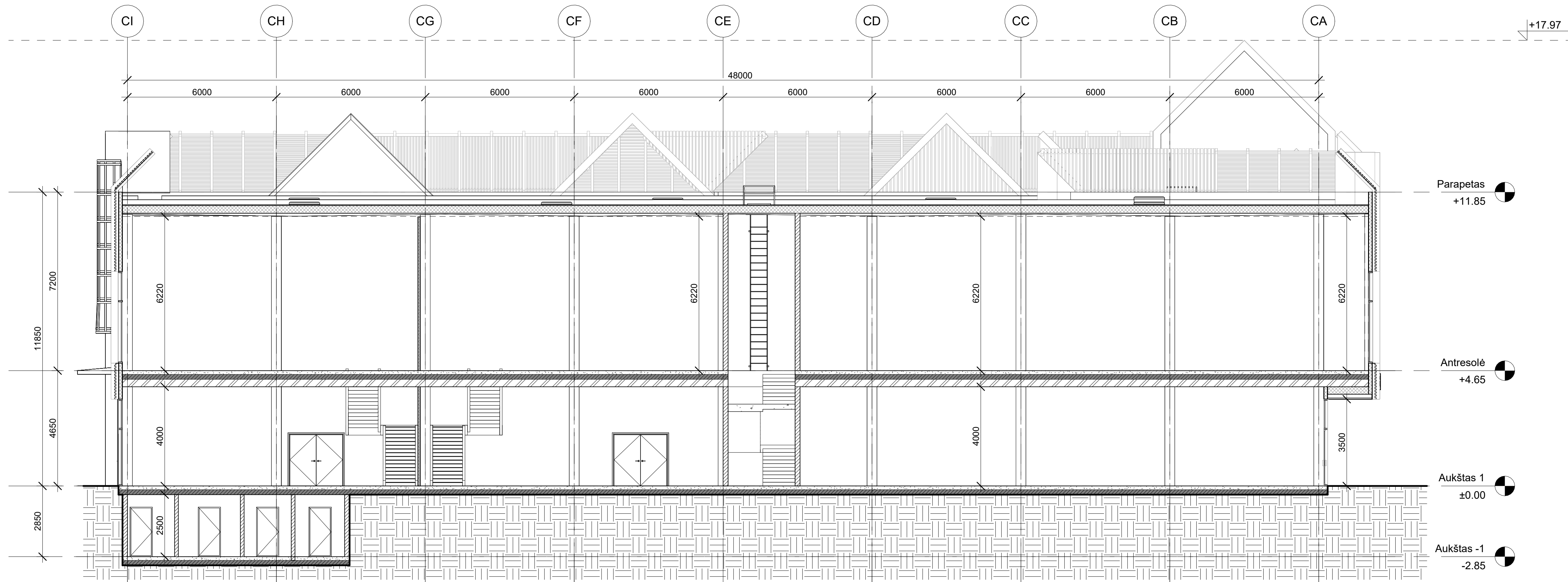
2 Pjūvis 1C 2-2 1 : 100
