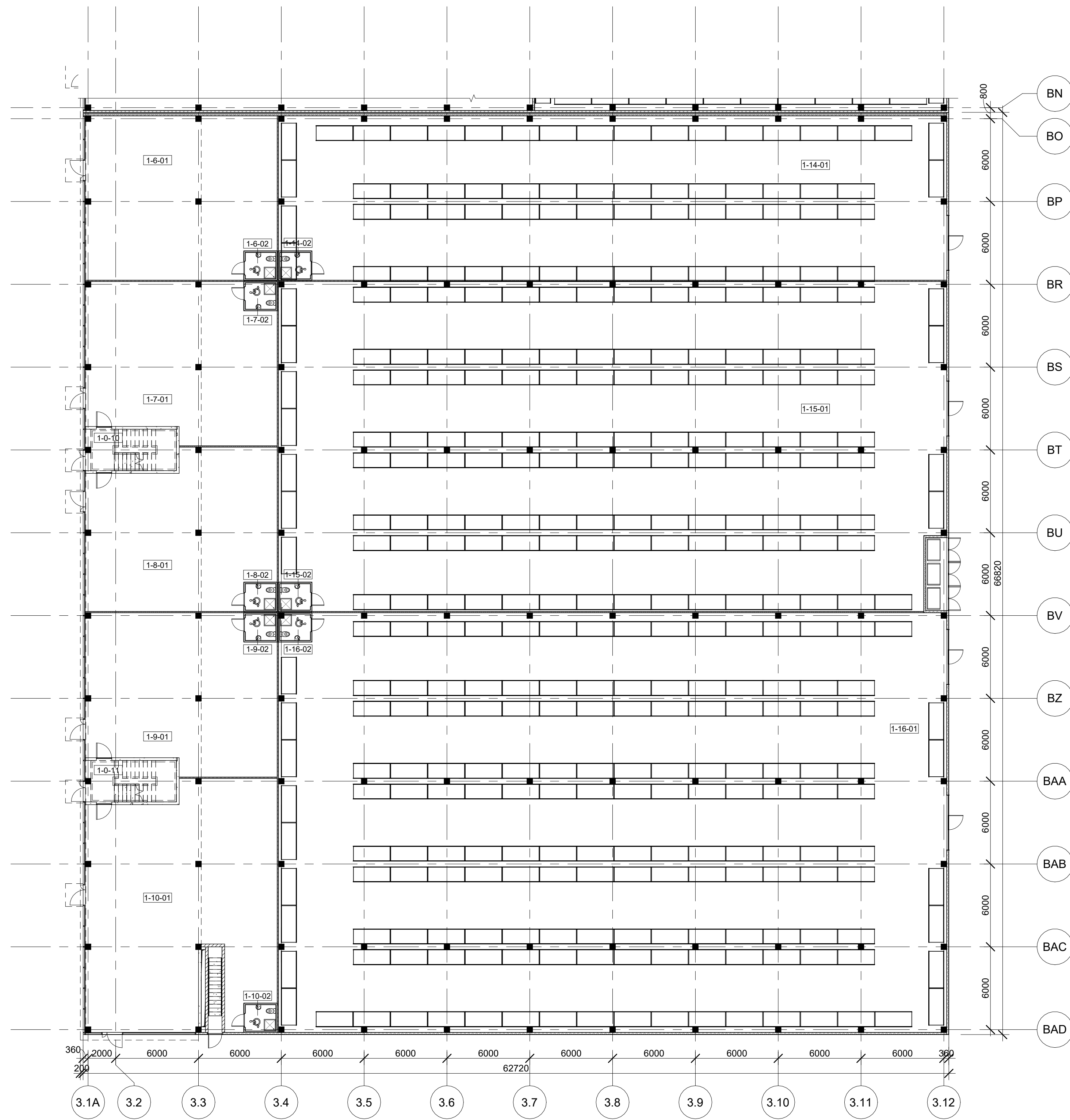
1 Pastatas 3B - Pirmo aukšto planas
