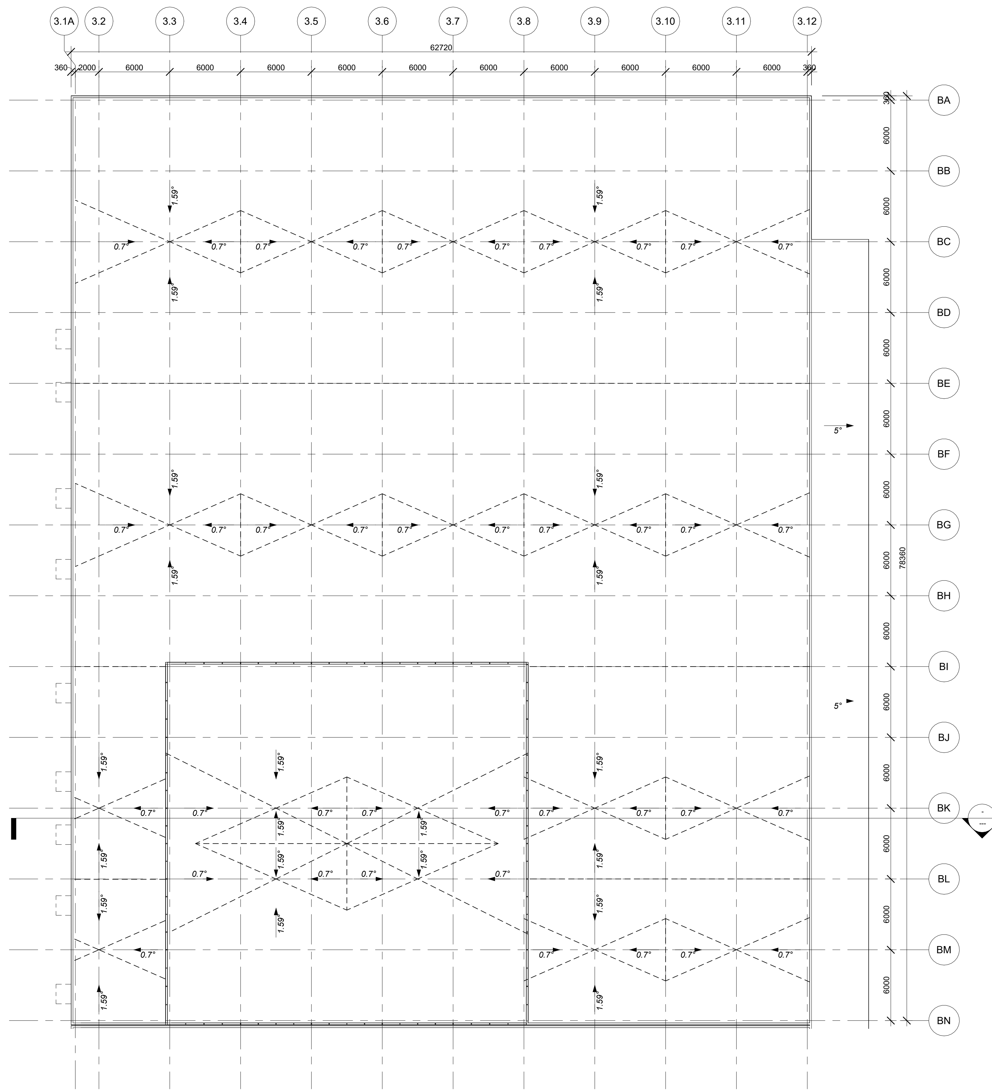
1 Pastatas 3B - Stogo planas 1 : 200
