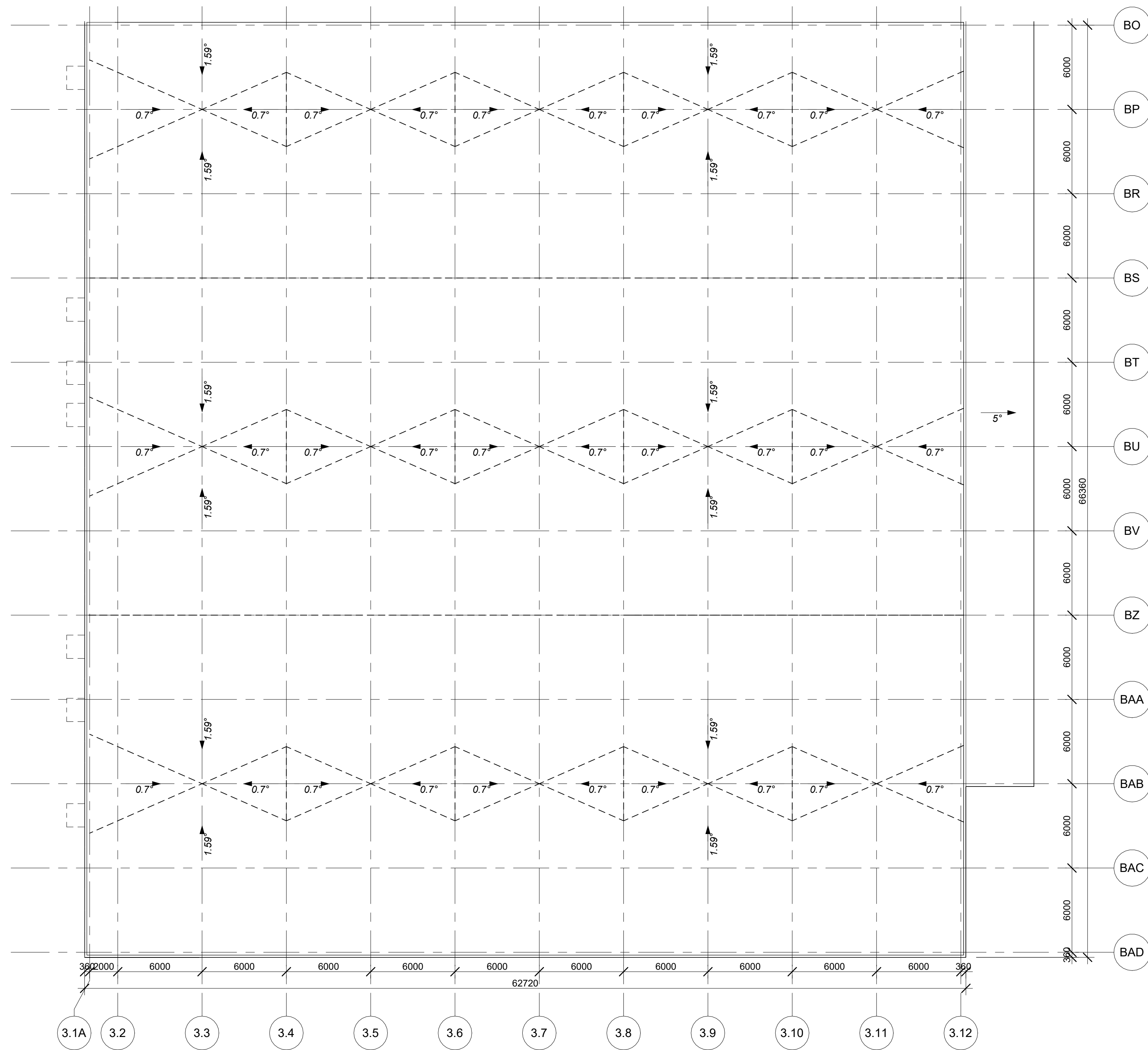
1 Pastatas 3B - Stogo planas 1 : 200
