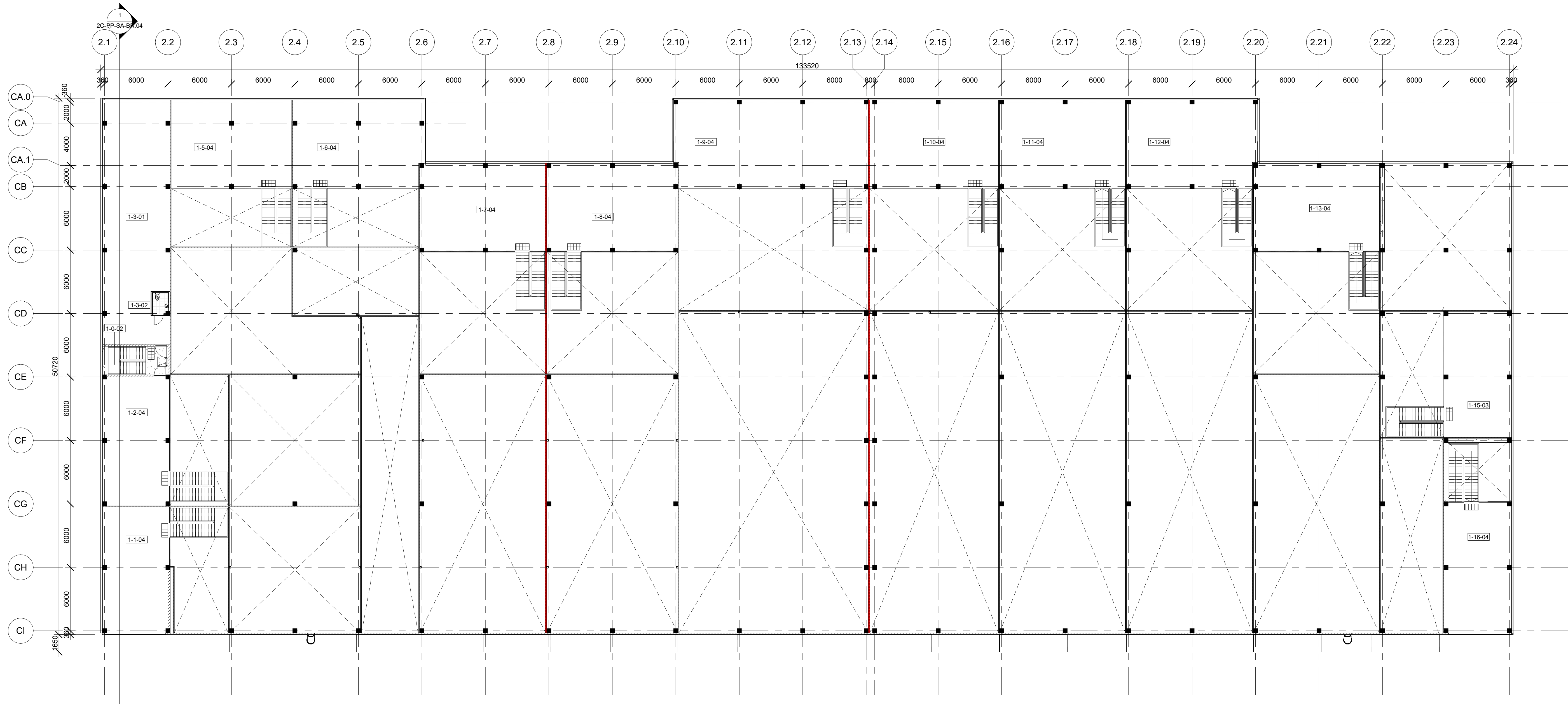
1 Pastatas 2C - Antresolės planas
