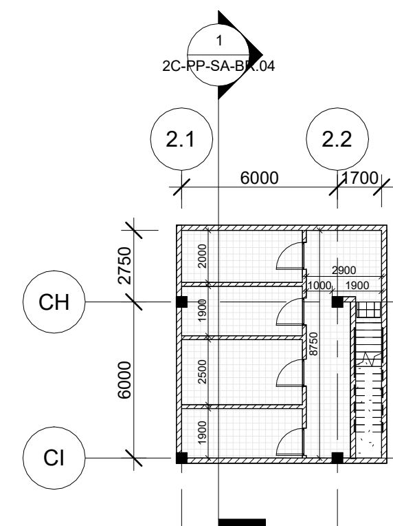
R1 Pastatas 2C - Rūsio planas 1 : 200
