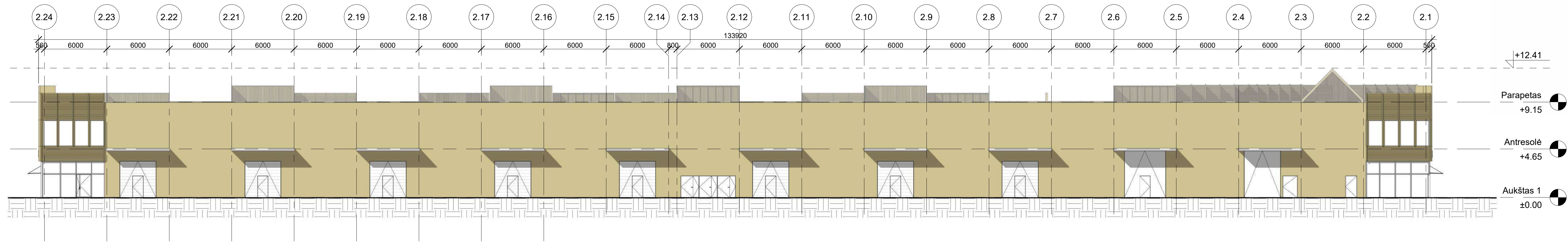
1 Šiaurės-vakarų fasadas 1 : 200
