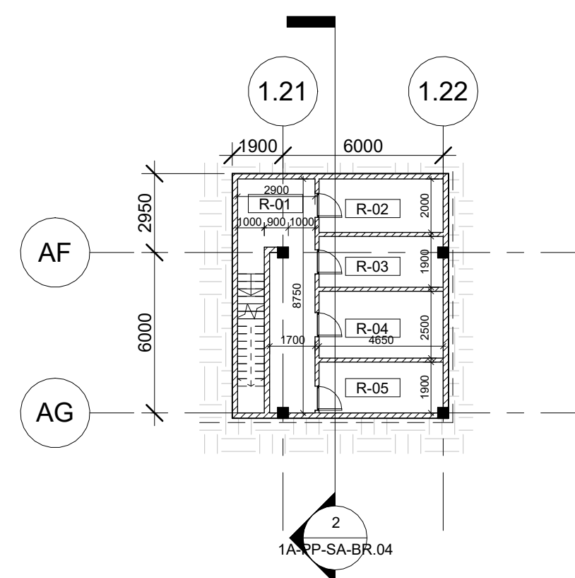
R Pastatas 1A - Rūsio planas
