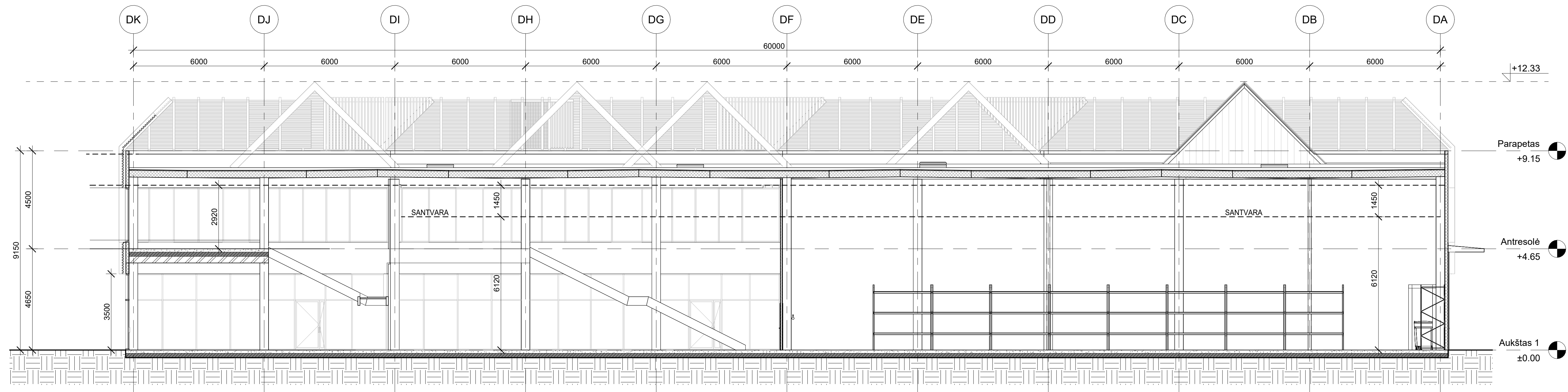
1 Pastatas 1D - Pjūvis 1-1 1 : 100
