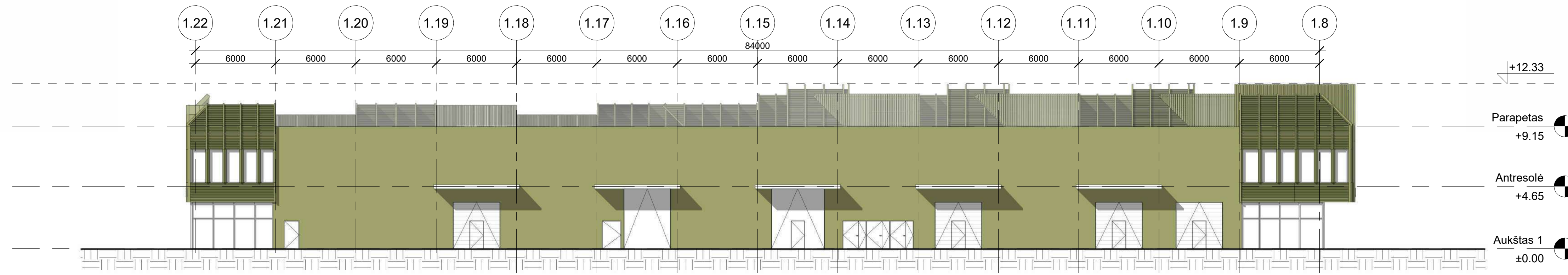
1 Šiaurės-vakarų fasadas 1 : 200
