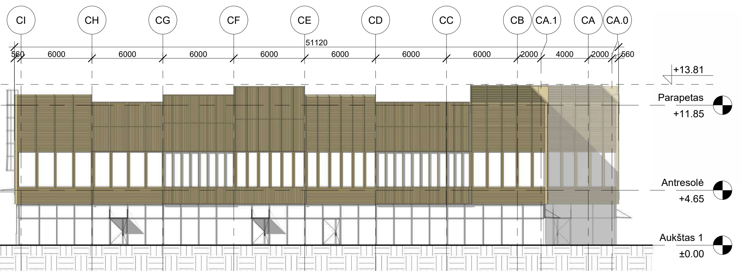
4 Pietvakarių fasadas 1 : 200
