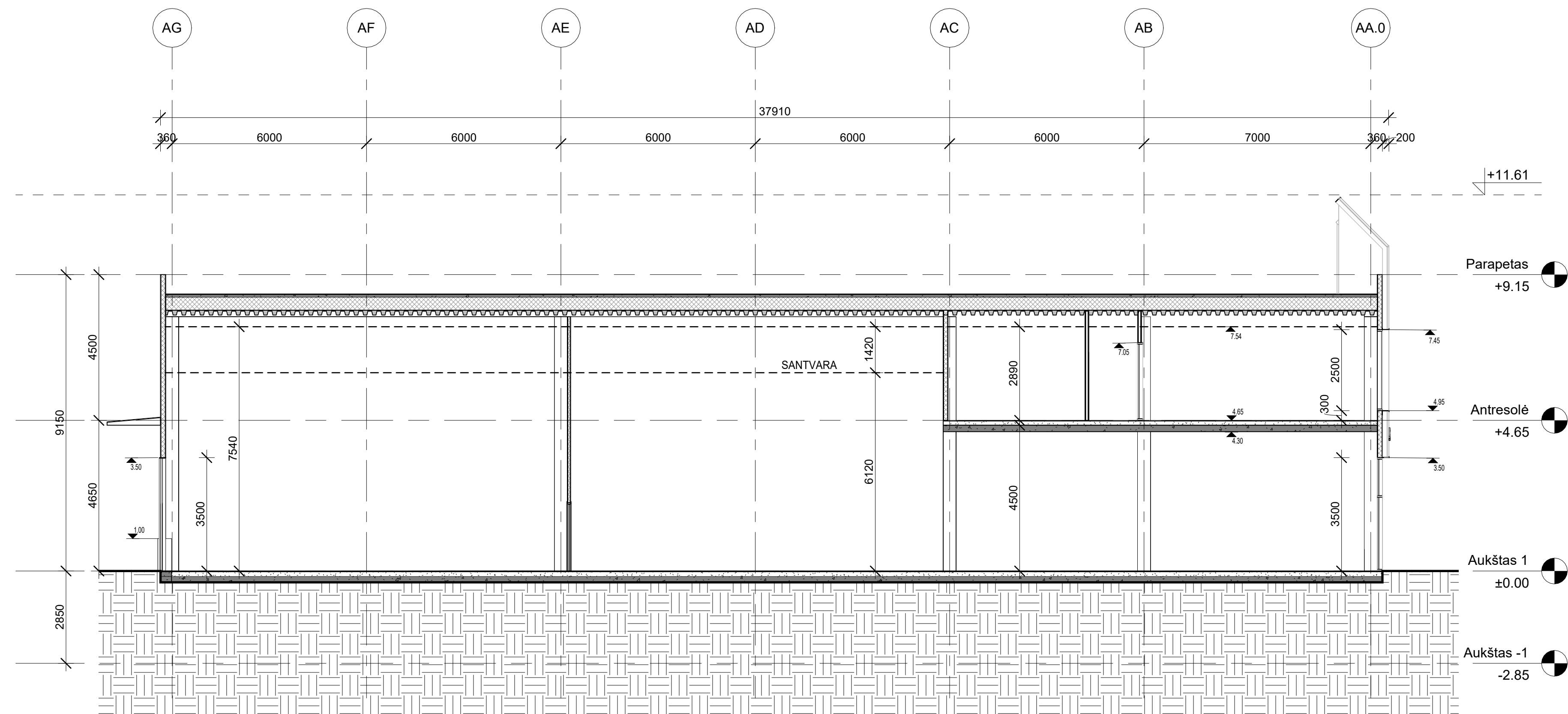
1 Pastatas 2A - Pjūvis 1-1 1:100
