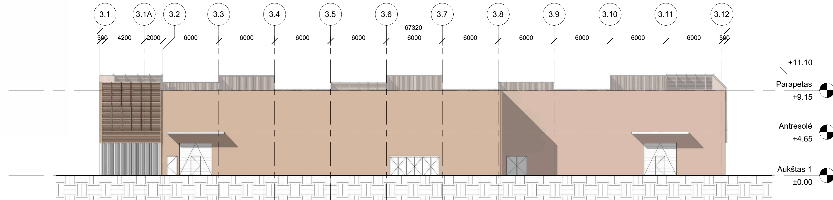
3 | Pietryčių fasadas 1 : 200
