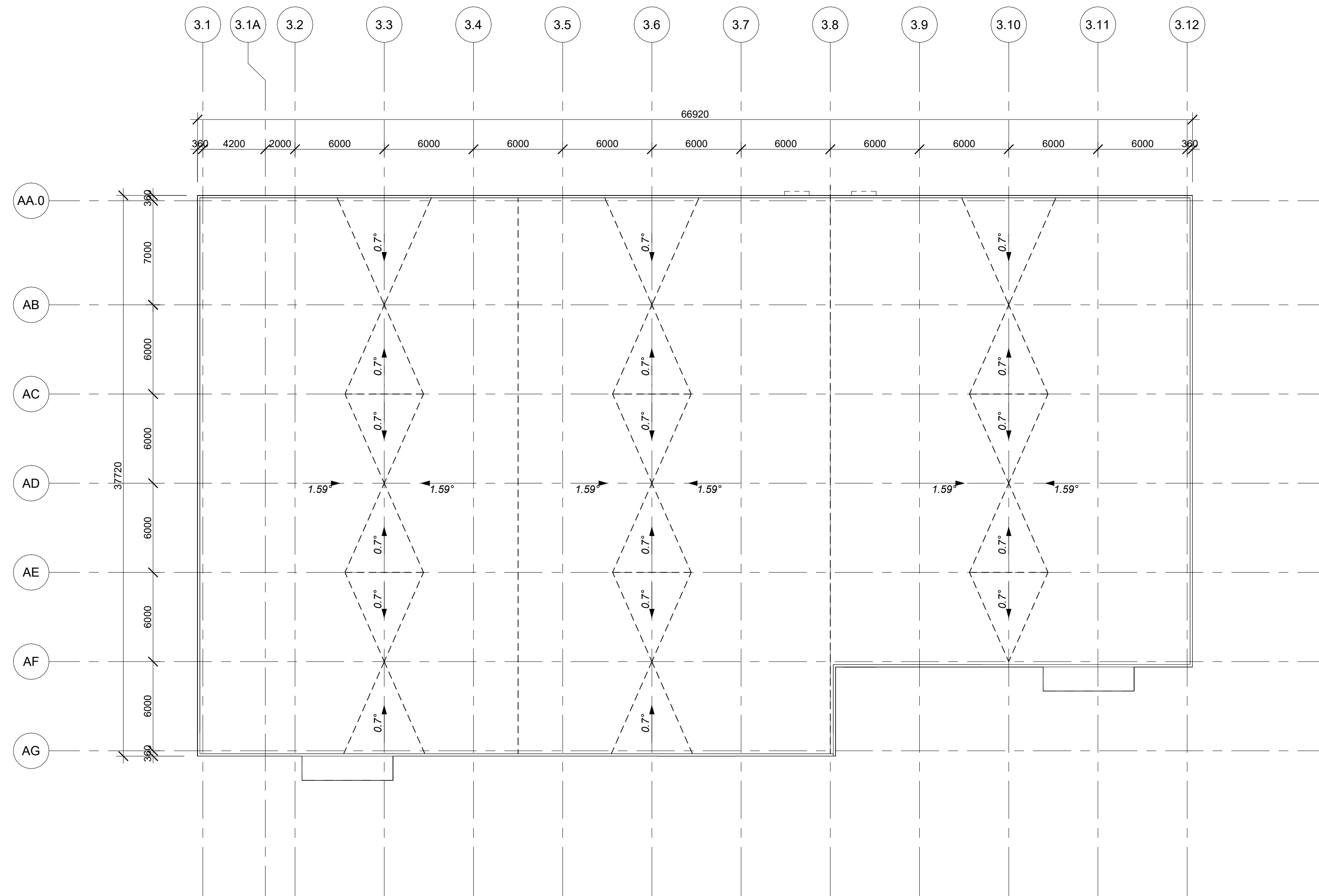
1 | Pastatas 3A - Stogo planas 1 : 200
