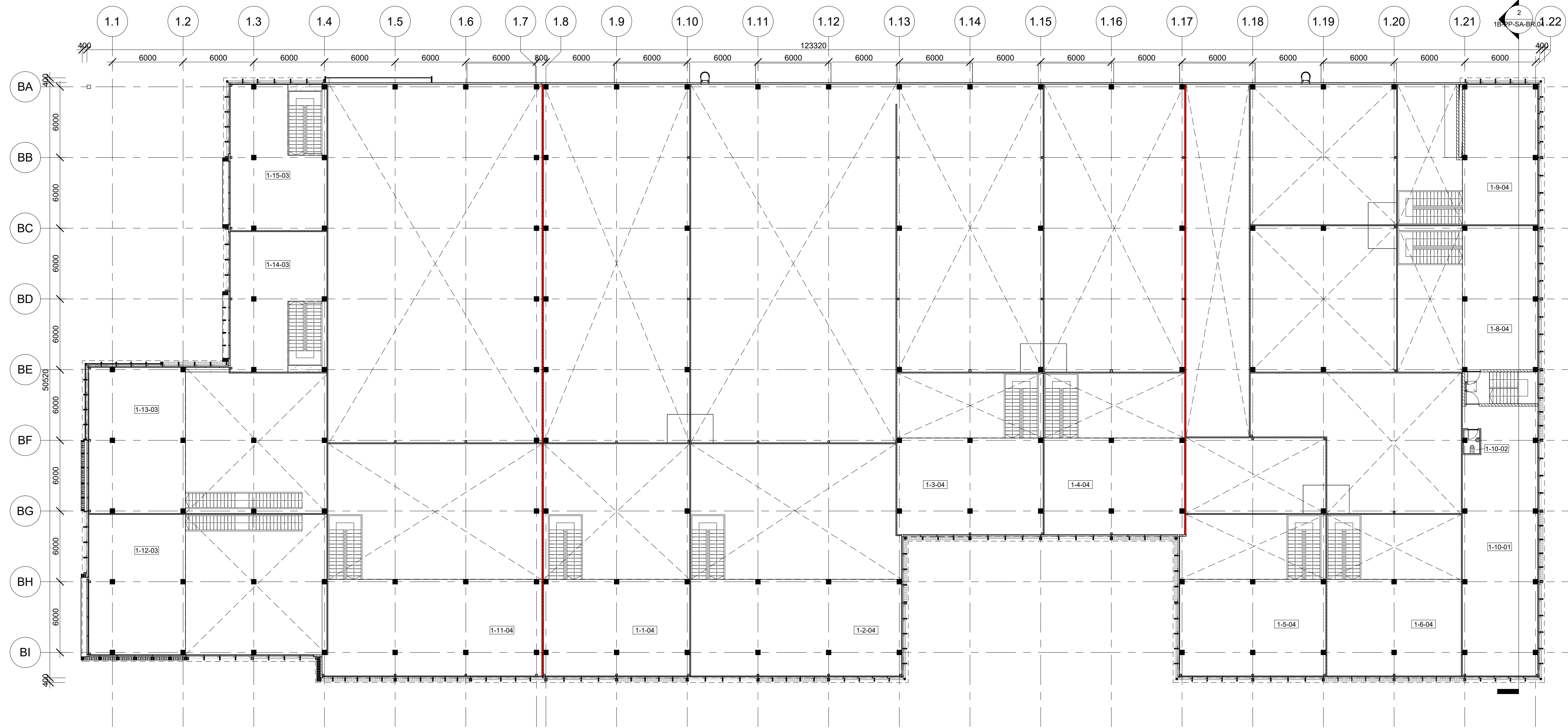
1 Pastatas 1B - Antresolės planas 1 : 200
