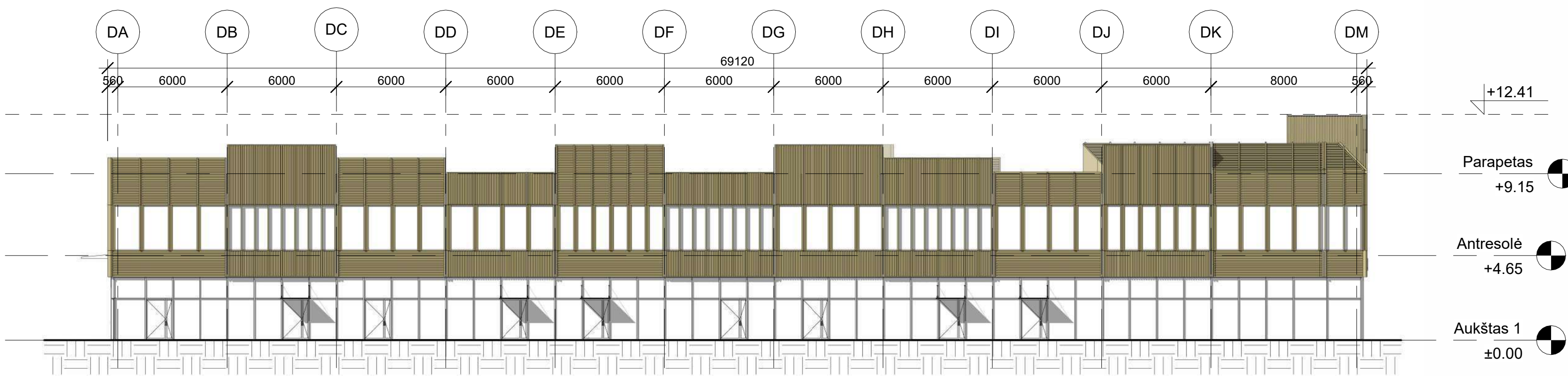
4 Pietvakarių fasadas 1 : 200
