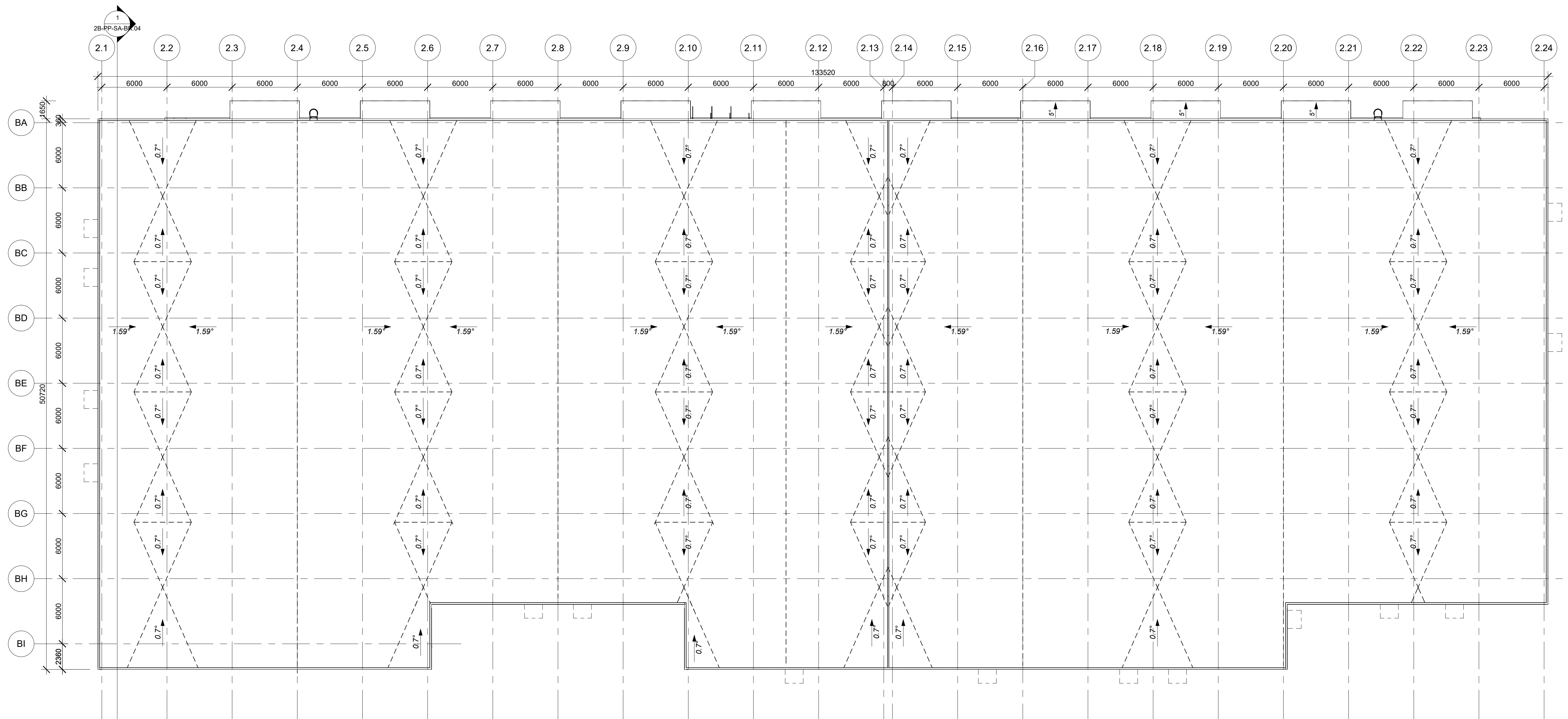
1 Pastatas 2B - Stogo planas 1 : 200
