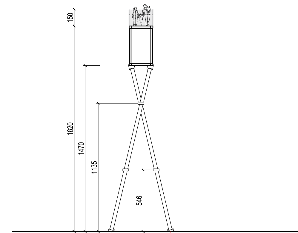
PJŪVIS A-A M1:200
