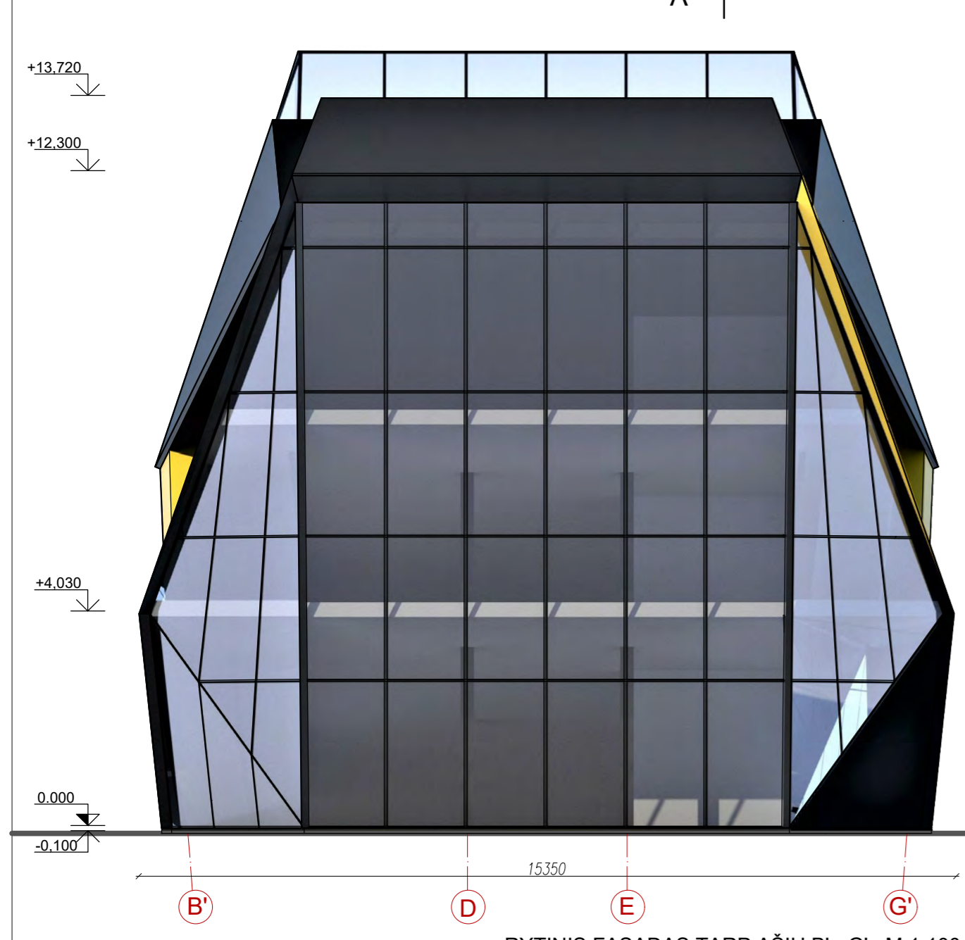
RYTINIS FASADAS TARP AŠIŲ B' - G' M 1:100
