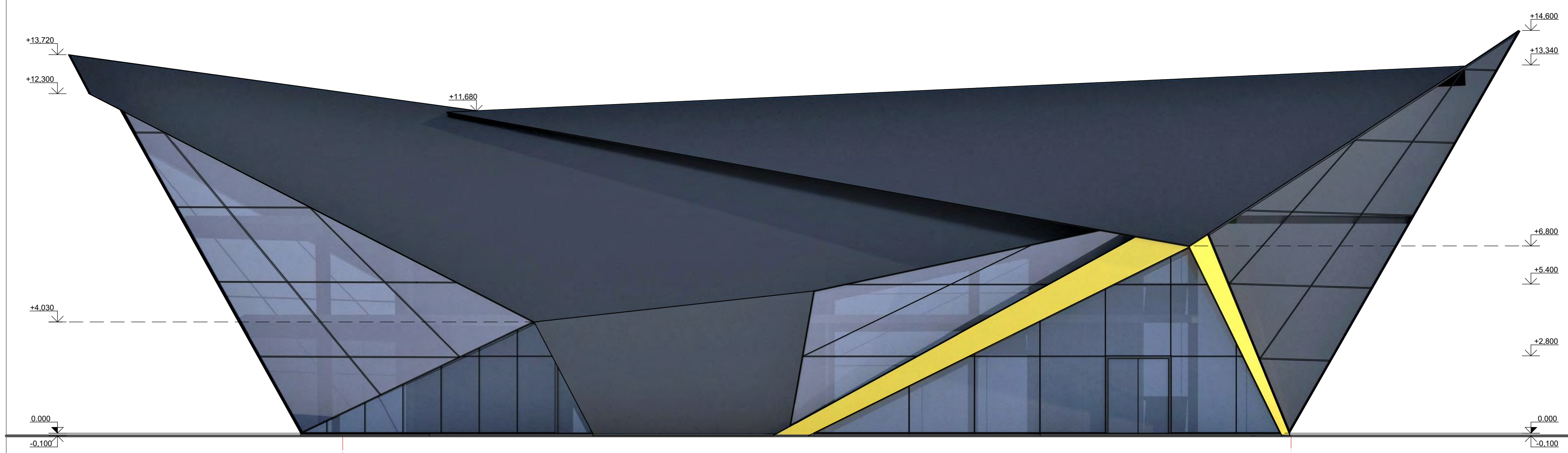
ŠIAURINIS FASADAS TARP AŠIŲ 8 - 1 M 1:100
