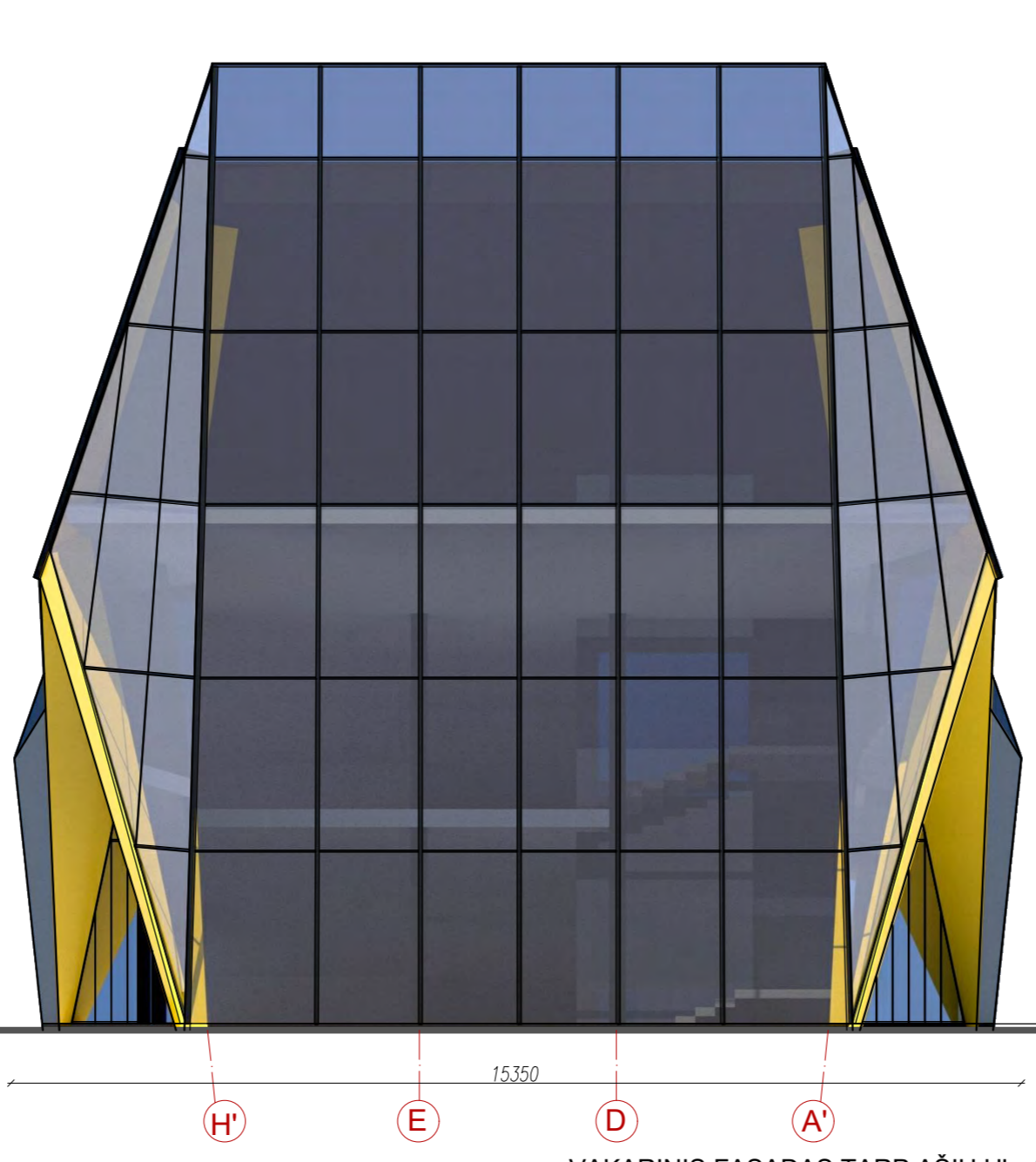
VAKARINIS FASADAS TARP AŠIŲ H' - A' M 1:100
