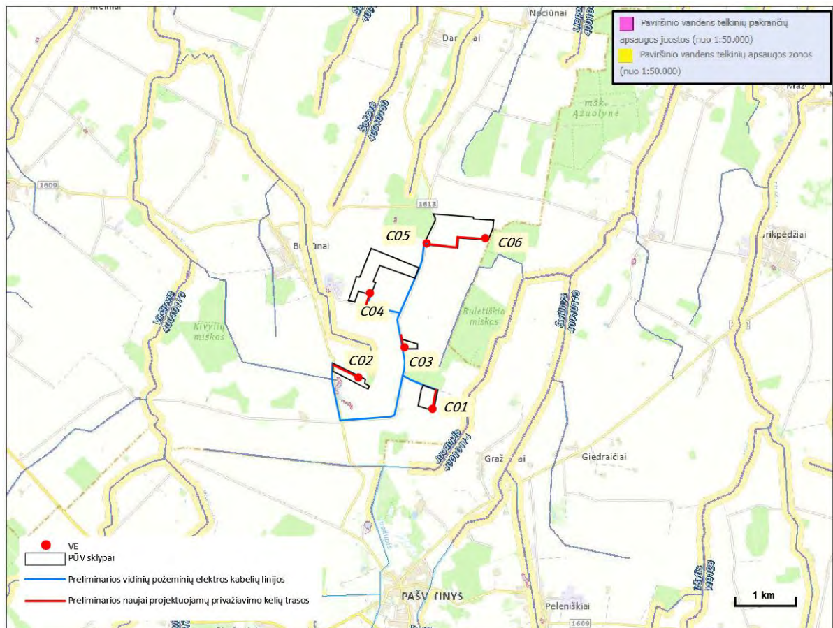
3.7.1 pav. VE, kabelių ir kelių išdėstymas paviršinių vandens telkinių pakrantės apsaugos juostų ir zonų atžvilgiu. Nei vienas planuojamų VE žemės sklypai nesiriboja su upėmis. (3.7.2 pav.).
