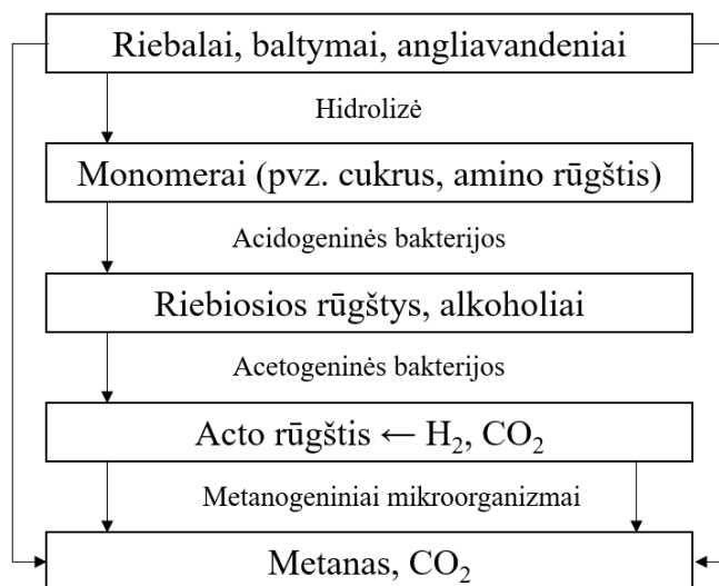
2 pav. Pagrindinės anaerobinės biodegradacijos stadijos
