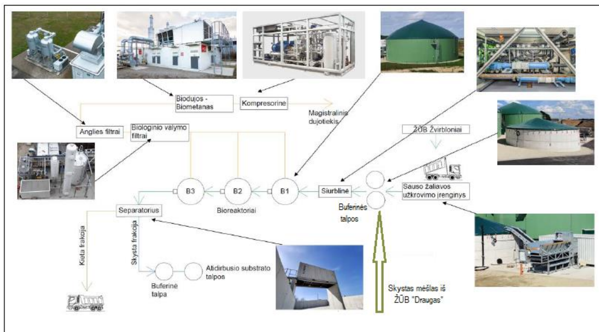
1 pav. Biodegalų gamybos principinė schema
