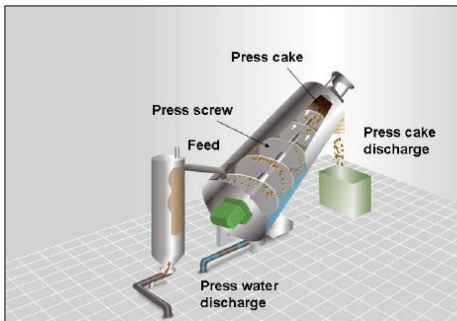
7 pav. Separavimo įrenginio veikimo principas
