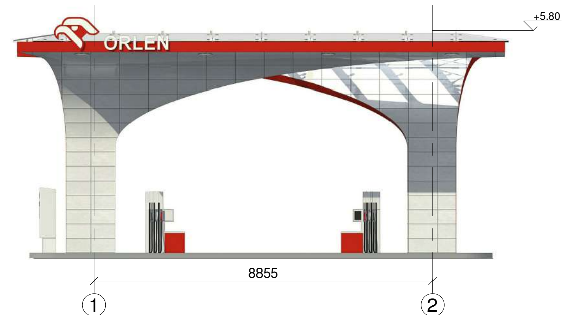
Šiaurės vakarų fasadas 1 : 100
