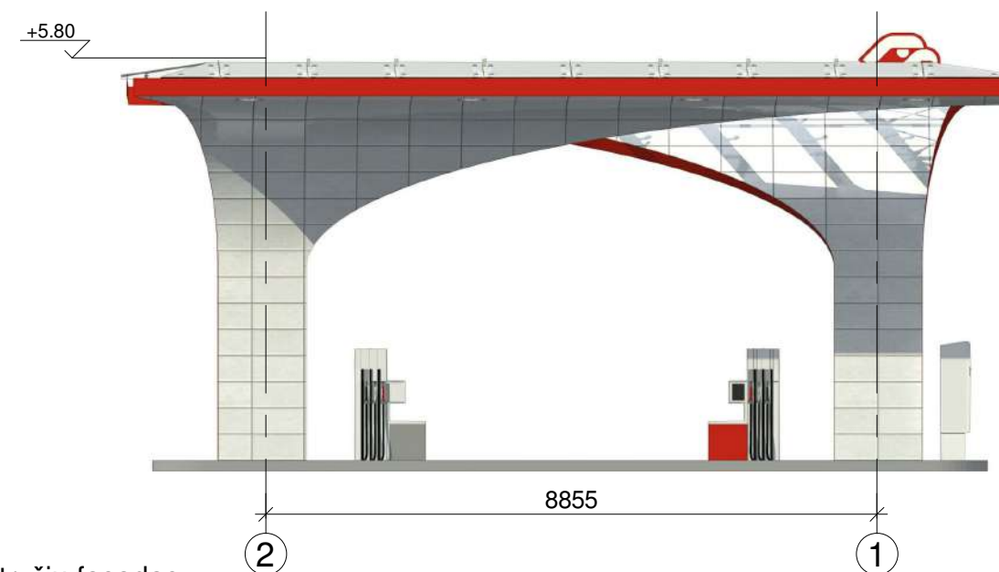
Pietryčių fasadas 1 : 100
