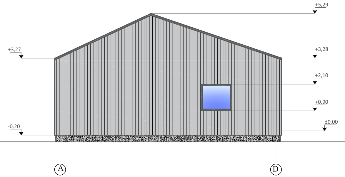
FASADAS D-A M 1:100
