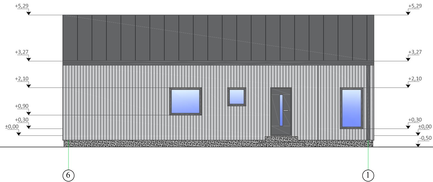
FASADAS 6-1 M 1:100
