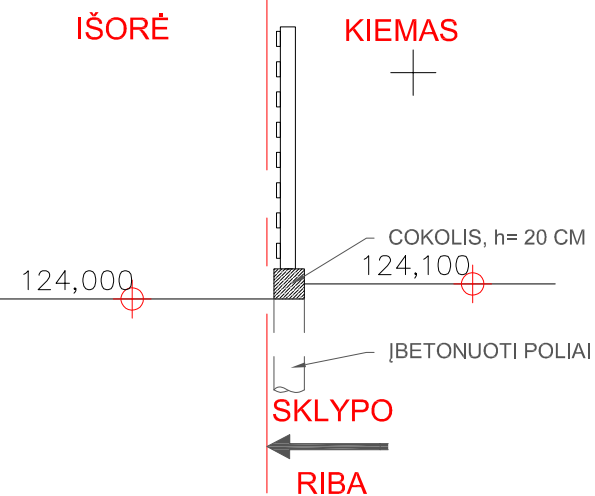
TVOROS SPRENDINIAI PJŪVIS A-A M 1:50
