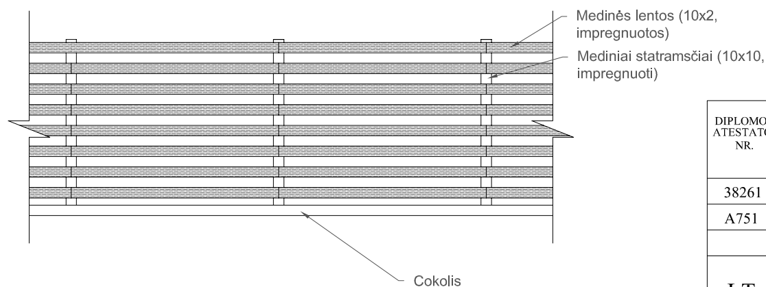
TVOROS SPRENDINIAI TVOROS VAIZDAS IŠ PRIEKIO M 1:50
