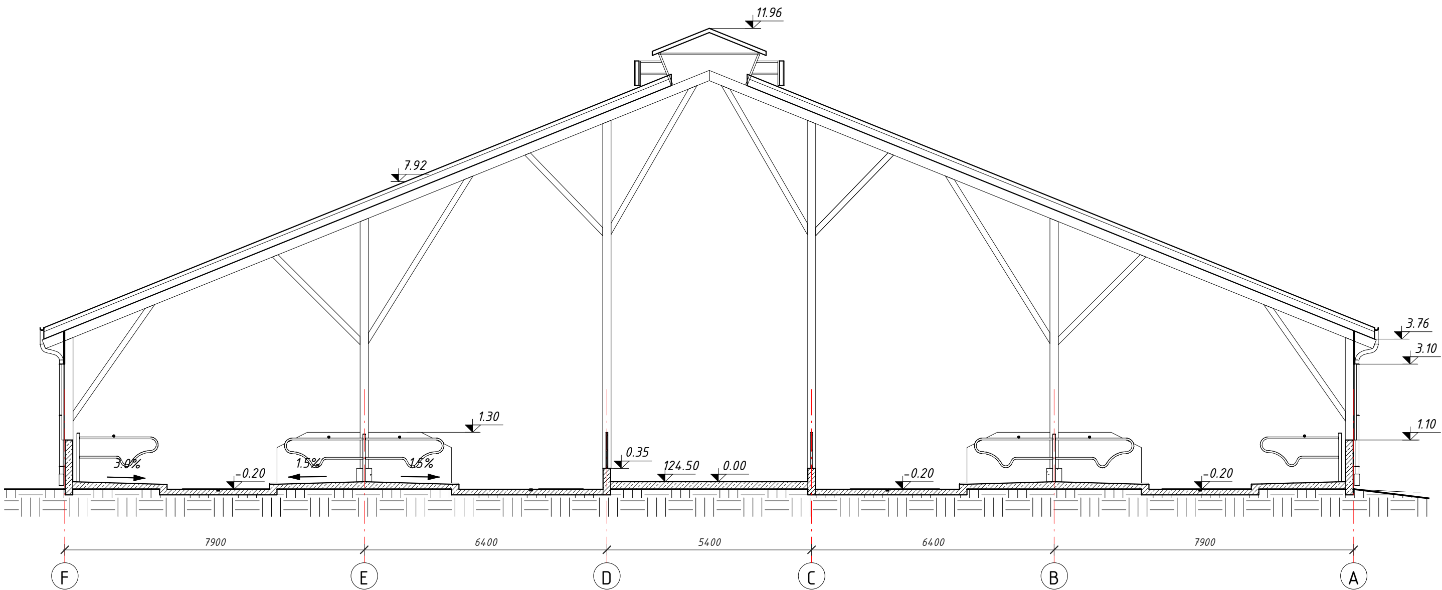
PJŪVIS "1-1", M 1 : 100
