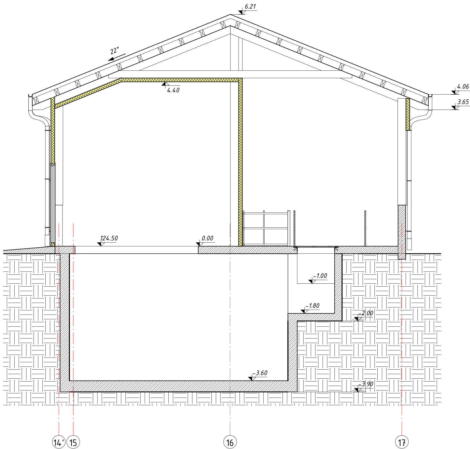
PJŪVIS "4-4", M 1 : 50
