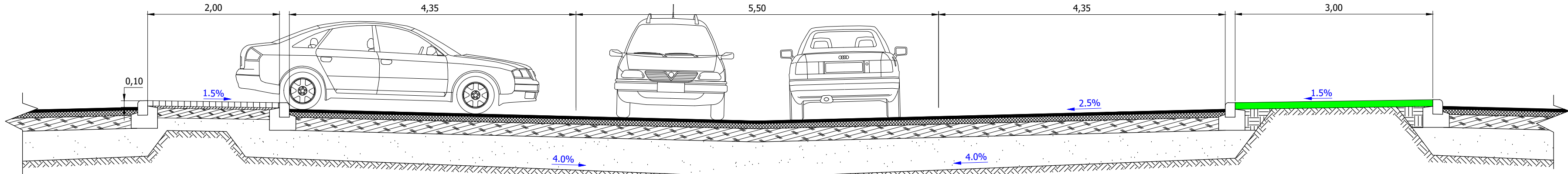
Stovėjimo aikštelės skersinis profilis
