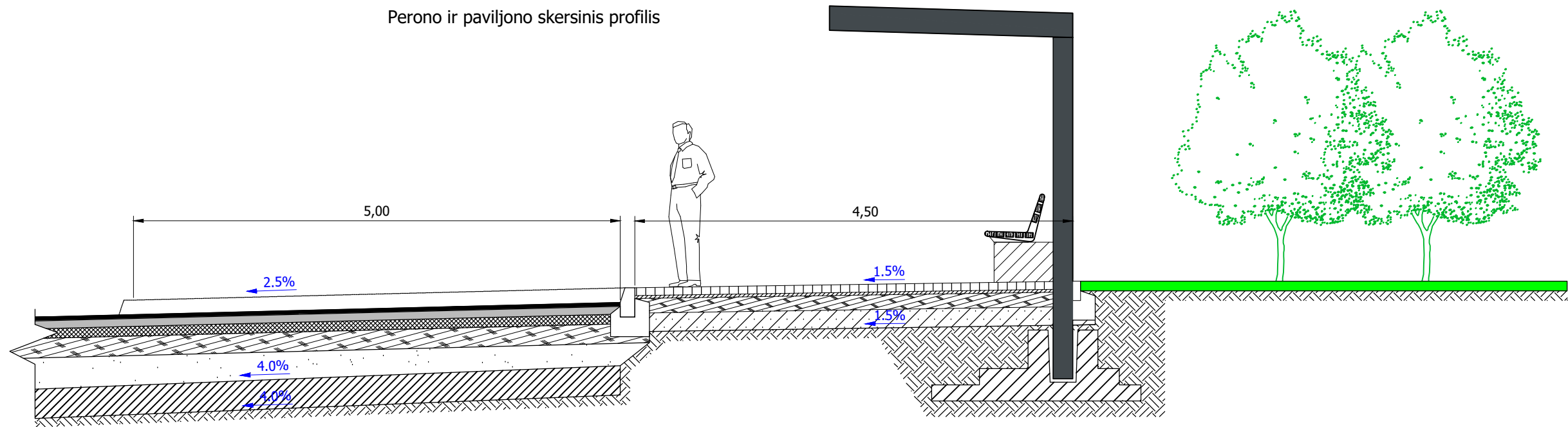
Perono ir paviljono skersinis profilis
