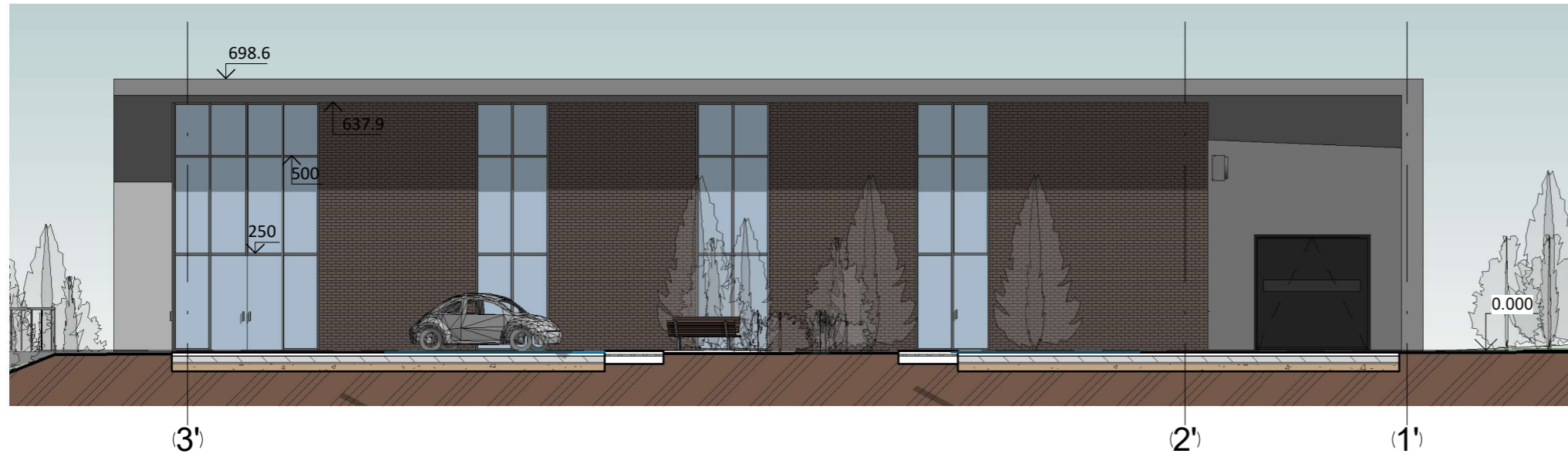
① FASADAS 3'-1' 1 : 150
