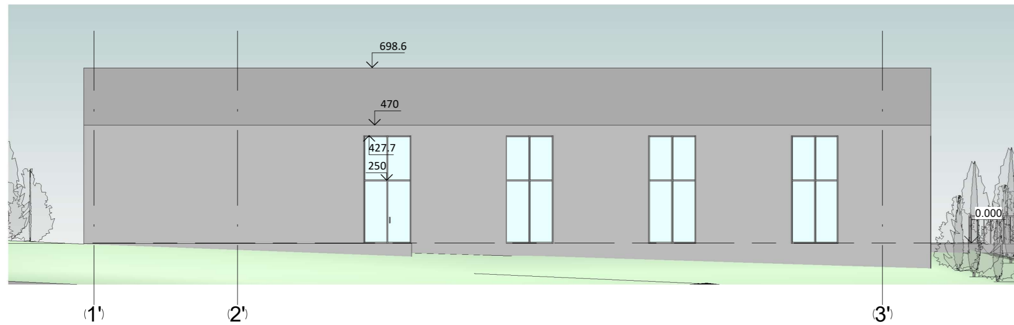
② FASADAS 1'-3' 1 : 150
