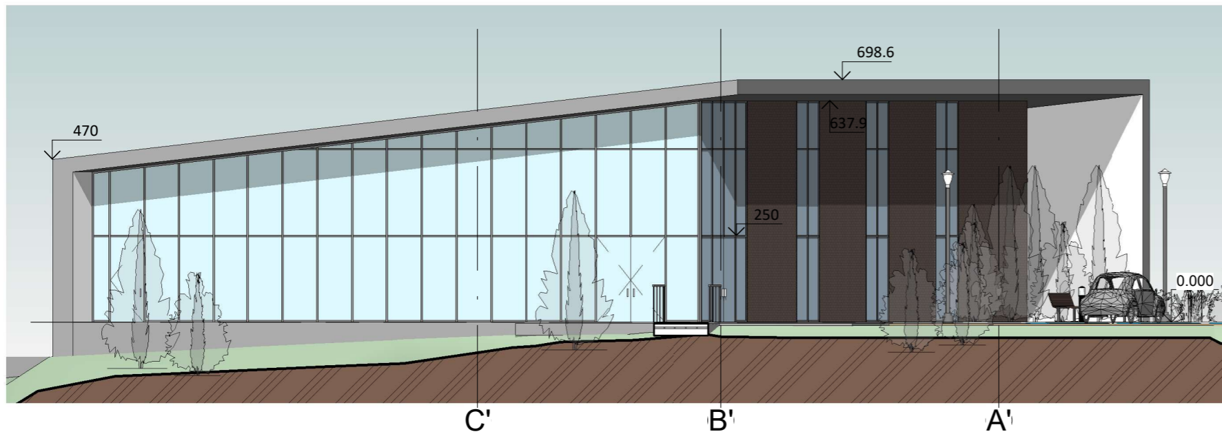
1 FASADAS C'-A' 1 : 150
