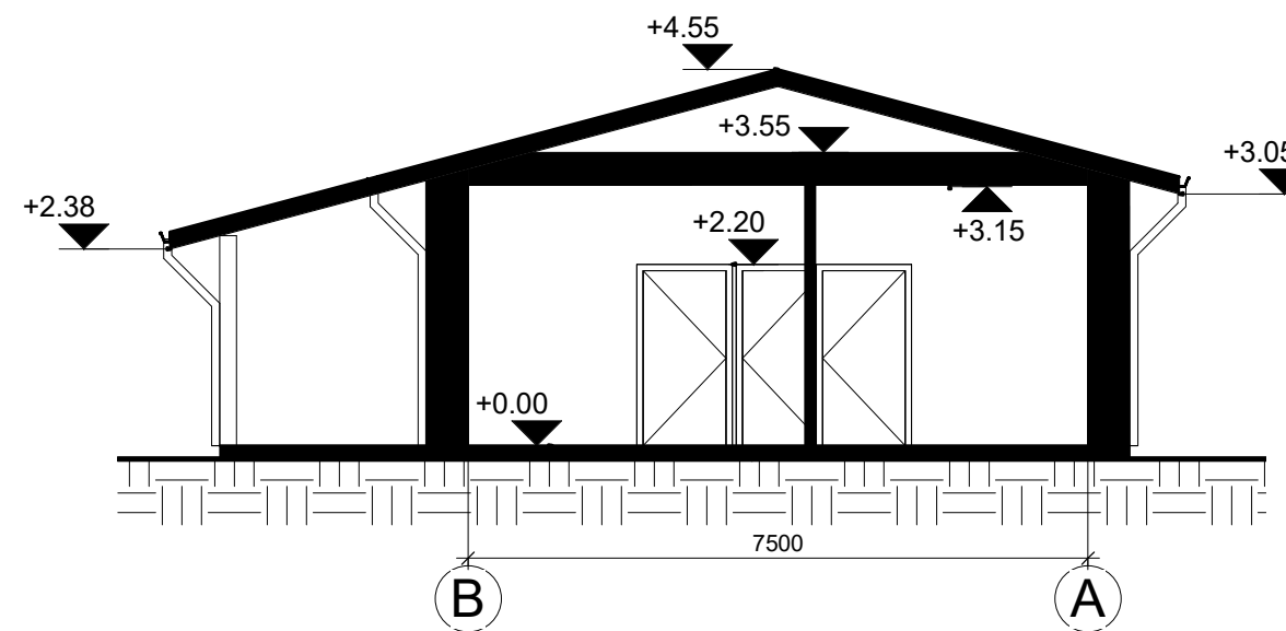
PJŪVIS B - B M 1:100
