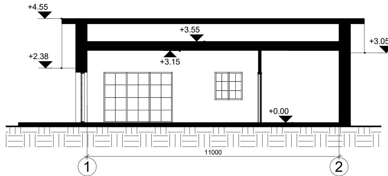
PJŪVIS A - A M 1:100
