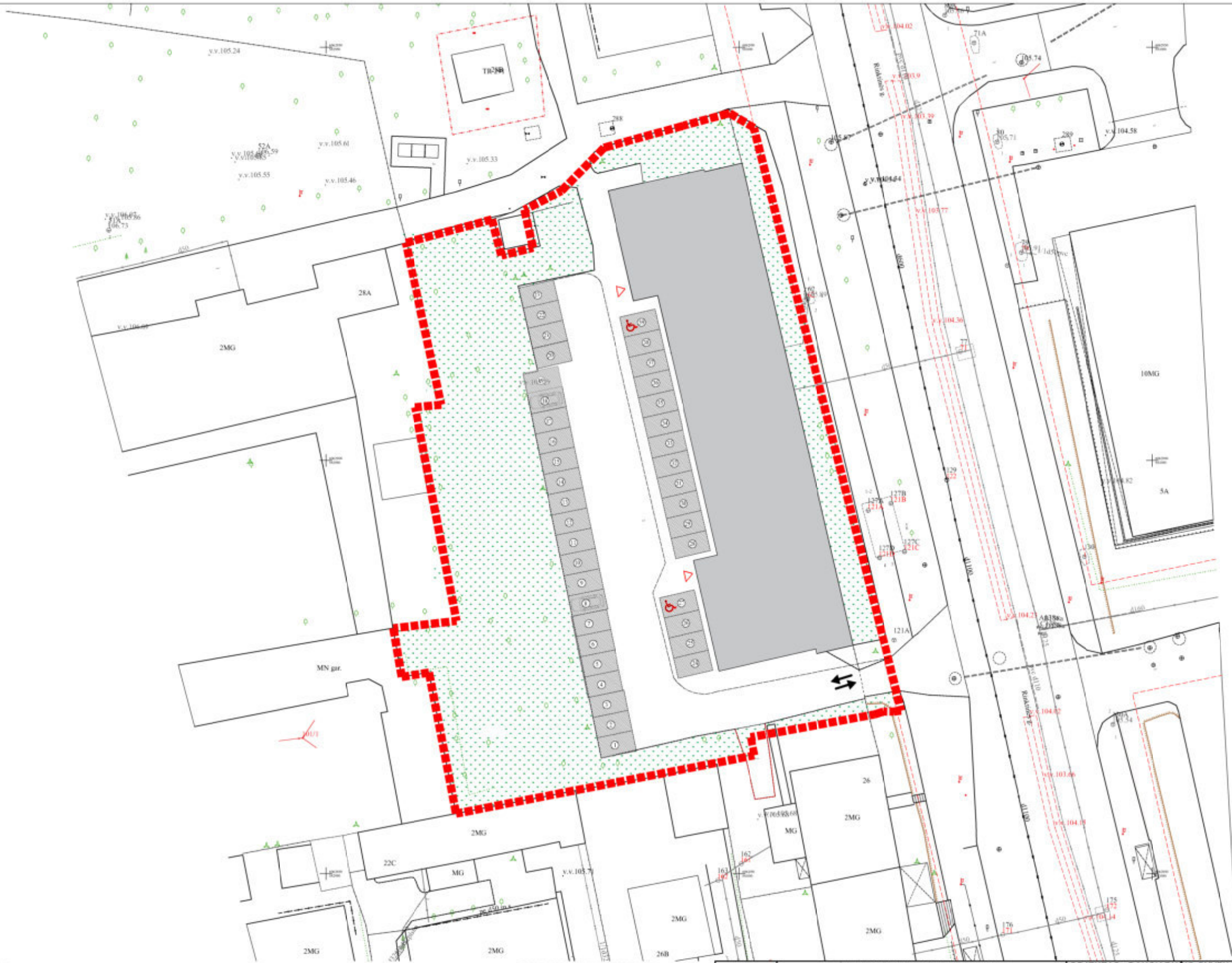
SKLYPO PLANAS M1:500
