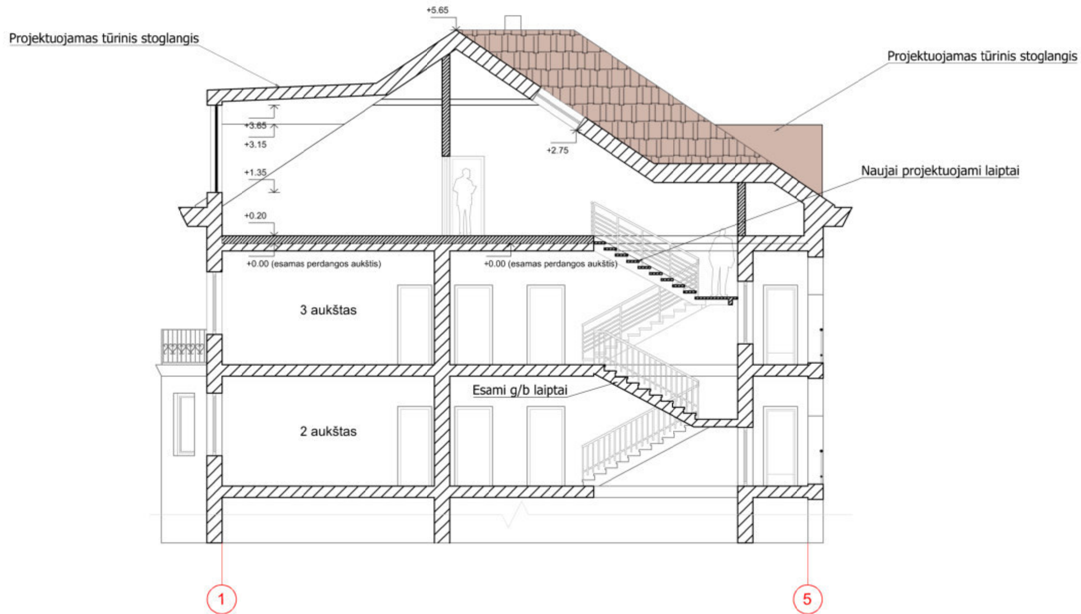
PJŪVIS 1-1 M1:100
