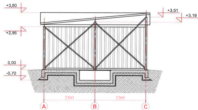
PJŪVIS 1-1 M 1:100
