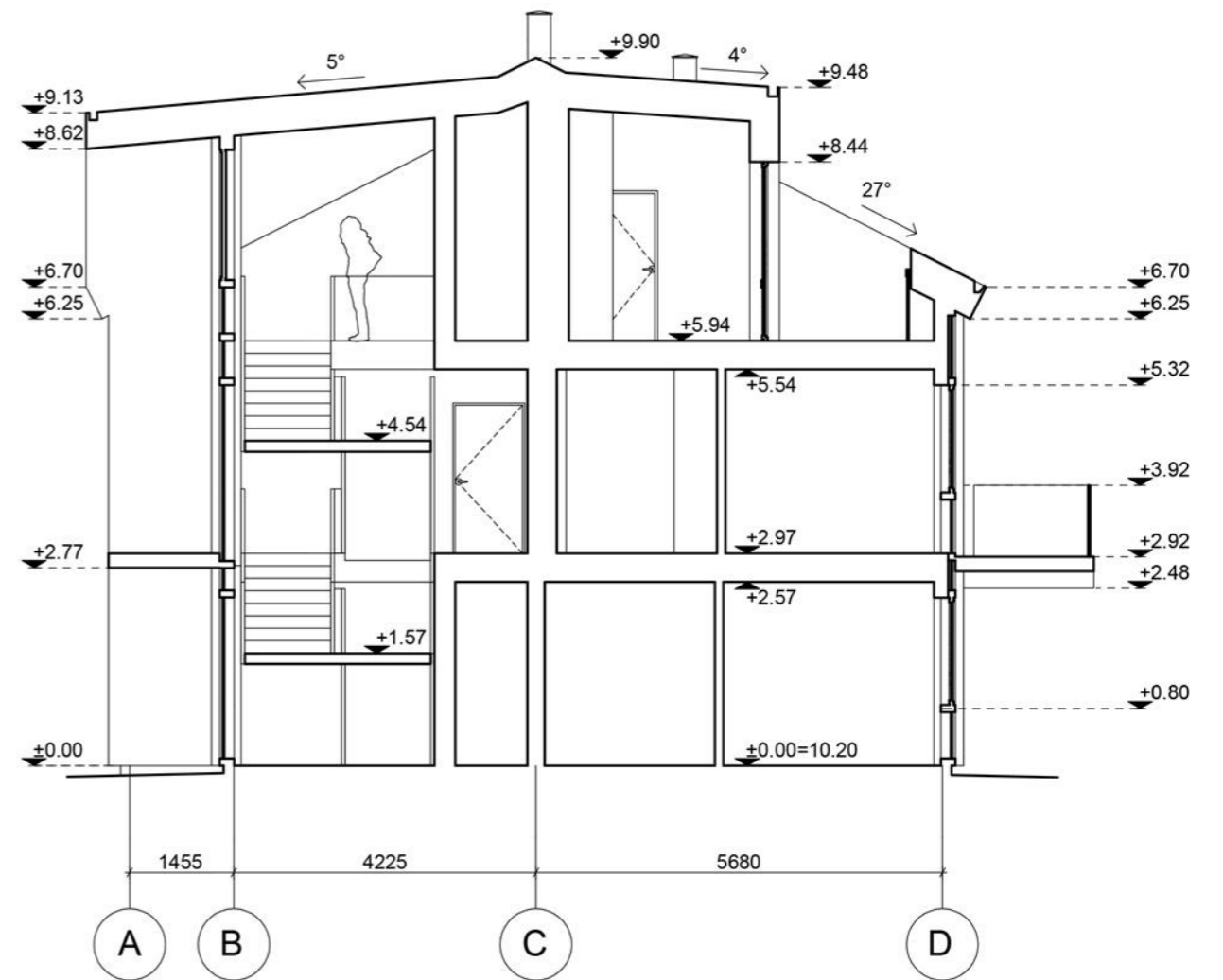
PJŪVIS 2-2 M1:100
