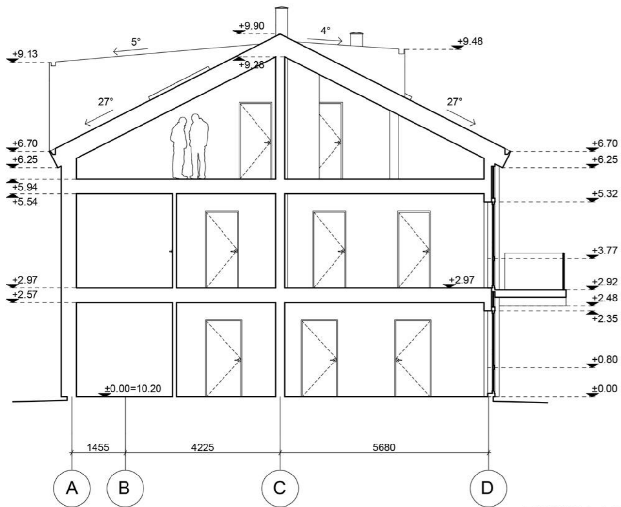
PJŪVIS 1-1 M1:100
