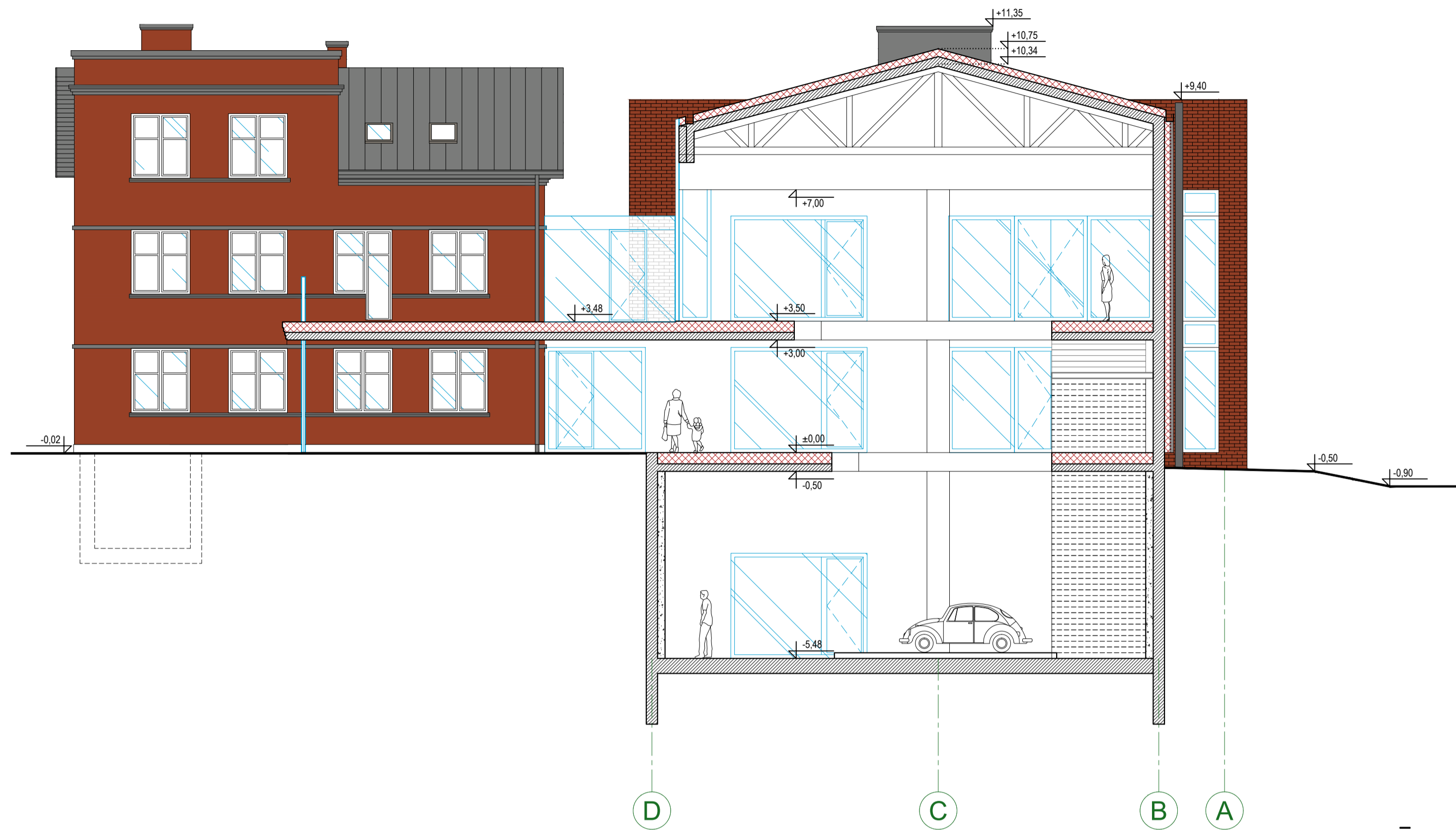
PJŪVIS I-I
