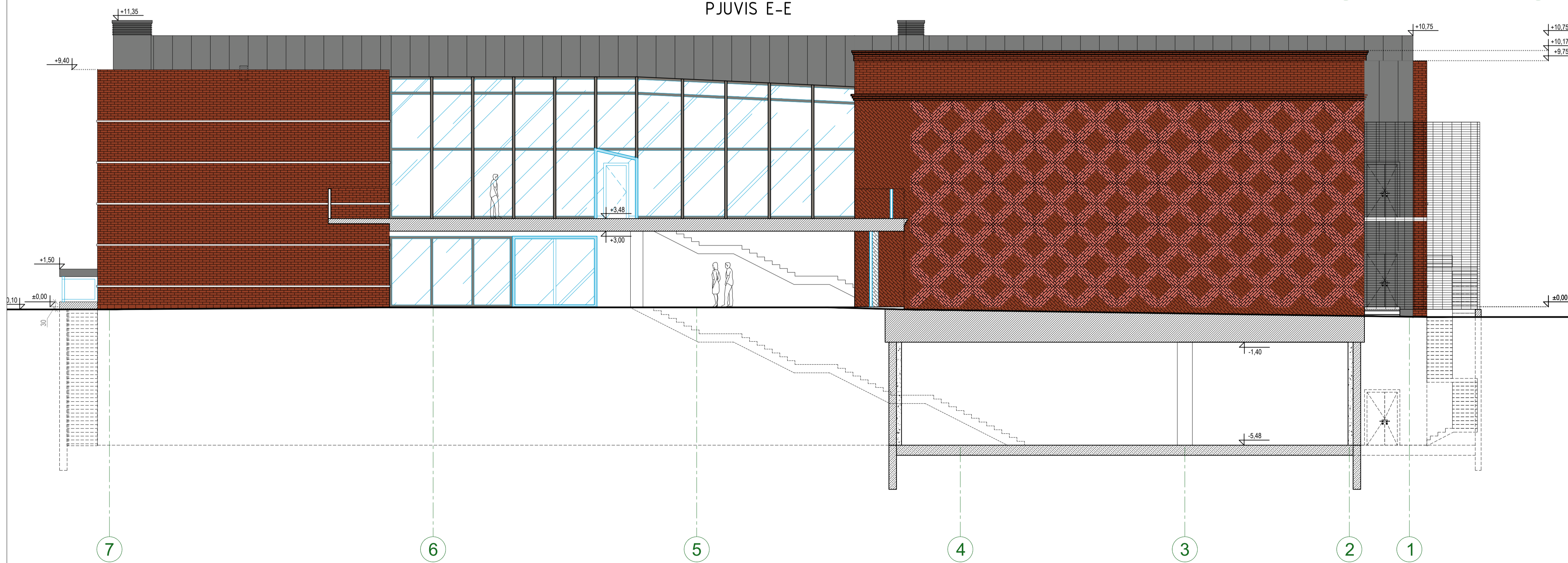
PJŪVIS E-E
