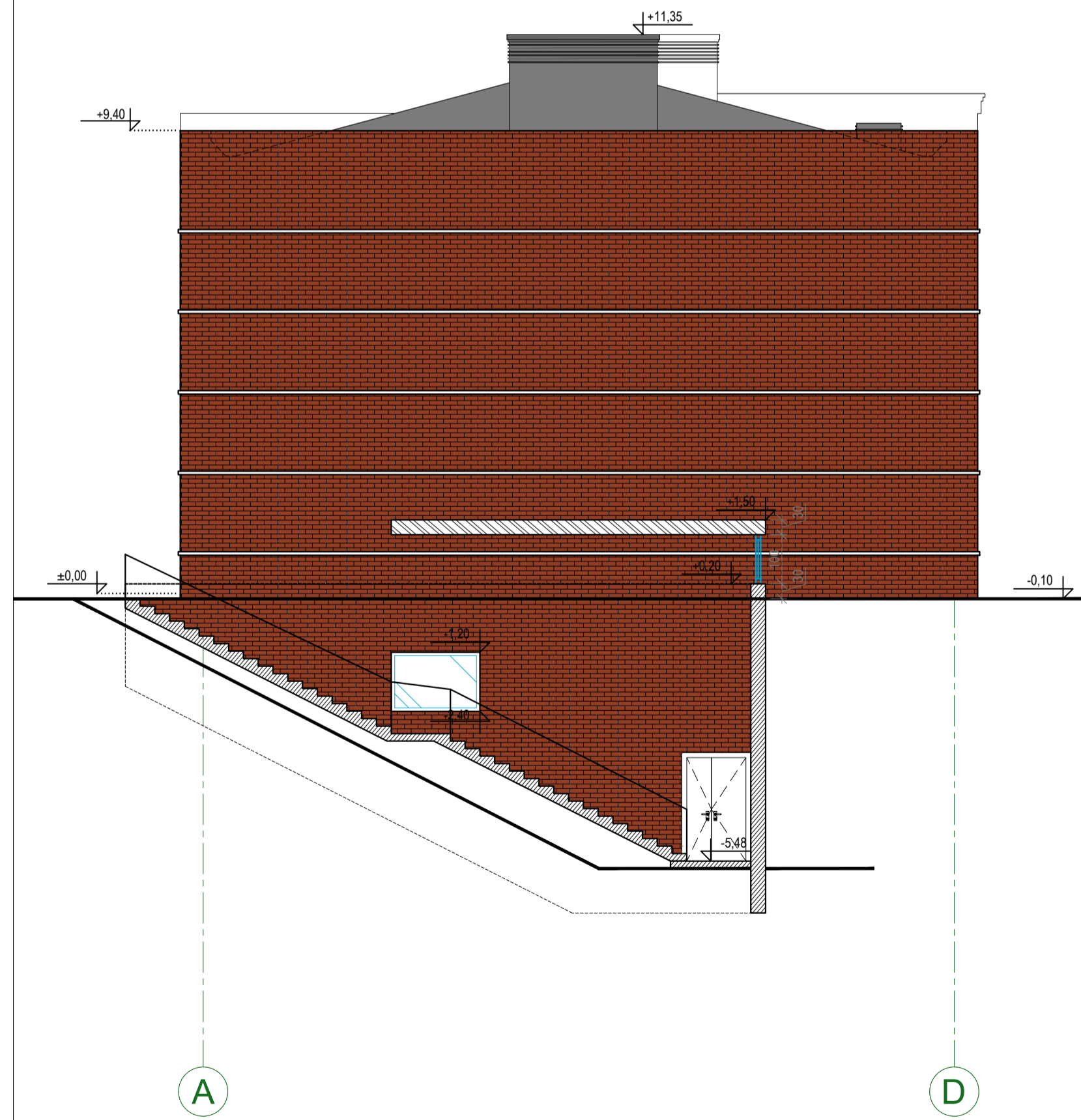
PJŪVIS G-G
