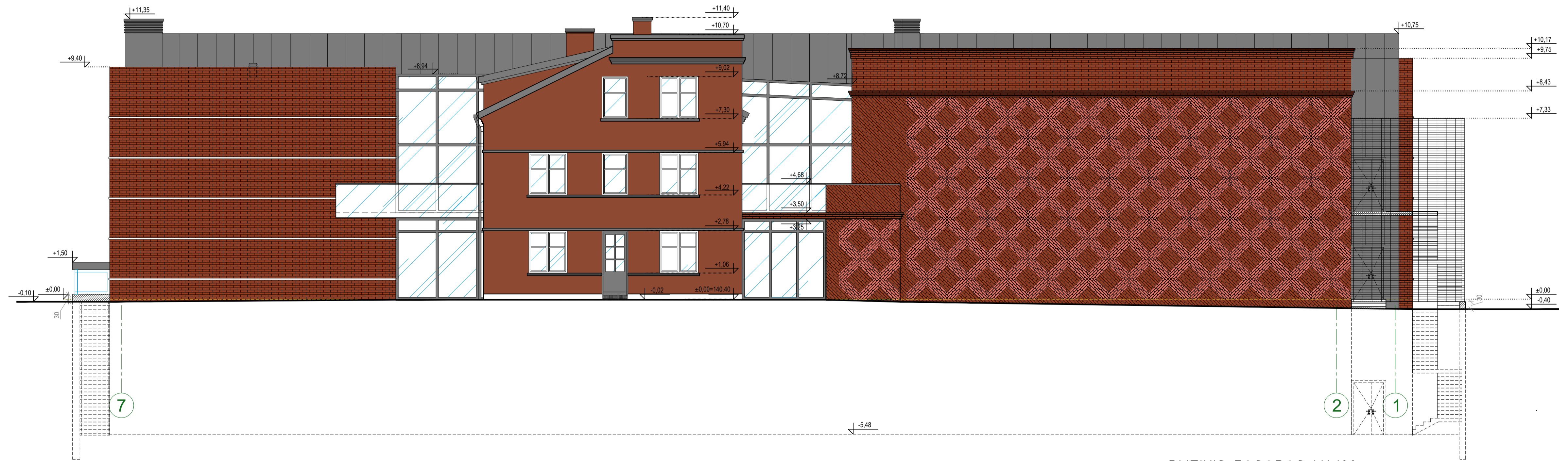
ŠIAURINIS FASADAS M1:100
