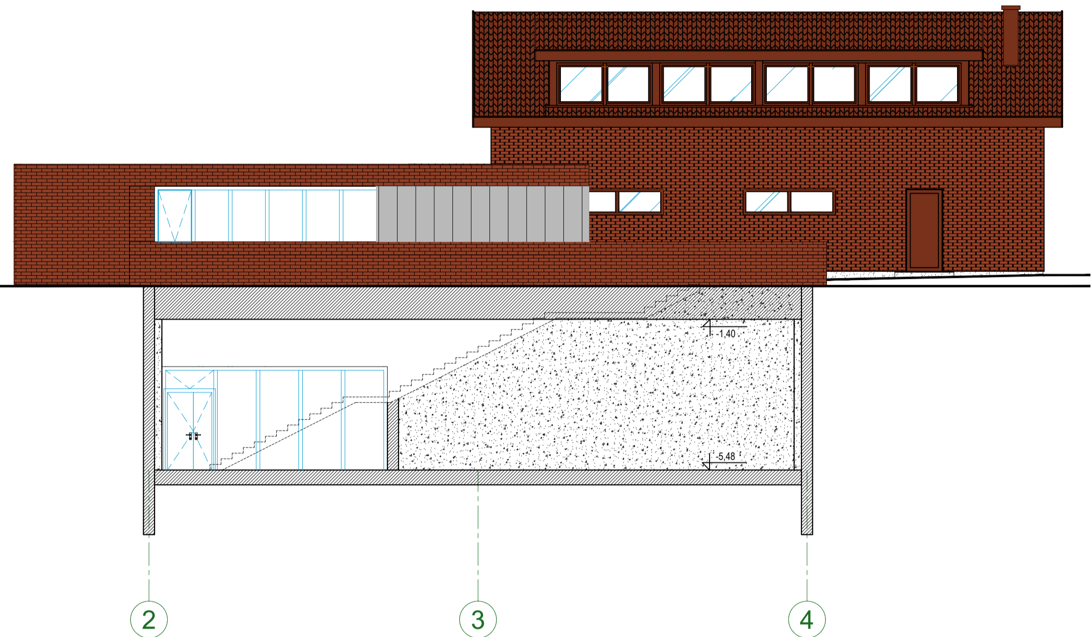
PJŪVIS E-E
