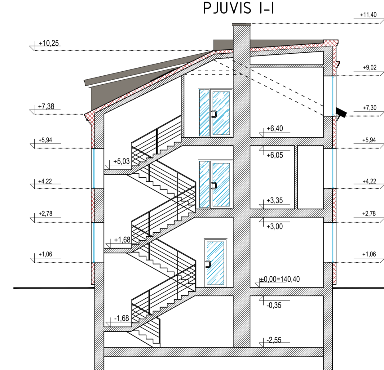
PJŪVIS I-I
