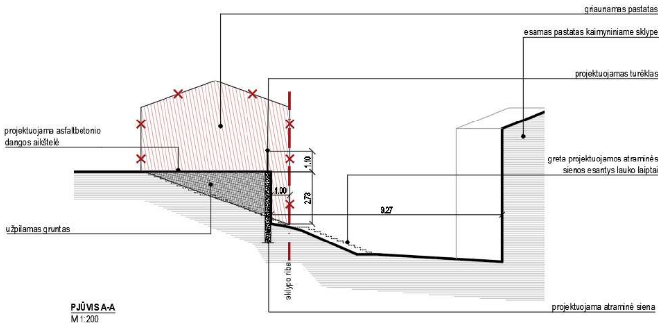
Pjūvis per projektuojamą atraminę sienutę schema
