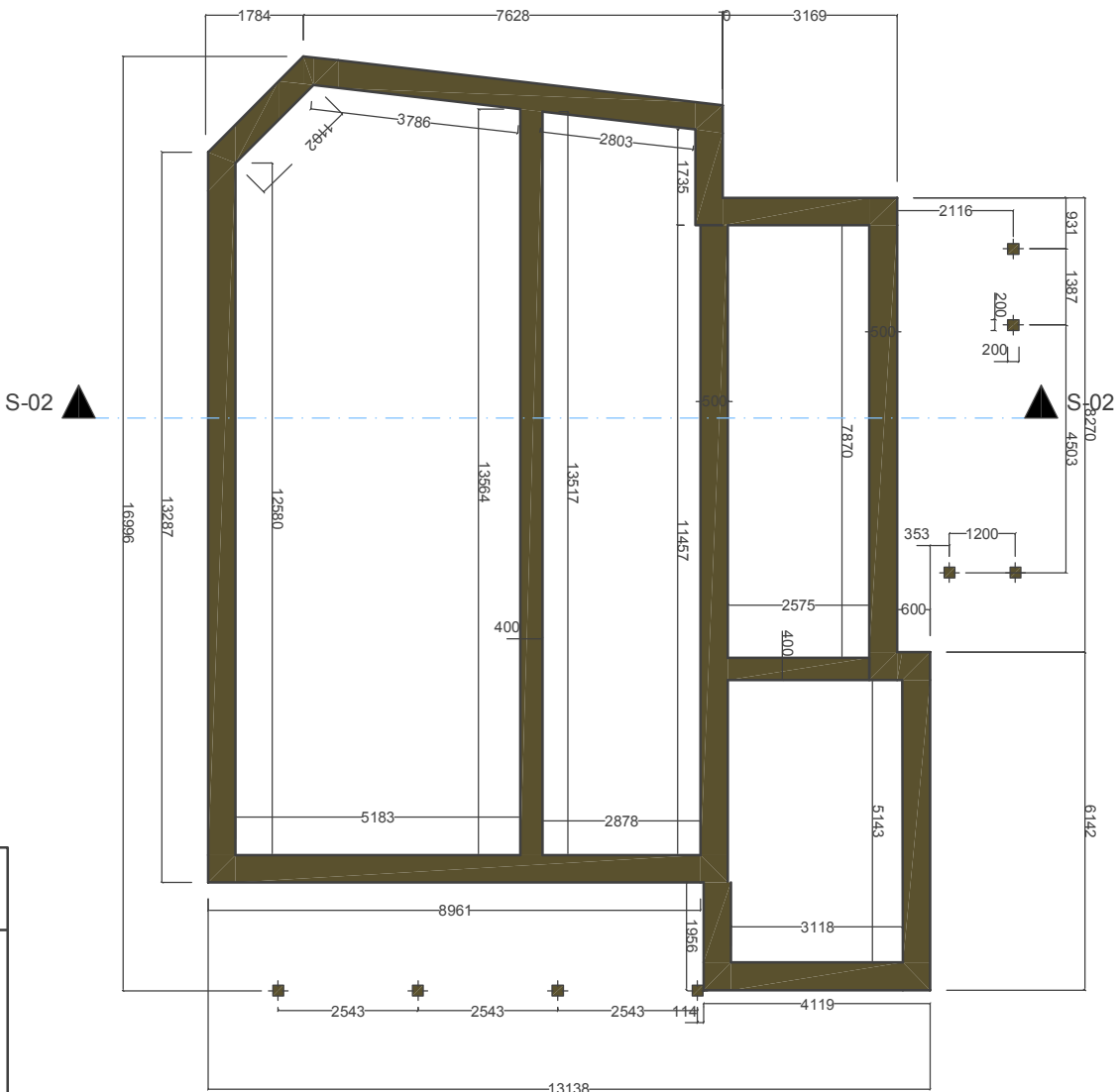
PAMATŲ PLANAS M 1 : 100
