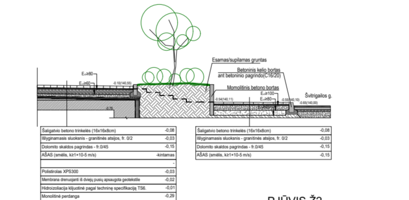
PJŪVIS Ž2
