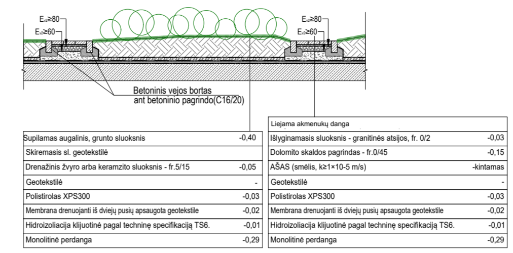
Pjūvis 2-2
