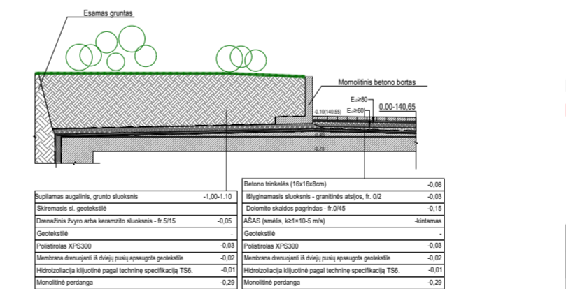
PJŪVIS Ž4
