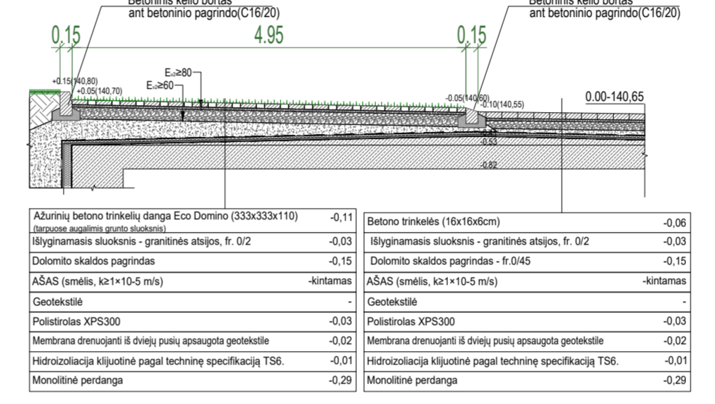
Pjūvis 2-2
