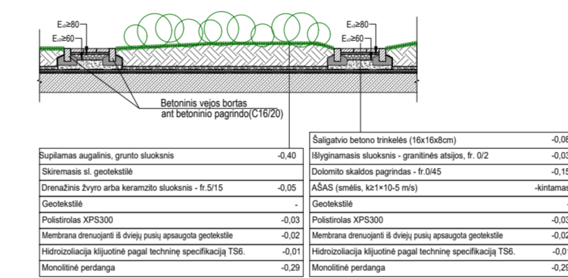
PJŪVIS Ž1
