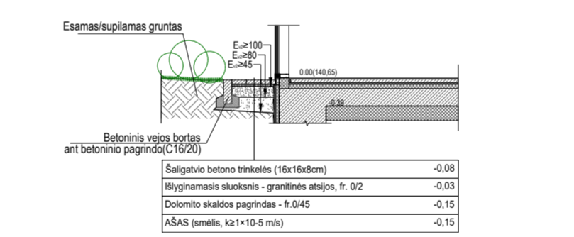
PJŪVIS Ž3
