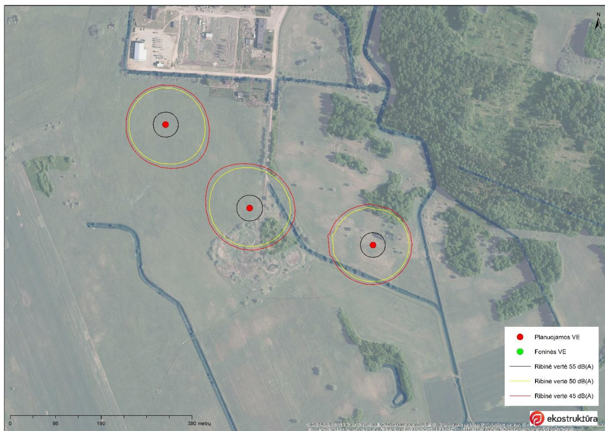
5 pav. Skirtingų paros periodų triukšmo izolinijos
