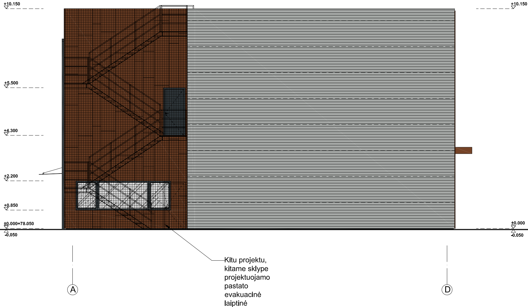
PIETRYČIŲ FASADAS A-D M 1:100
