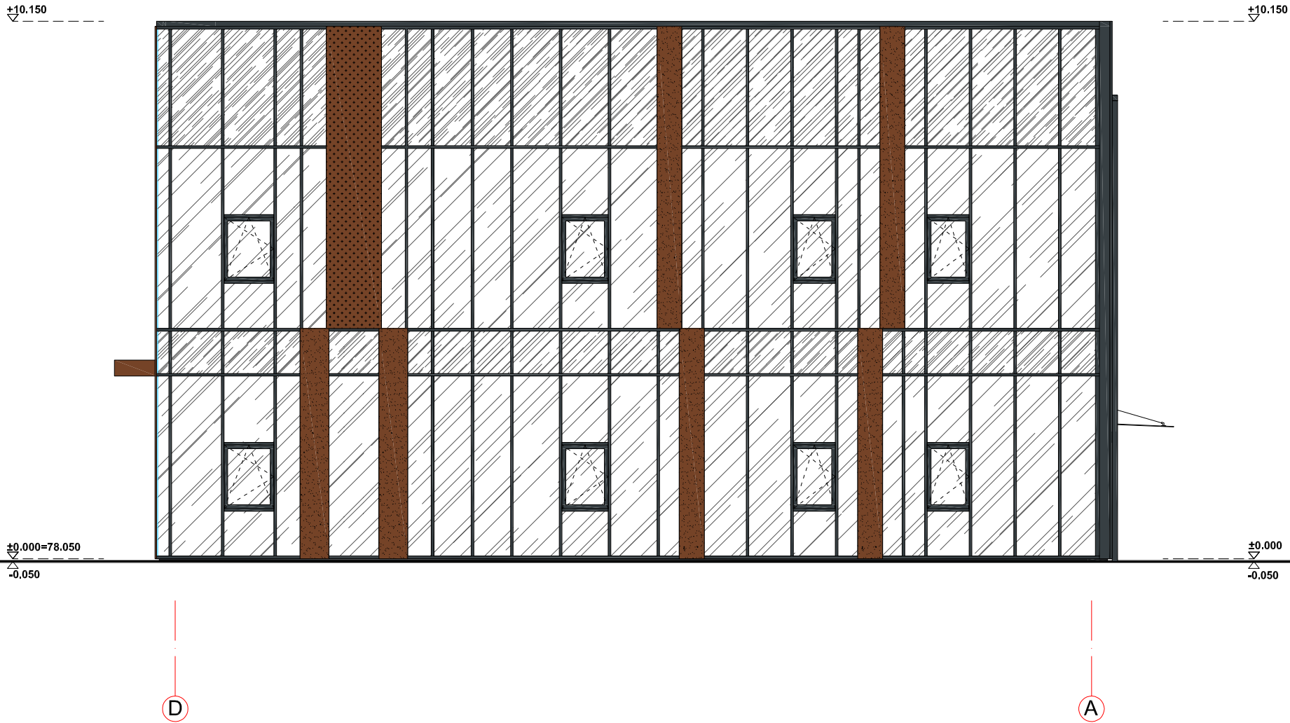
ŠIAURĖS VAKARŲ FASADAS D-A M 1:100
